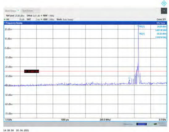
Band41-5MHz-QPSK-41215-1RB#0- Range2:1000~3000MHz
