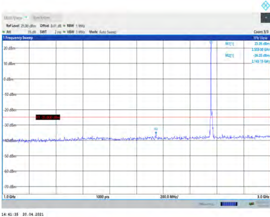
Band41-10MHz-16QAM-40290-1RB#0- Range2:1000~3000MHz
