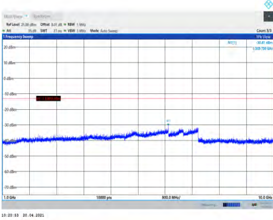
Band26-5MHz-QPSK-26715-1RB#0- Range2:1000~10000MHz
