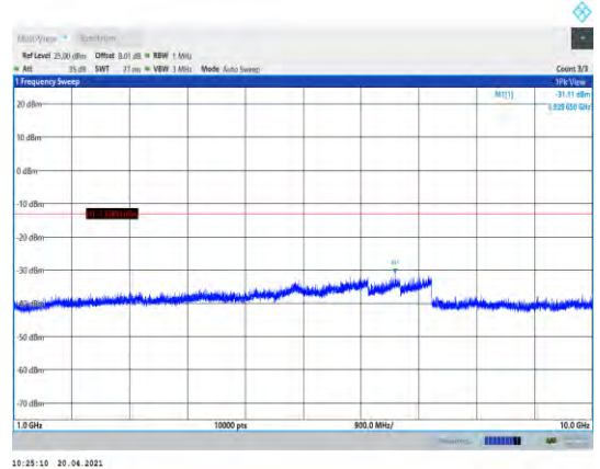
Band26-3MHz-QPSK-26775-1RB#0- Range2:1000~10000MHz
