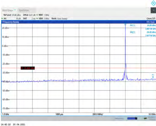
Band41-10MHz-QPSK-40740-1RB#0- Range2:1000~3000MHz
