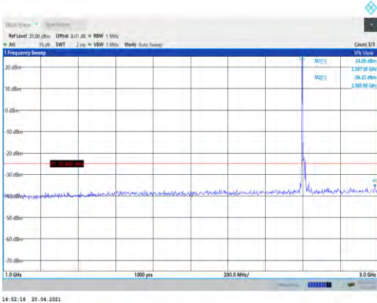
Band41-20MHz-QPSK-40740-1RB#0- Range2:1000~3000MHz
