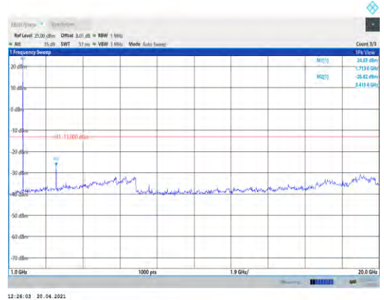
Band66-3MHz-QPSK-131987-1RB#0- Range2:1000~20000MHz
