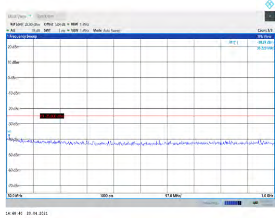
Band41-10MHz-QPSK-40290-1RB#0- Range1:30~1000MHz
