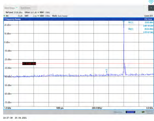
Band38-20MHz-QPSK-38150-1RB#0- Range2:1000~3000MHz
