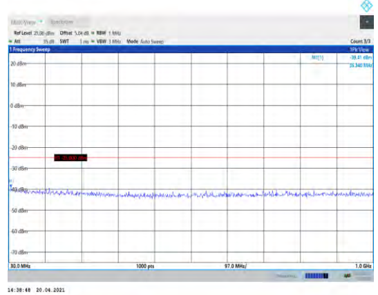
Band41-5MHz-QPSK-41215-1RB#0- Range1:30~1000MHz
