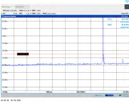
Band38-20MHz-QPSK-38000-1RB#0- Range2:1000~3000MHz
