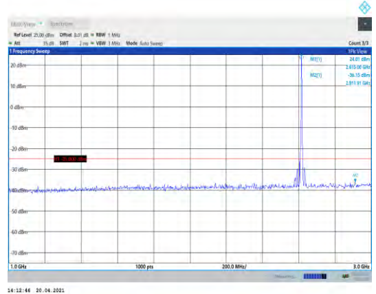
Band38-5MHz-QPSK-38225-1RB#0- Range2:1000~3000MHz
