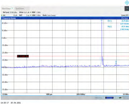
Band38-20MHz-16QAM-37850-1RB#0- Range2:1000~3000MHz
