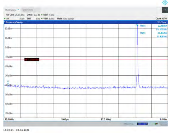
Band26-5MHz-QPSK-26765-1RB#0- Range1:30~1000MHz
