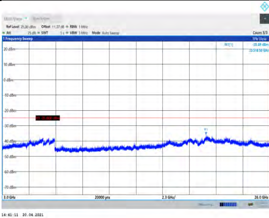
Band41-10MHz-QPSK-40290-1RB#0- Range3:3000~26000MHz
