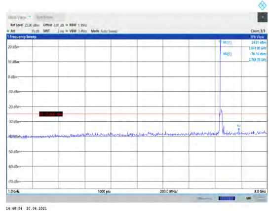
Band41-15MHz-QPSK-41165-1RB#0- Range2:1000~3000MHz
