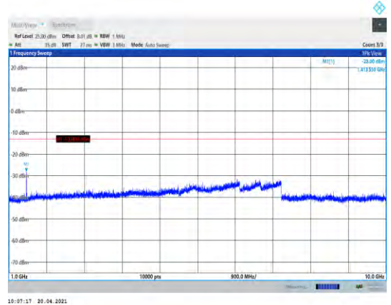
Band12-10MHz-QPSK-23130-1RB#0- Range2:1000~10000MHz
