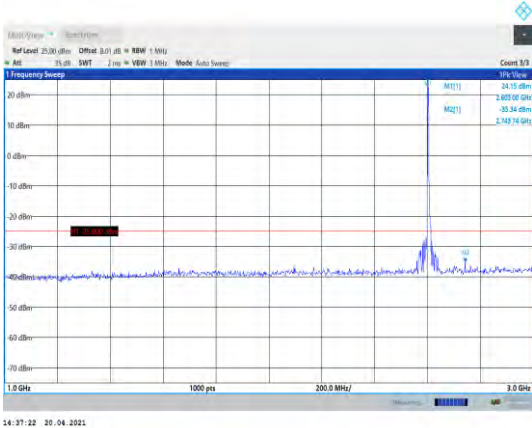
Band41-5MHz-QPSK-40740-1RB#0- Range2:1000~3000MHz
