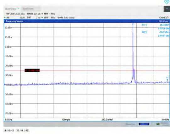
Band41-20MHz-QPSK-40340-1RB#0- Range2:1000~3000MHz
