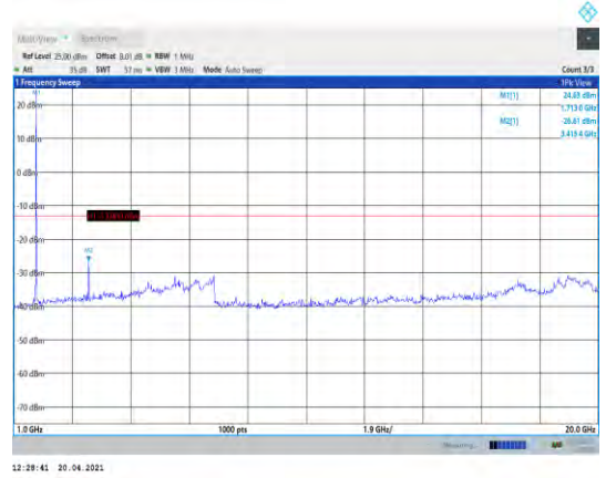
Band66-5MHz-QPSK-131997-1RB#0- Range2:1000~20000MHz
