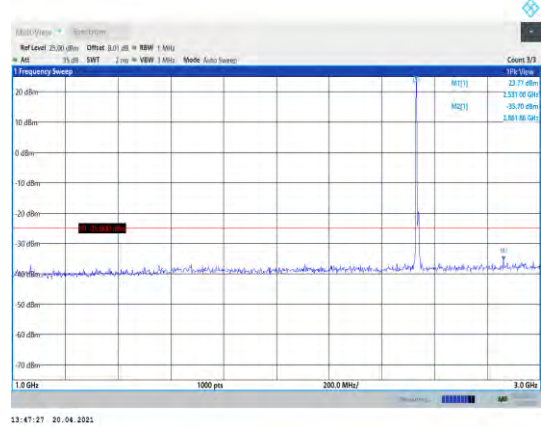
Band7-10MHz-QPSK-21100-1RB#0-Range2:1000~3000MHz
