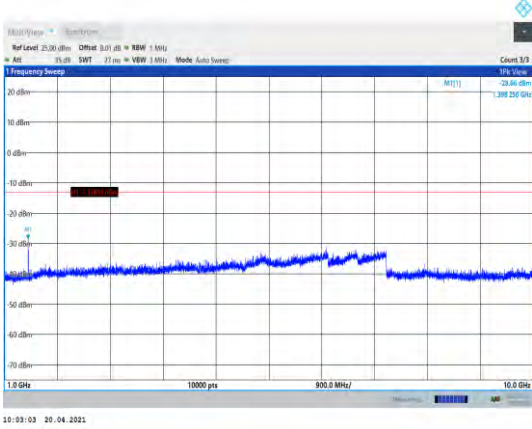
Band12-1.4MHz-QPSK-23017-1RB#0- Range2:1000~10000MHz
