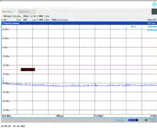
Band7-20MHz-QPSK-21350-1RB#0- Range1:30~1000MHz
