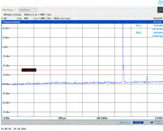
Band7-10MHz-QPSK-20800-1RB#0-Range2:1000~3000MHz
