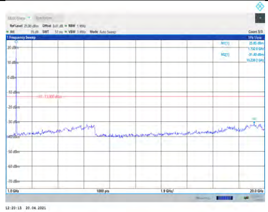
Band4-20MHz-QPSK-20175-1RB#0- Range2:1000~20000MHz
