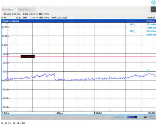
Band4-15MHz-QPSK-20025-1RB#0- Range2:1000~20000MHz
