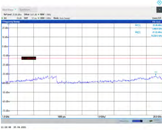
Band2-20MHz-16QAM-18700-1RB#0- Range2:1000~20000MHz
