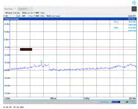
Band2-10MHz-QPSK-19150-1RB#0- Range2:1000~20000MHz
