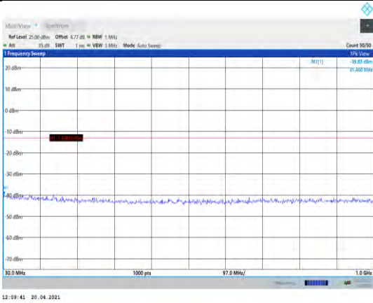
Band4-3MHz-QPSK-19965-1RB#0- Range1:30~1000MHz
