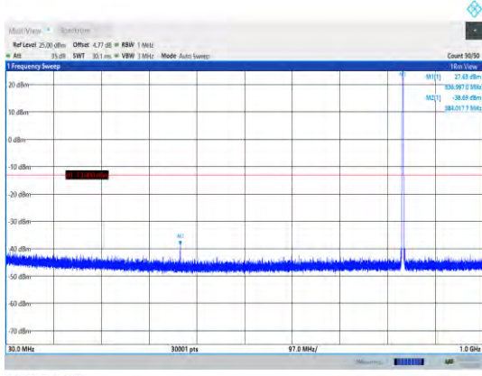
EGPRS850-128-30~1000MHz
