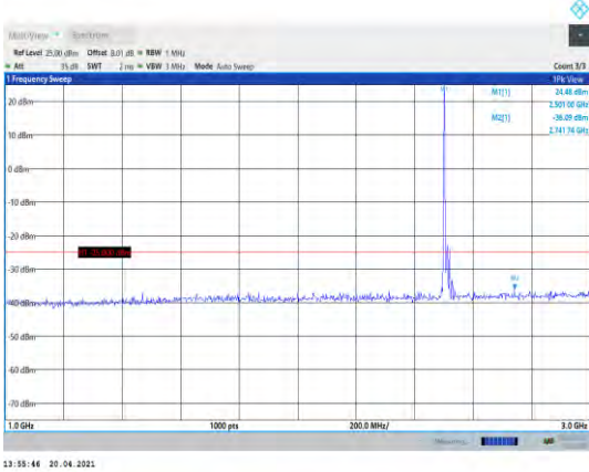
Band7-20MHz-QPSK-20850-1RB#0- Range2:1000~3000MHz
