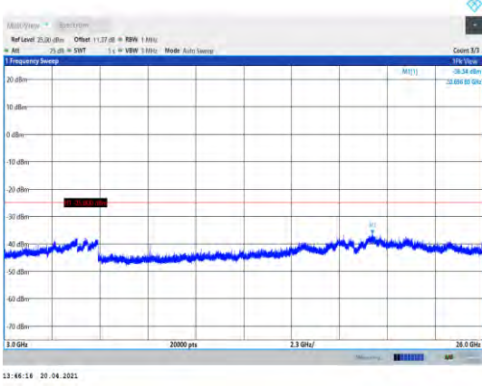
Band7-10MHz-QPSK-20800-1RB#0-Range3:3000~26000MHz
