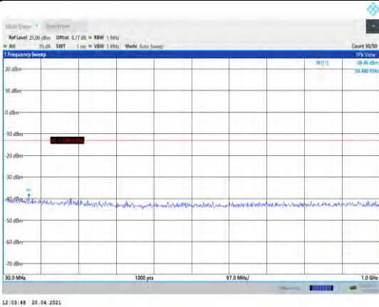
Band4-10MHz-QPSK-20000-1RB#0- Range1:30~1000MHz
