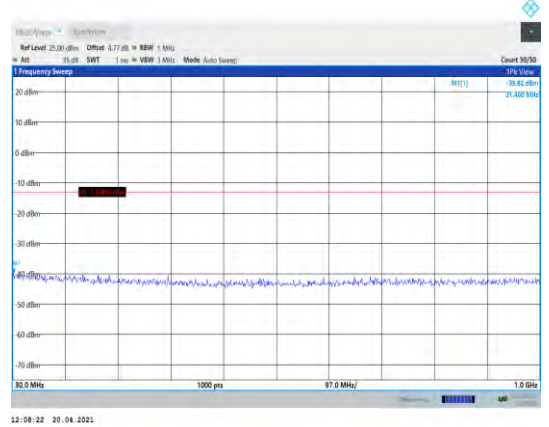
Band4-5MHz-QPSK-20375-1RB#0- Range1:30~1000MHz
