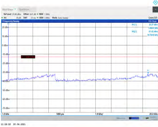
Band2-20MHz-QPSK-18700-1RB#0- Range2:1000~20000MHz
