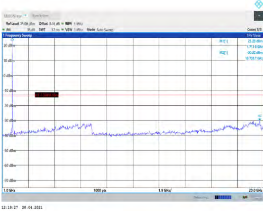
Band4-20MHz-QPSK-20050-1RB#0- Range2:1000~20000MHz
