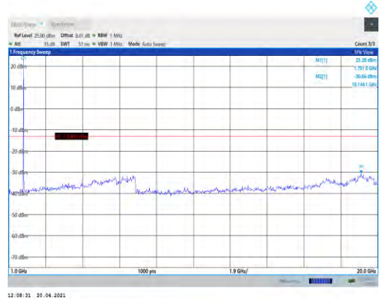
Band4-5MHz-QPSK-20375-1RB#0- Range2:1000~20000MHz
