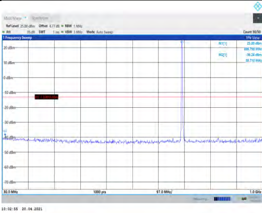
Band12-1.4MHz-QPSK-23017-1RB#0- Range1:30~1000MHz
