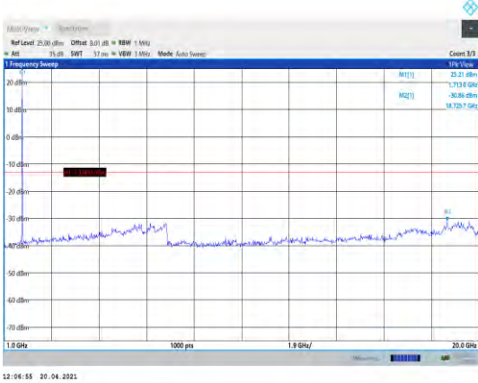
Band4-5MHz-QPSK-19975-1RB#0- Range2:1000~20000MHz
