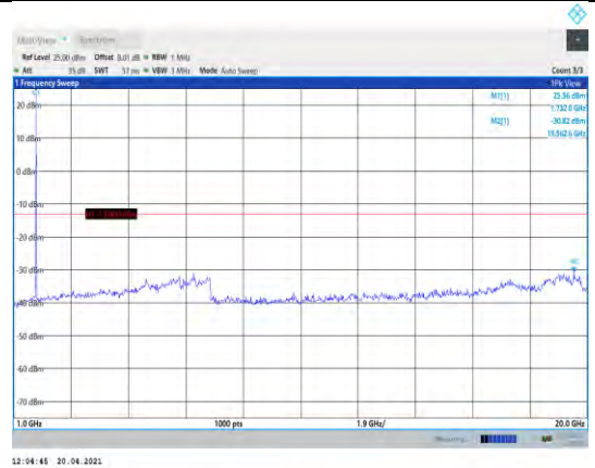
Band4-10MHz-QPSK-20175-1RB#0- Range2:1000~20000MHz
