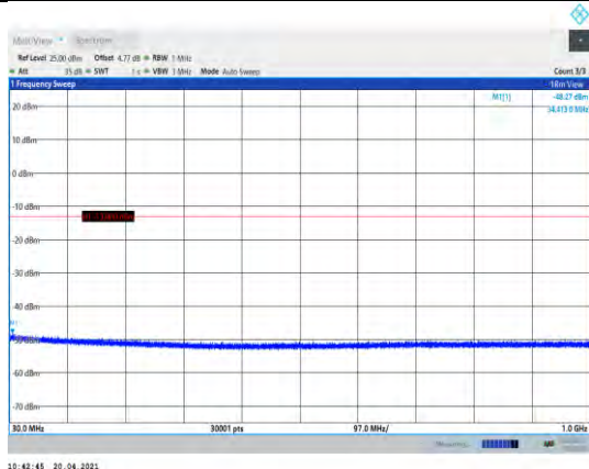
Band4-1413-30~1000MHz
