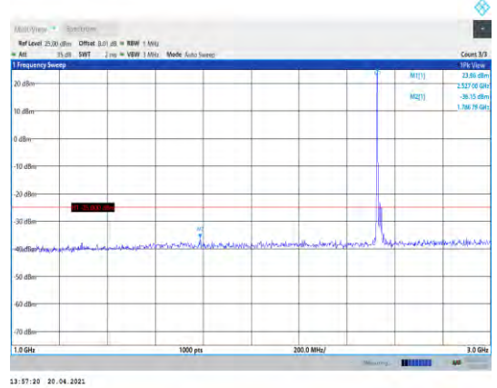
Band7-20MHz-QPSK-21100-1RB#0- Range2:1000~3000MHz
