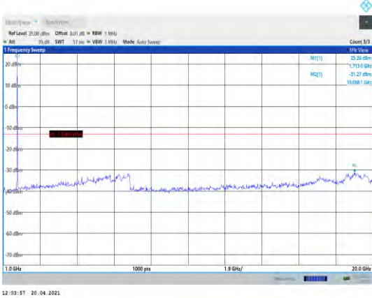
Band4-10MHz-QPSK-20000-1RB#0- Range2:1000~20000MHz
