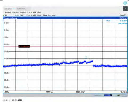
Band5-10MHz-QPSK-20525-1RB#0- Range2:1000~10000MHz
