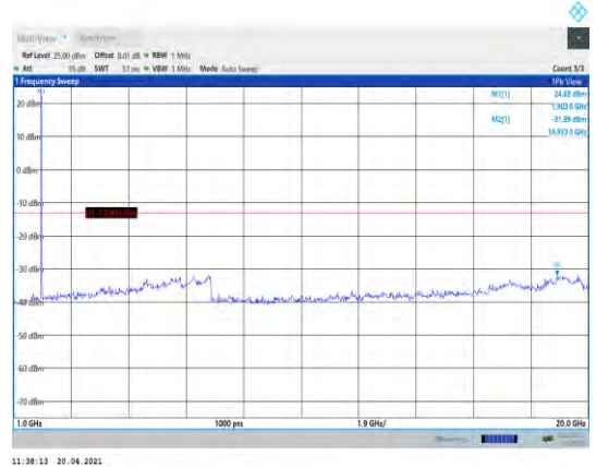
Band2-5MHz-16QAM-19175-1RB#0- Range2:1000~20000MHz
