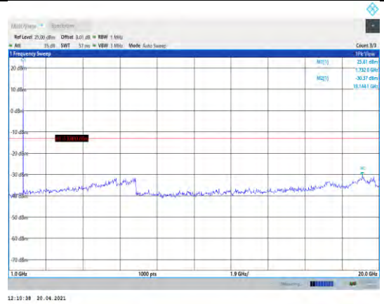
Band4-3MHz-QPSK-20175-1RB#0- Range2:1000~20000MHz
