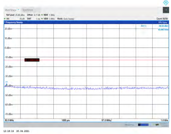
Band4-1.4MHz-QPSK-20393-1RB#0- Range1:30~1000MHz
