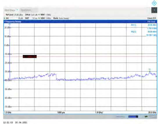
Band4-20MHz-QPSK-20300-1RB#0- Range2:1000~20000MHz
