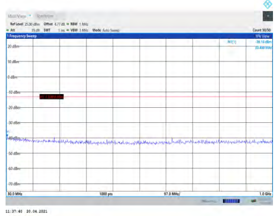
Band2-5MHz-QPSK-19175-1RB#0- Range1:30~1000MHz
