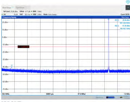
EGPRS850-190-30~1000MHz
