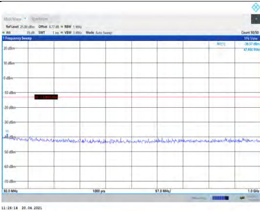
Band2-20MHz-QPSK-18700-1RB#0- Range1:30~1000MHz
