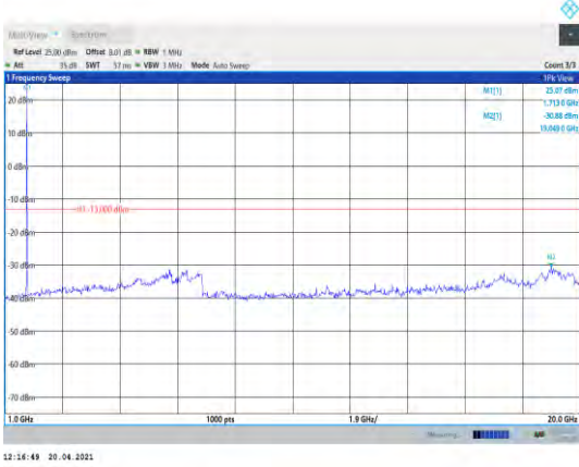
Band4-1.4MHz-QPSK-19957-1RB#0- Range2:1000~20000MHz
