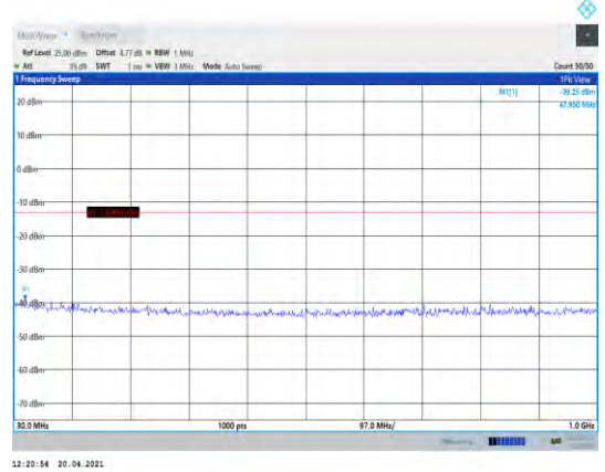
Band4-20MHz-QPSK-20300-1RB#0- Range1:30~1000MHz
