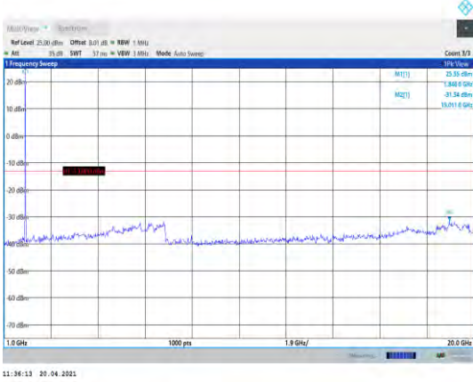
Band2-5MHz-QPSK-18625-1RB#0- Range2:1000~20000MHz
