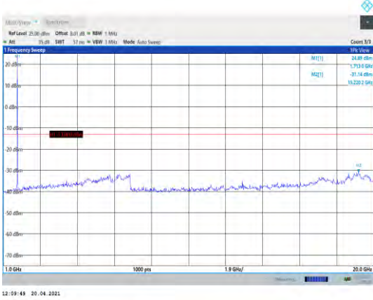
Band4-3MHz-QPSK-19965-1RB#0- Range2:1000~20000MHz
