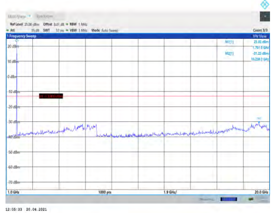
Band4-10MHz-QPSK-20350-1RB#0- Range2:1000~20000MHz
