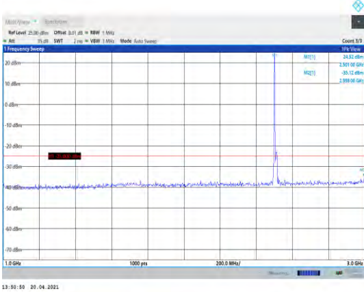
Band7-15MHz-QPSK-20825-1RB#0- Range2:1000~3000MHz
