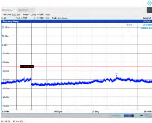
Band7-20MHz-QPSK-20850-1RB#0- Range3:3000~26000MHz
