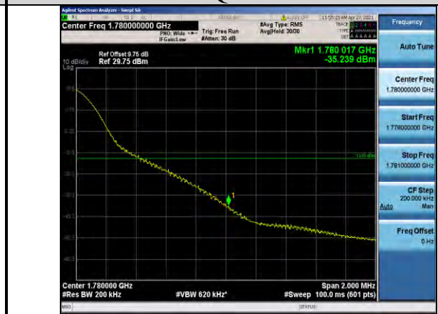
Band66-20MHz-QPSK-132572-1RB#99
