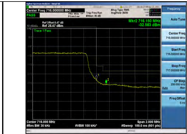
Band12-3MHz-QPSK-23165-15RB#0
