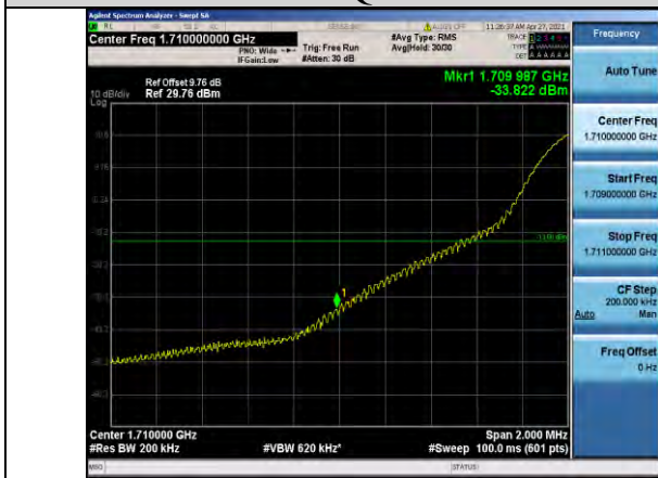
Band66-20MHz-QPSK-132072-1RB#0
