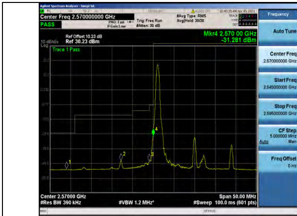
Band38-20MHz-QPSK-37850-1RB#0
