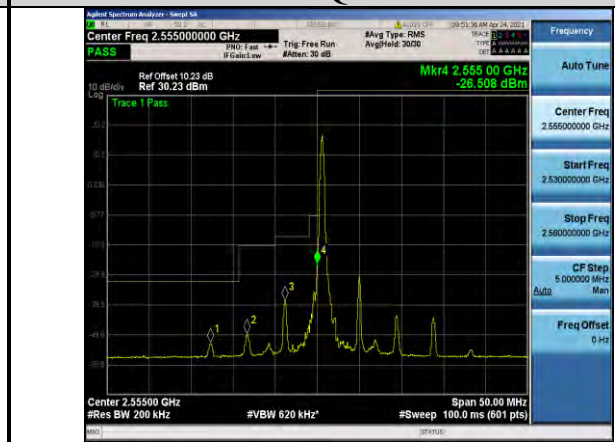
Band41-10MHz-QPSK-40290-1RB#0
