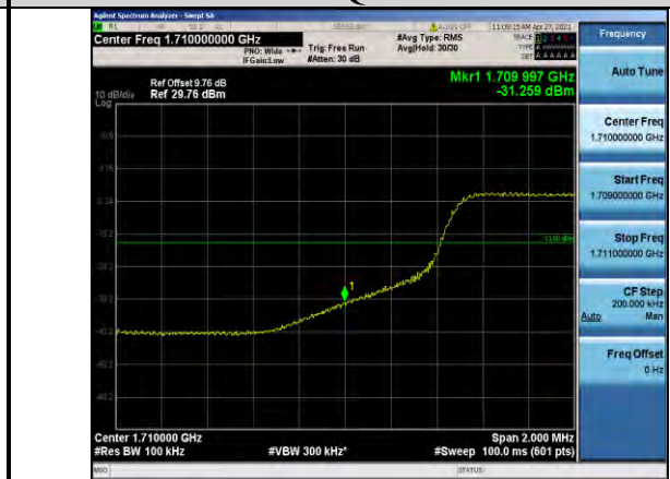
Band66-10MHz-QPSK-132022-50RB#0
