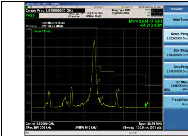
Band38-15MHz-QPSK-38175-1RB#74
