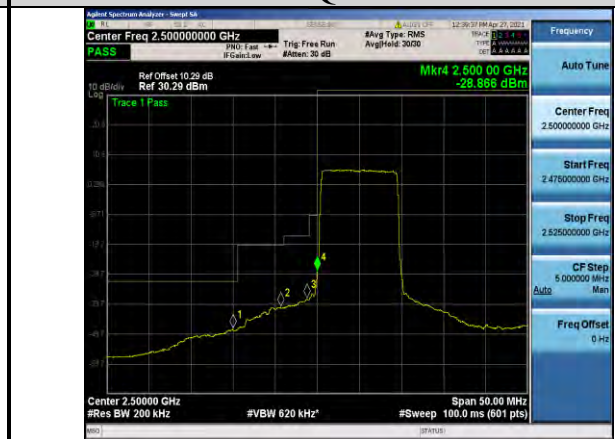
Band7-10MHz-QPSK-20800-50RB#0
