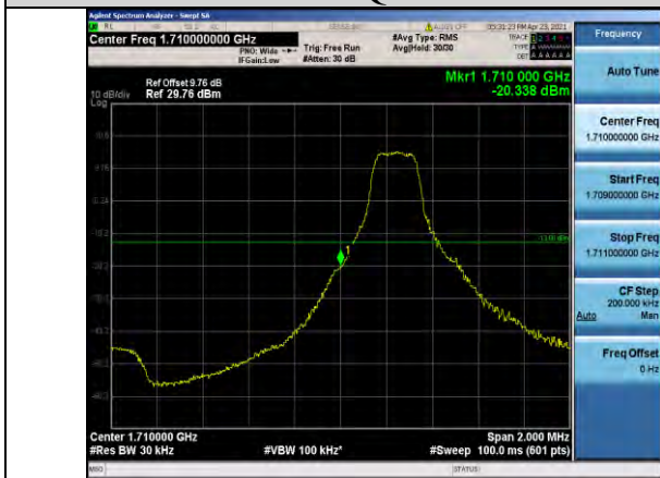
Band4-3MHz-QPSK-19965-1RB#0
