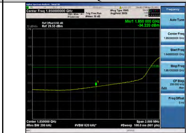
Band2-20MHz-QPSK-18700-100RB#0
