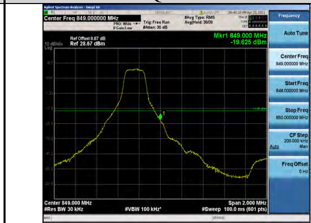
Band5-3MHz-QPSK-20635-1RB#14
