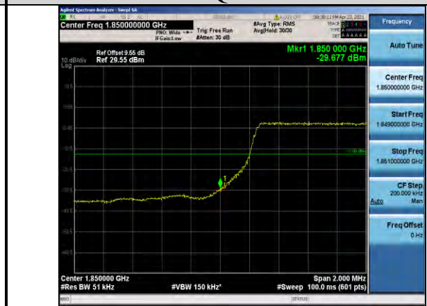
Band2-5MHz-QPSK-18625-25RB#0
