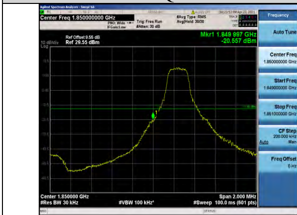
Band2-3MHz-QPSK-18615-1RB#0
