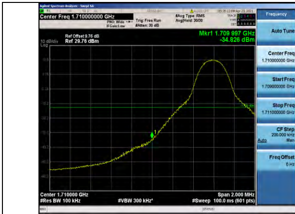
Band4-10MHz-QPSK-20000-1RB#0
