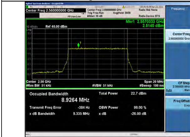
Band41-10MHz-QPSK-40290-50RB#0-8.9264
