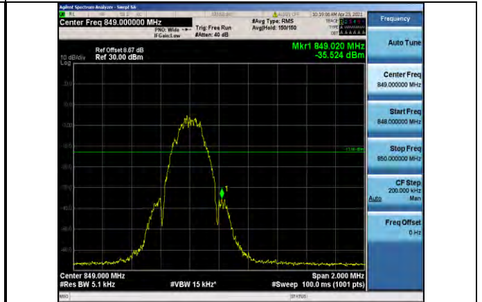
EGPRS850-251
