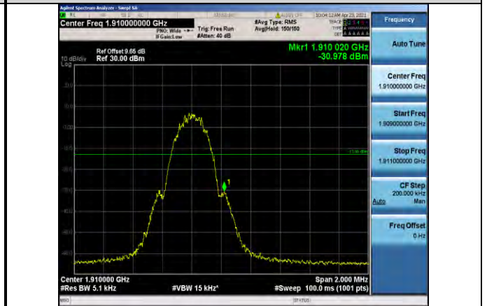
GSM1900-810
