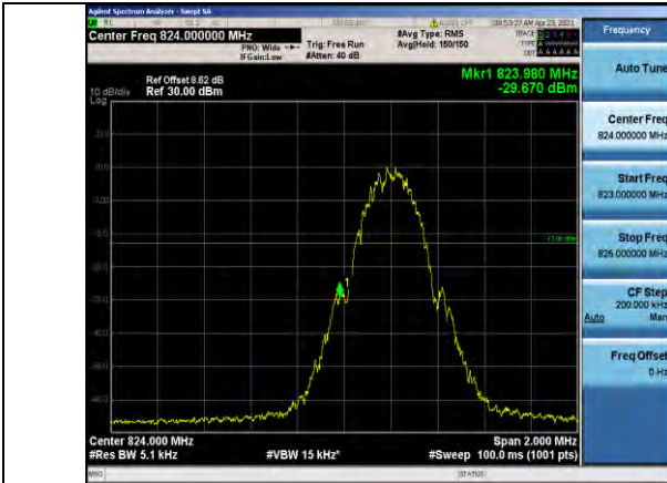
GSM850-128
