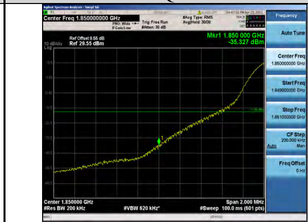
Band2-20MHz-QPSK-18700-1RB#0
