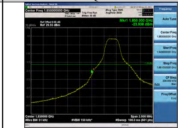
Band2-5MHz-QPSK-18625-1RB#0
