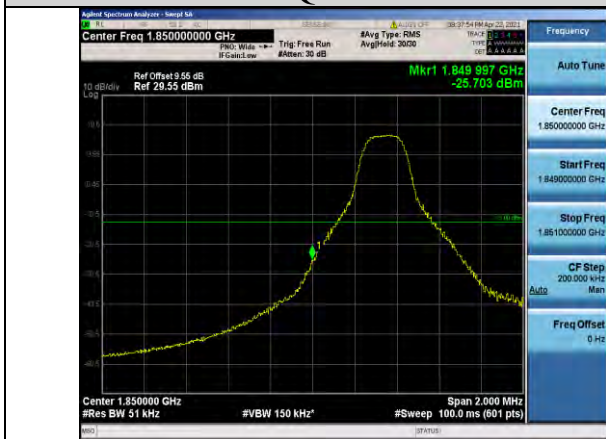
Band2-5MHz-16QAM-18625-1RB#0
