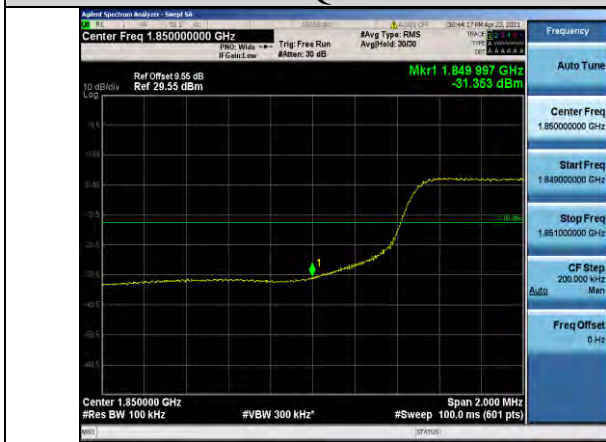
Band2-10MHz-QPSK-18650-50RB#0
