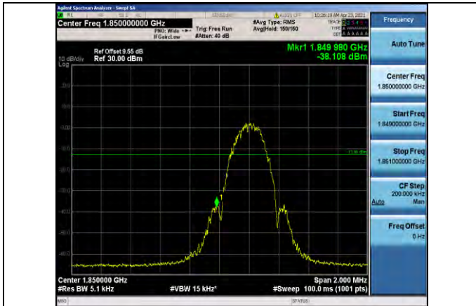
EGPRS1900-512
