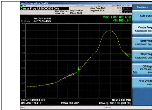
Band2-10MHz-QPSK-18650-1RB#0
