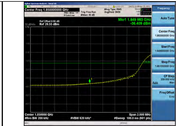
Band2-20MHz-16QAM-18700-100RB#0
