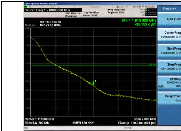
Band2-20MHz-QPSK-19100-1RB#99
