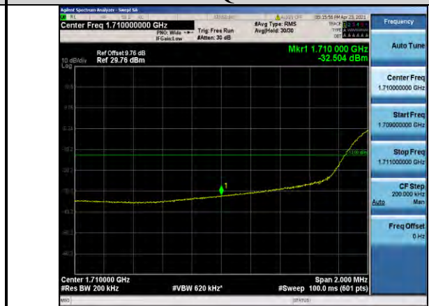
Band4-20MHz-QPSK-20050-100RB#0
