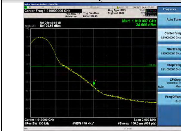
Band2-15MHz-16QAM-19125-1RB#74
