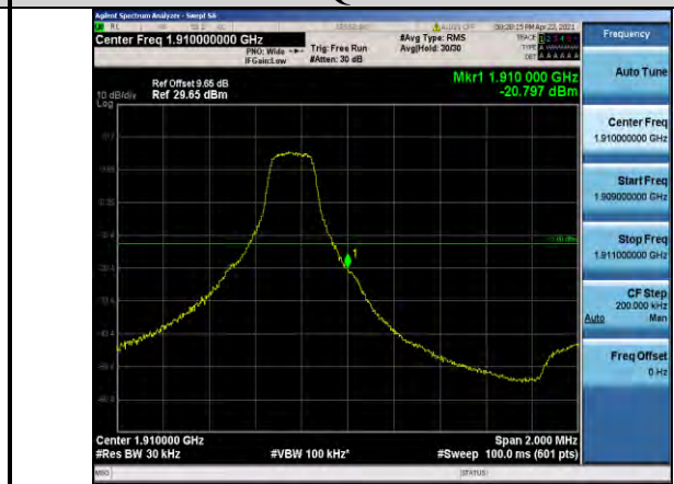
Band2-3MHz-QPSK-19185-1RB#14
