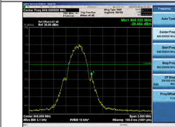
GSM850-251
