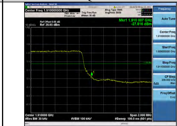
Band2-3MHz-QPSK-19185-15RB#0
