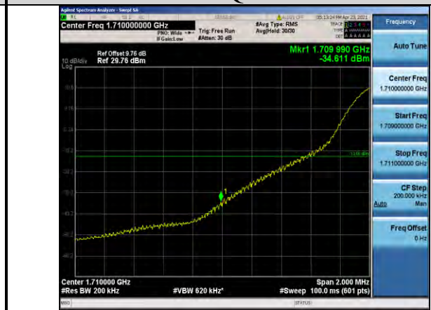
Band4-20MHz-QPSK-20050-1RB#0
