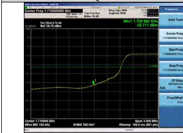
Band4-10MHz-QPSK-20000-50RB#0
