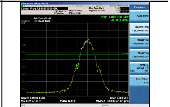
GSM1900-512
