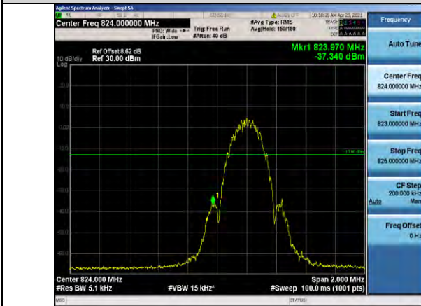
EGPRS850-128
