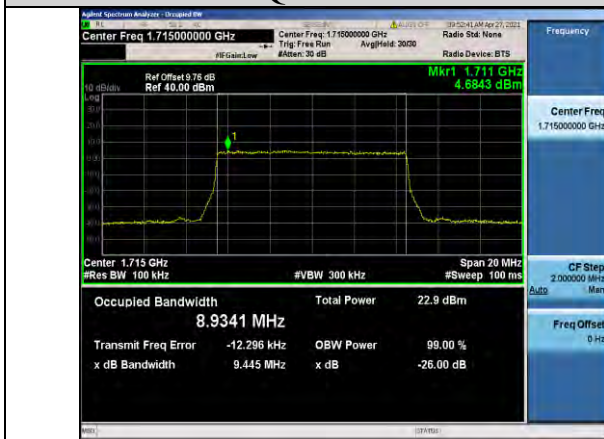
Band66-10MHz-QPSK-132022-50RB#0-8.9341
