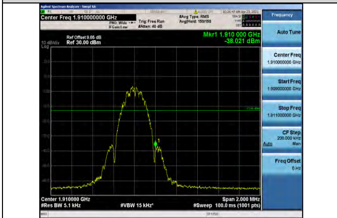
EGPRS1900-810
