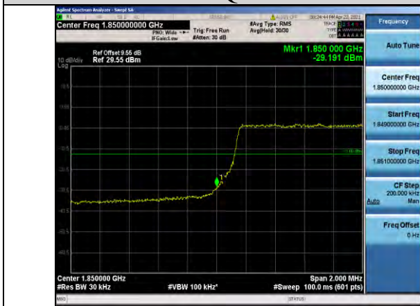
Band2-3MHz-16QAM-18615-15RB#0
