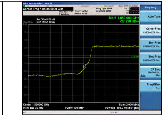
Band2-3MHz-QPSK-18615-15RB#0
