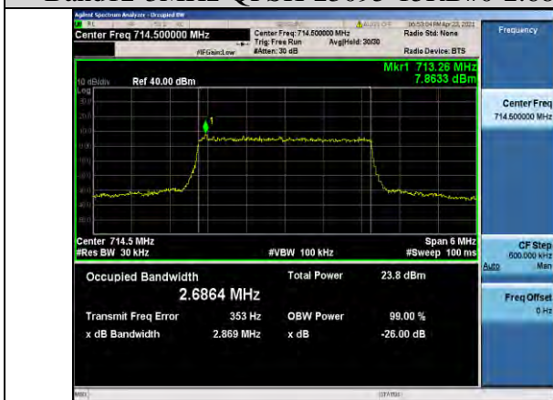
Band12-3MHz-QPSK-23165-15RB#0-2.6864
