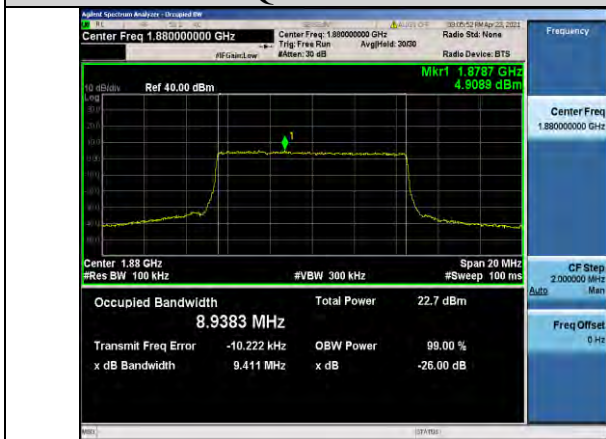
Band2-10MHz-QPSK-18900-50RB#0-8.9383
