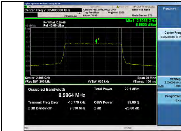
Band7-10MHz-QPSK-20800-50RB#0-8.9864
