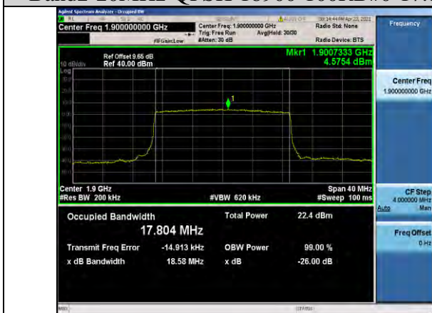
Band2-20MHz-QPSK-19100-100RB#0-17.804
