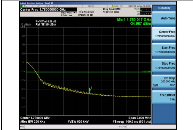
Band66-20MHz-QPSK-132572-100RB#0
