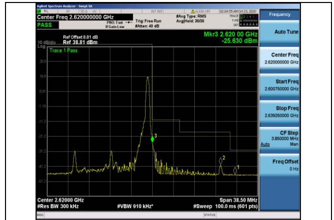
Band38-15MHz-QPSK-38175-1RB#74
