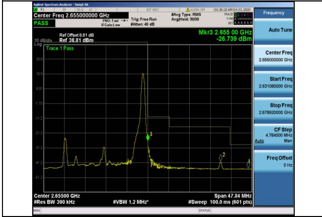
Band41-20MHz-QPSK-41140-1RB#99
