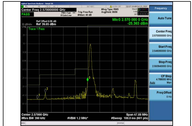
Band38-20MHz-QPSK-37850-1RB#0
