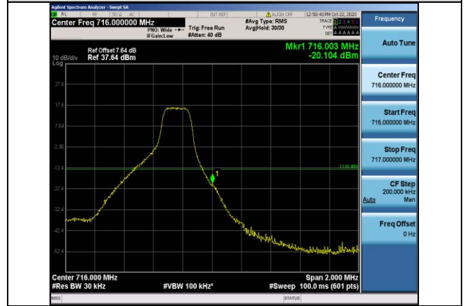
Band12-3MHz-QPSK-23165-1RB#14
