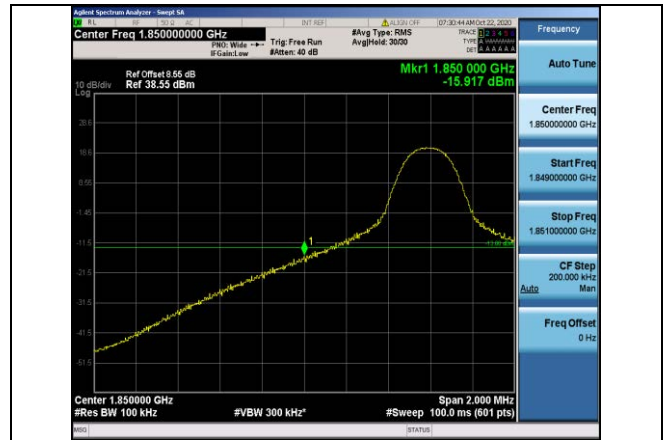
Band2-10MHz-QPSK-18650-1RB#0
