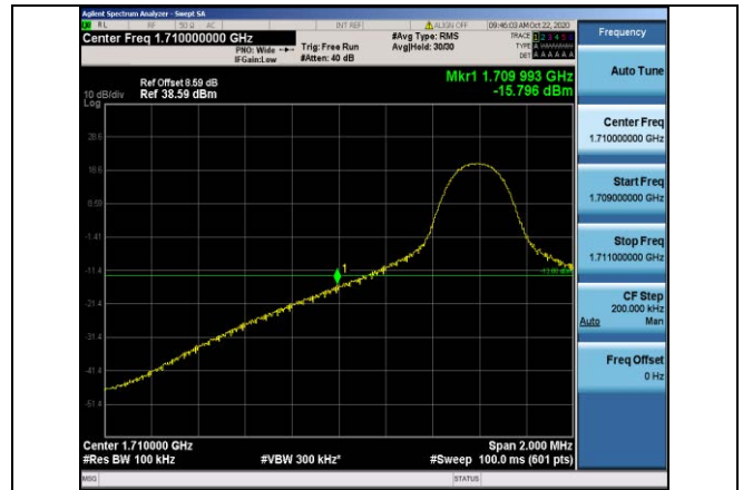
Band4-10MHz-QPSK-20000-1RB#0
