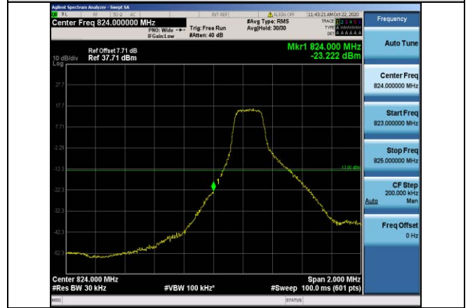
Band5-3MHz-QPSK-20415-1RB#0
