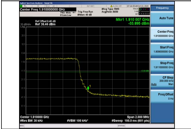
Band2-3MHz-QPSK-19185-15RB#0
