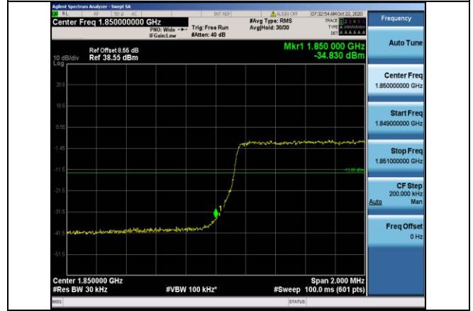
Band2-3MHz-16QAM-18615-15RB#0
