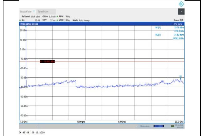
Band66-5MHz-QPSK-132647-1RB#0- Range2:1000~20000MHz
