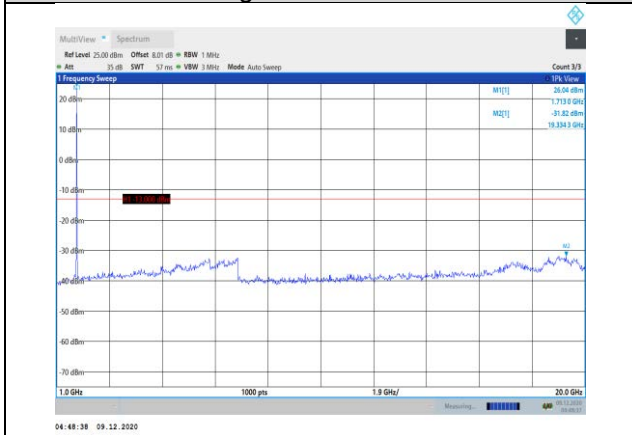
Band66-10MHz-QPSK-132022-1RB#0- Range2:1000~20000MHz
