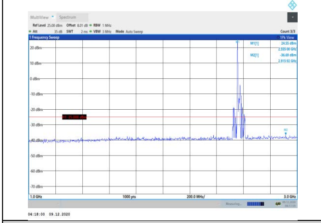
Band41-10MHz-QPSK-40290-1RB#0- Range2:1000~3000MHz
