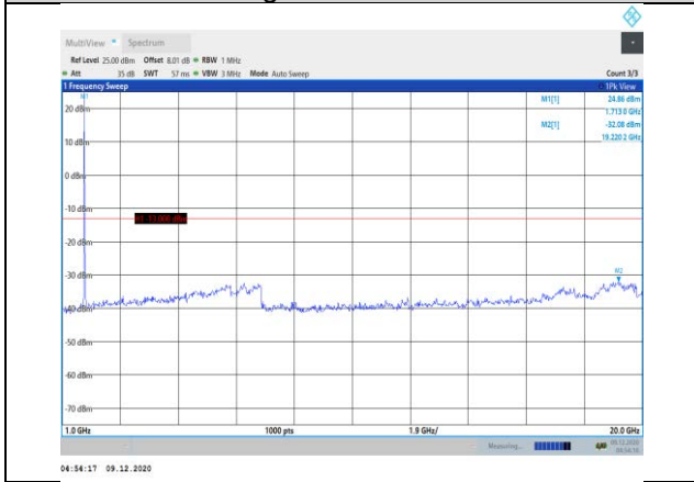
Band66-20MHz-16QAM-132072-1RB#0- Range2:1000~20000MHz
