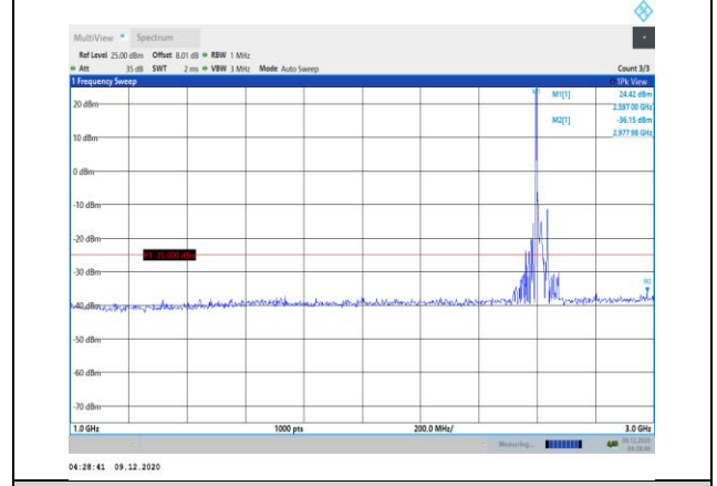
Band41-20MHz-QPSK-40740-1RB#0- Range2:1000~3000MHz
