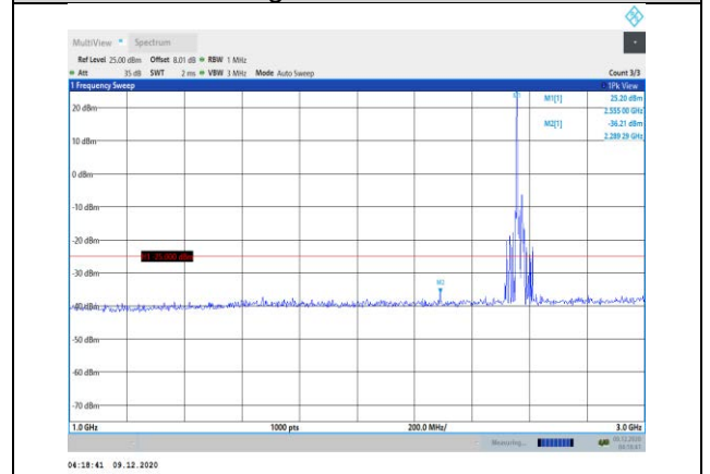
Band41-10MHz-16QAM-40290-1RB#0- Range2:1000~3000MHz
