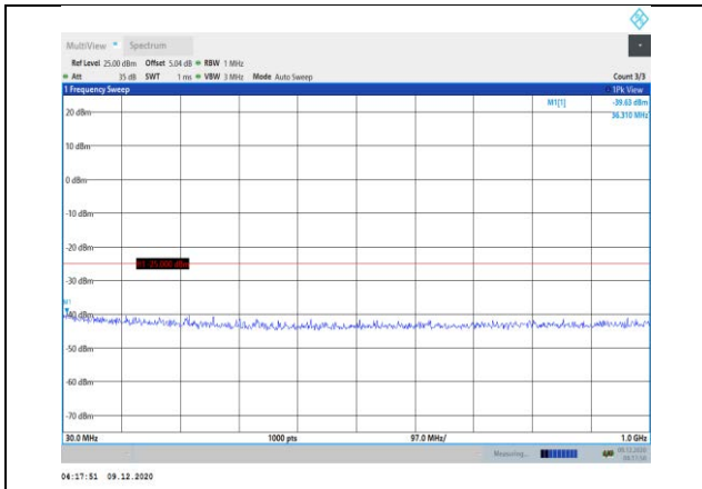
Band41-10MHz-QPSK-40290-1RB#0- Range1:30~1000MHz
