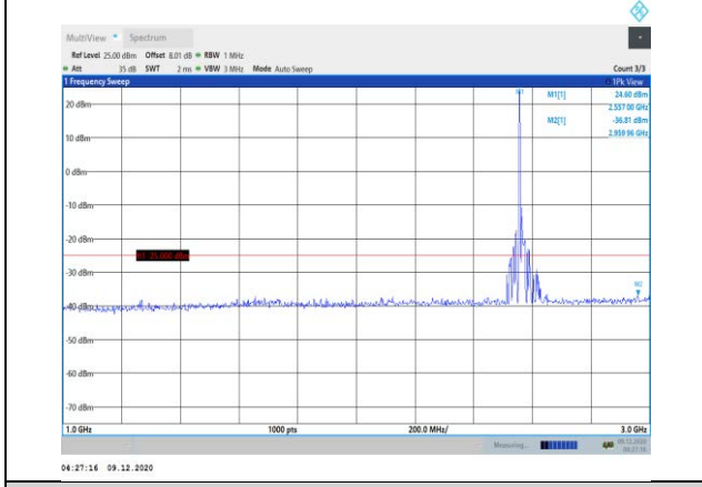
Band41-20MHz-QPSK-40340-1RB#0- Range2:1000~3000MHz
