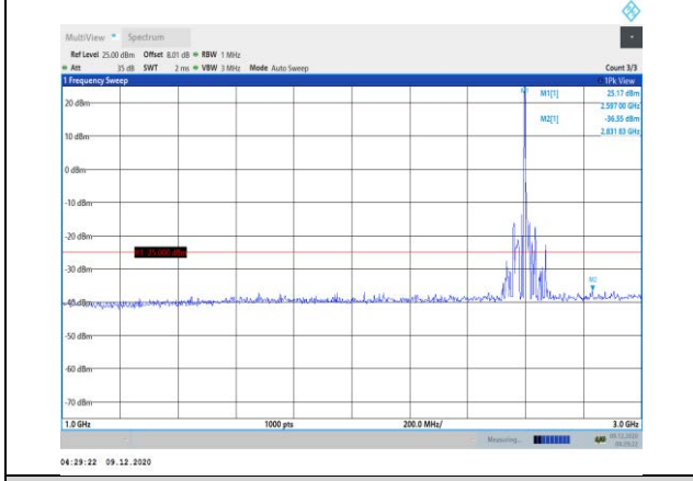
Band41-20MHz-16QAM-40740-1RB#0-Range2:1000~3000MHz
