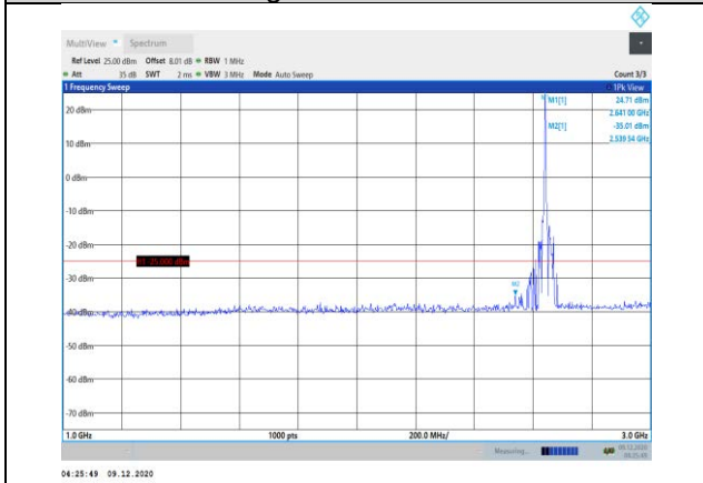
Band41-15MHz-QPSK-41165-1RB#0- Range2:1000~3000MHz
