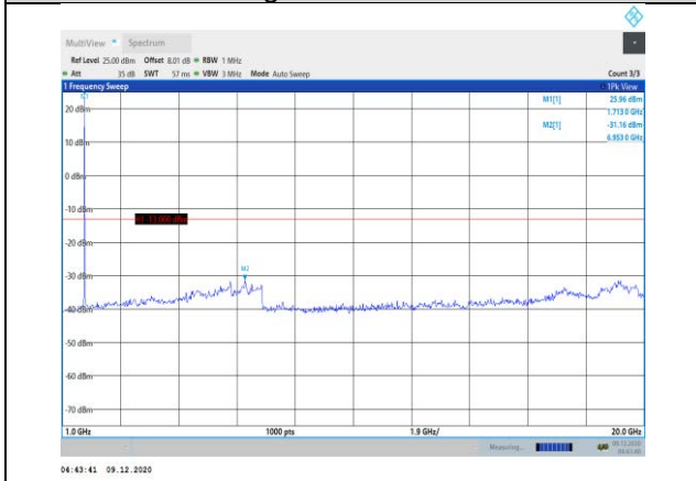
Band66-5MHz-QPSK-131997-1RB#0- Range2:1000~20000MHz
