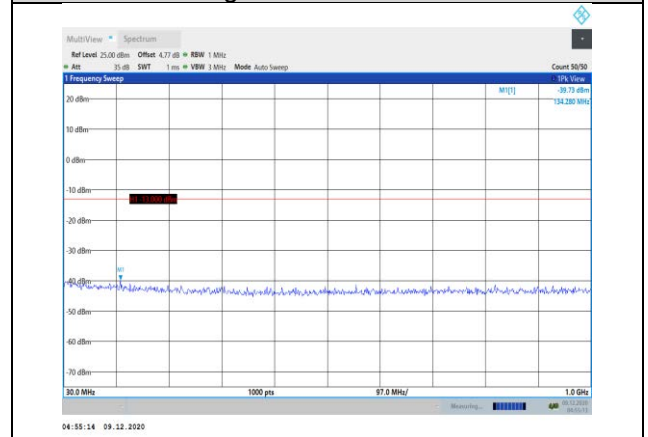
Band66-20MHz-QPSK-132572-1RB#0- Range1:30~1000MHz
