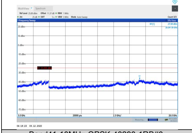
Band41-10MHz-QPSK-40290-1RB#0- Range3:3000~26000MHz
