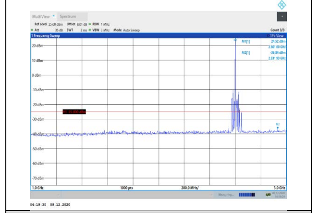
Band41-10MHz-QPSK-40740-1RB#0- Range2:1000~3000MHz
