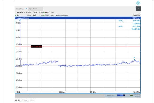
Band66-20MHz-QPSK-132572-1RB#0- Range2:1000~20000MHz
