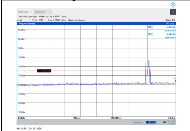
Band41-10MHz-QPSK-41190-1RB#0- Range2:1000~3000MHz
