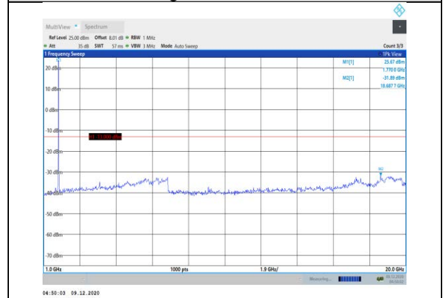
Band66-10MHz-QPSK-132622-1RB#0- Range2:1000~20000MHz
