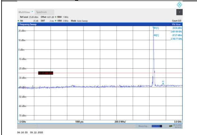
Band41-5MHz-QPSK-41215-1RB#0-Range2:1000~3000MHz
