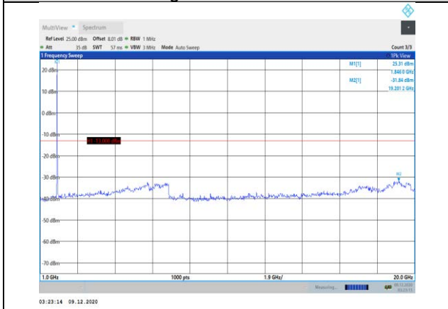
Band25-15MHz-QPSK-26115-1RB#0- Range2:1000~20000MHz
