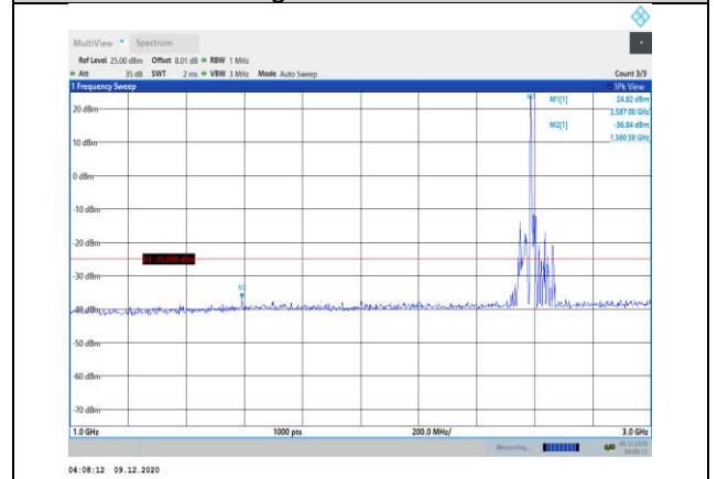
Band38-20MHz-QPSK-38000-1RB#0- Range2:1000~3000MHz
