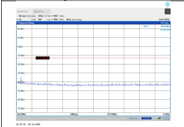
Band25-20MHz-QPSK-26365-1RB#0- Range1:30~1000MHz
