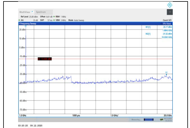
Band25-10MHz-16QAM-26365-1RB#0-Range2:1000~20000MHz
