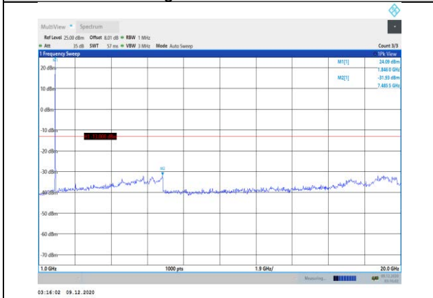
Band25-5MHz-QPSK-26065-1RB#0- Range2:1000~20000MHz
