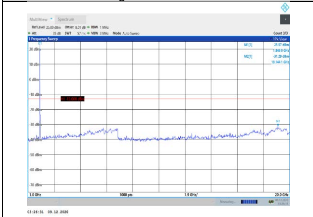
Band25-20MHz-QPSK-26140-1RB#0- Range2:1000~20000MHz
