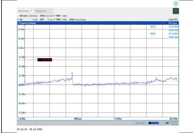
Band25-10MHz-QPSK-26090-1RB#0-Range2:1000~20000MHz
