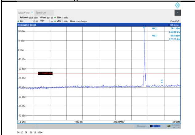
Band41-5MHz-QPSK-40265-1RB#0- Range2:1000~3000MHz
