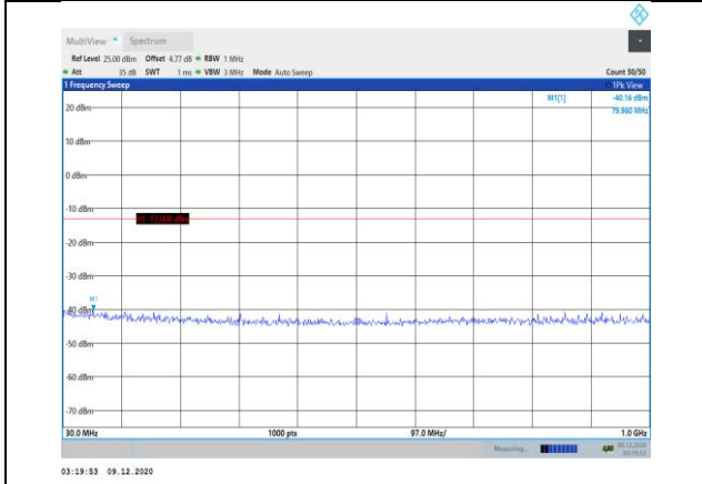
Band25-10MHz-QPSK-26365-1RB#0-Range1:30~1000MHz
