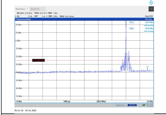
Band38-20MHz-QPSK-38150-1RB#0- Range2:1000~3000MHz
