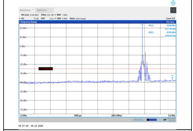
Band38-20MHz-16QAM-37850-1RB#0- Range2:1000~3000MHz
