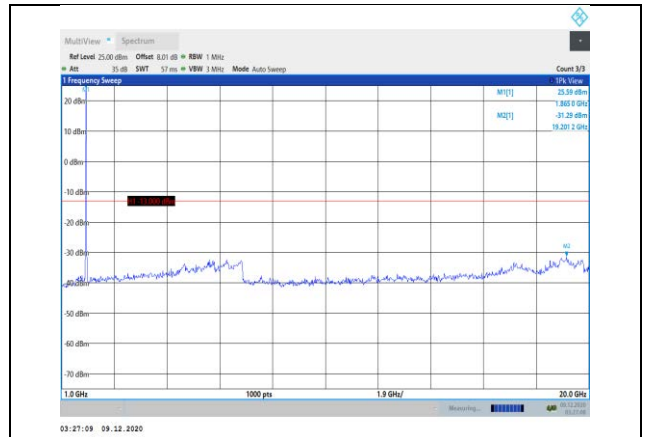
Band25-20MHz-QPSK-26365-1RB#0- Range2:1000~20000MHz
