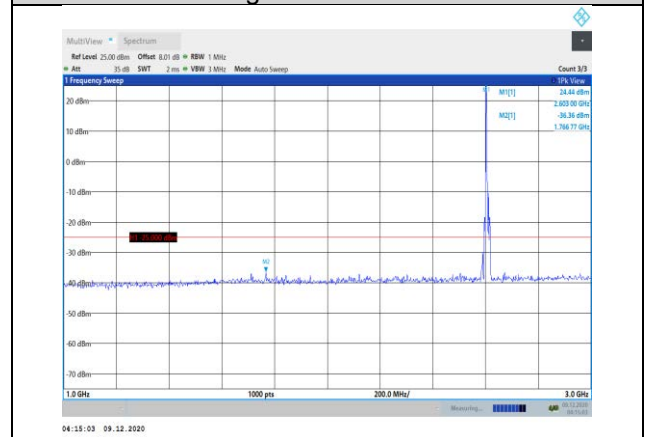
Band41-5MHz-QPSK-40740-1RB#0- Range2:1000~3000MHz
