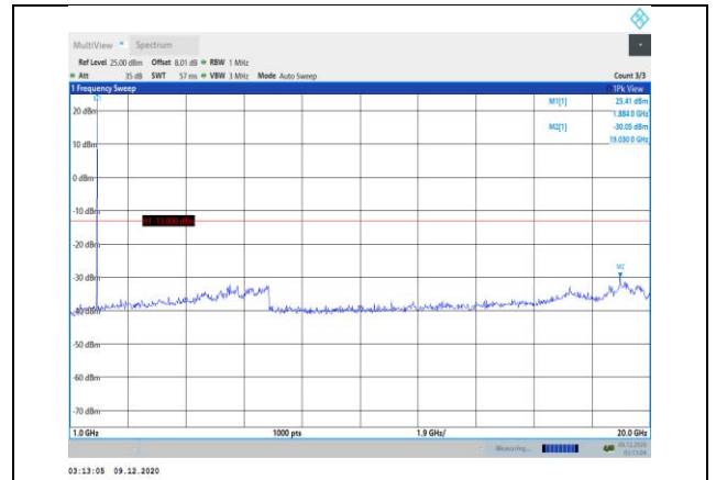
Band25-3MHz-QPSK-26365-1RB#0- Range2:1000~20000MHz
