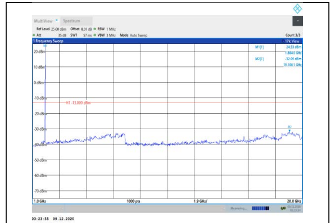
Band25-15MHz-QPSK-26365-1RB#0- Range2:1000~20000MHz
