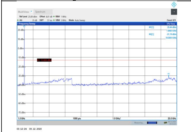
Band25-3MHz-QPSK-26055-1RB#0- Range2:1000~20000MHz
