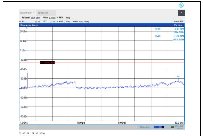
Band25-10MHz-QPSK-26365-1RB#0-Range2:1000~20000MHz
