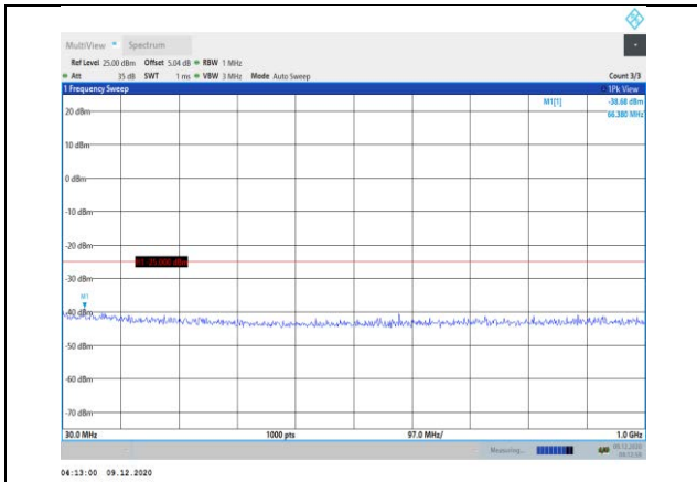
Band41-5MHz-QPSK-40265-1RB#0- Range1:30~1000MHz
