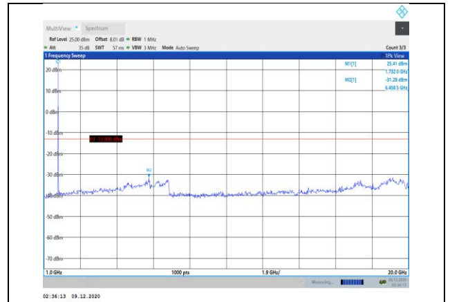
Band4-5MHz-QPSK-20175-1RB#0- Range2:1000~20000MHz
