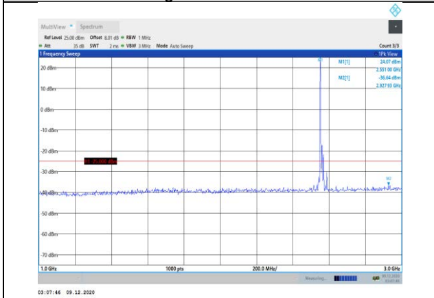
Band7-20MHz-QPSK-21350-1RB#0- Range2:1000~3000MHz
