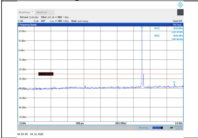
Band7-10MHz-QPSK-20800-1RB#0- Range2:1000~3000MHz
