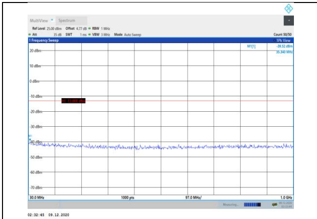
Band4-3MHz-QPSK-19965-1RB#0- Range1:30~1000MHz
