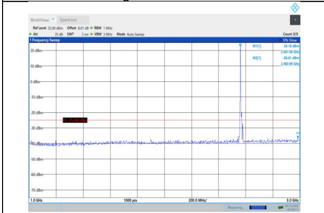
Band7-10MHz-QPSK-21400-1RB#0- Range2:1000~3000MHz
