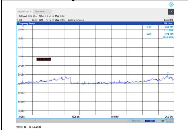
Band4-20MHz-QPSK-20050-1RB#0-Range2:1000~20000MHz
