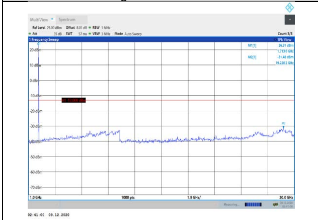
Band4-10MHz-QPSK-20000-1RB#0-Range2:1000~20000MHz
