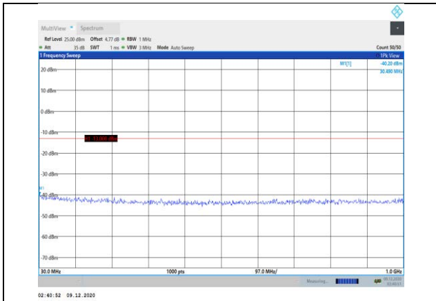
Band4-10MHz-QPSK-20000-1RB#0-Range1:30~1000MHz
