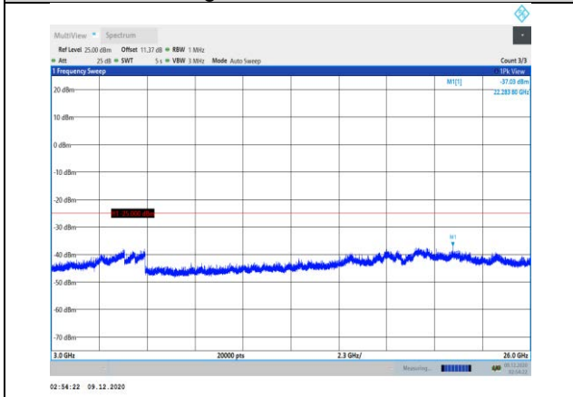
Band7-10MHz-QPSK-20800-1RB#0- Range3:3000~26000MHz
