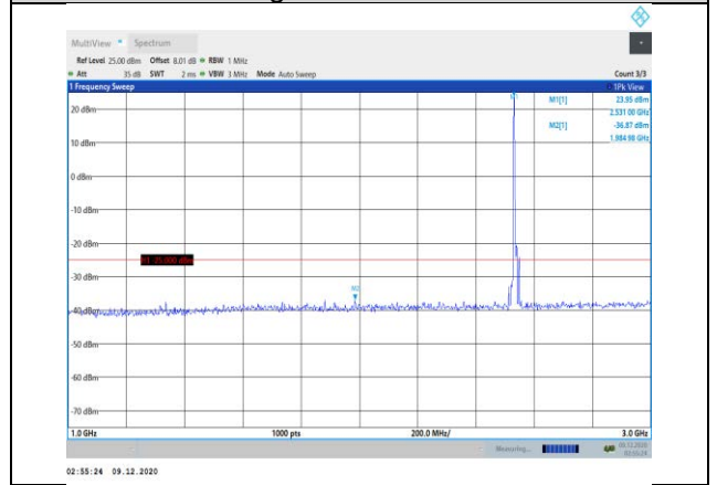
Band7-10MHz-QPSK-21100-1RB#0- Range2:1000~3000MHz
