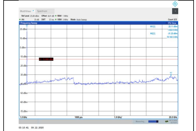
Band25-1.4MHz-QPSK-26683-1RB#0-Range2:1000~20000MHz
