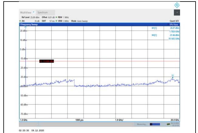
Band4-3MHz-QPSK-20175-1RB#0- Range2:1000~20000MHz
