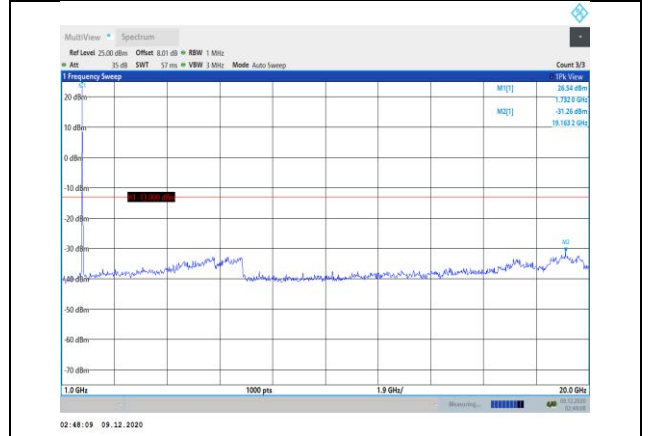
Band4-20MHz-QPSK-20300-1RB#0-Range2:1000~20000MHz
