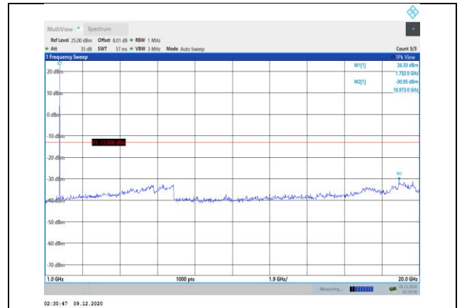
Band4-1.4MHz-QPSK-20175-1RB#0- Range2:1000~20000MHz
