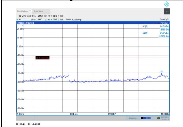
Band25-1.4MHz-QPSK-26047-1RB#0-Range2:1000~20000MHz
