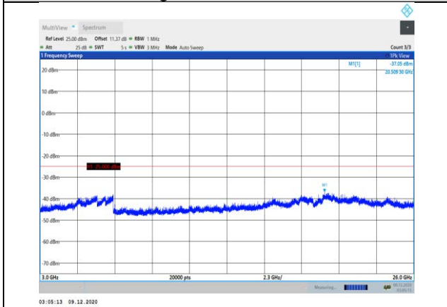
Band7-20MHz-QPSK-20850-1RB#0- Range3:3000~26000MHz
