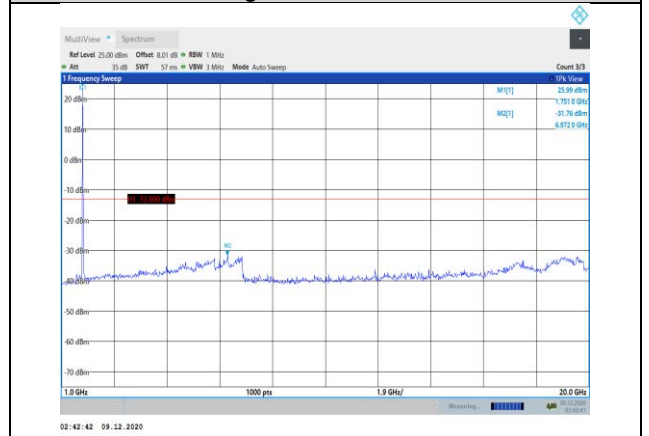
Band4-10MHz-QPSK-20350-1RB#0-Range2:1000~20000MHz
