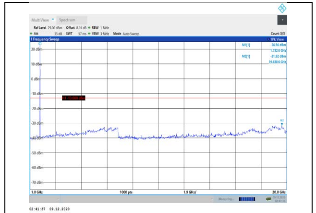
Band4-10MHz-QPSK-20175-1RB#0-Range2:1000~20000MHz
