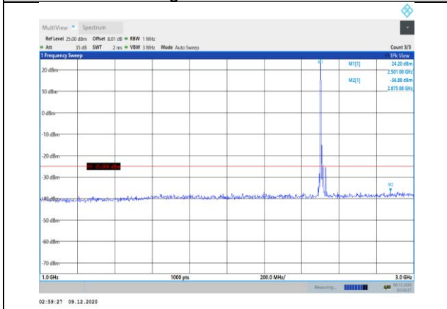
Band7-15MHz-QPSK-20825-1RB#0- Range2:1000~3000MHz
