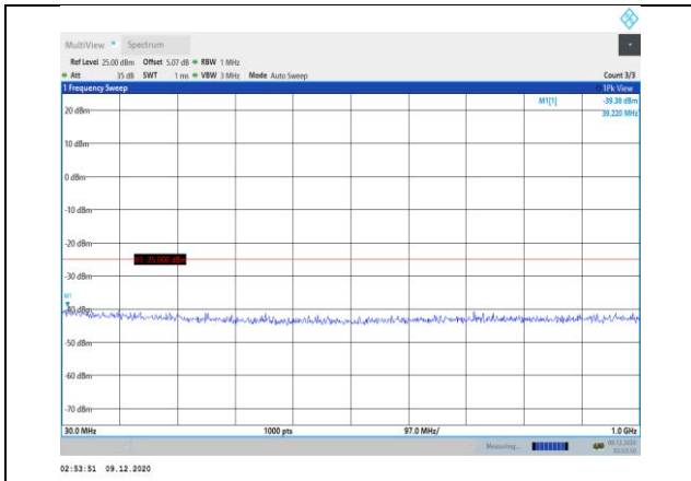
Band7-10MHz-QPSK-20800-1RB#0- Range1:30~1000MHz
