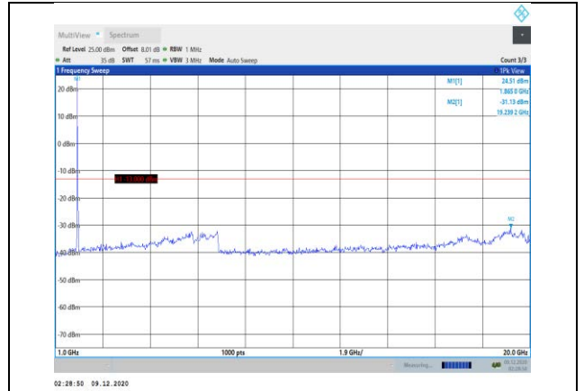
Band2-20MHz-16QAM-18900-1RB#0- Range2:1000~20000MHz
