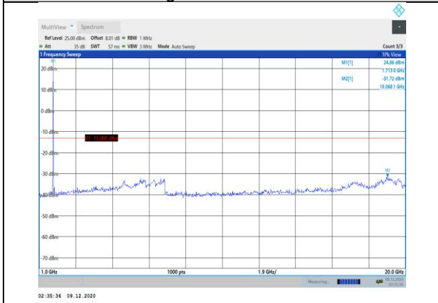
Band4-5MHz-QPSK-19975-1RB#0- Range2:1000~20000MHz
