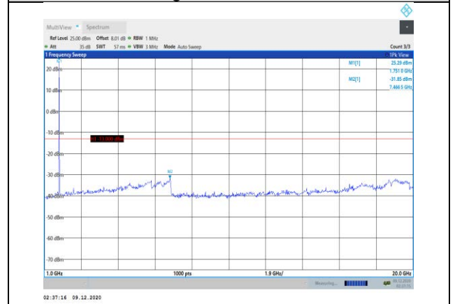
Band4-5MHz-QPSK-20375-1RB#0- Range2:1000~20000MHz
