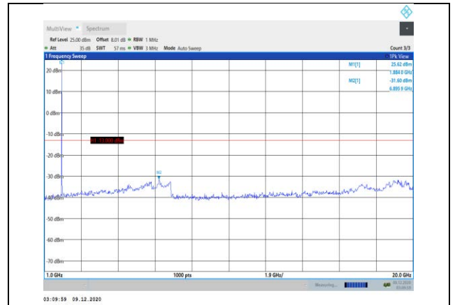
Band25-1.4MHz-QPSK-26365-1RB#0-Range2:1000~20000MHz
