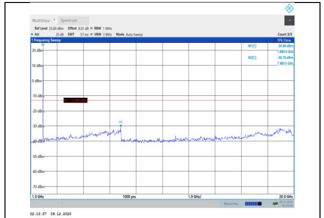
Band2-3MHz-QPSK-18900-1RB#0- Range2:1000~20000MHz
