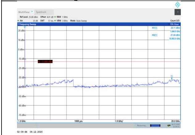
Band2-3MHz-QPSK-18615-1RB#0- Range2:1000~20000MHz
