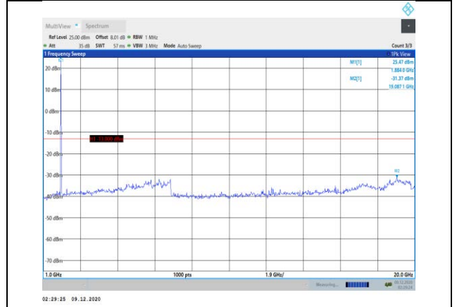
Band2-20MHz-QPSK-19100-1RB#0- Range2:1000~20000MHz
