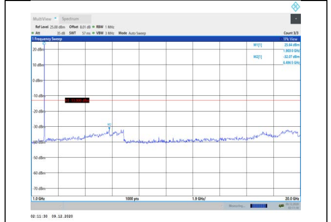
Band2-3MHz-QPSK-19185-1RB#0- Range2:1000~20000MHz
