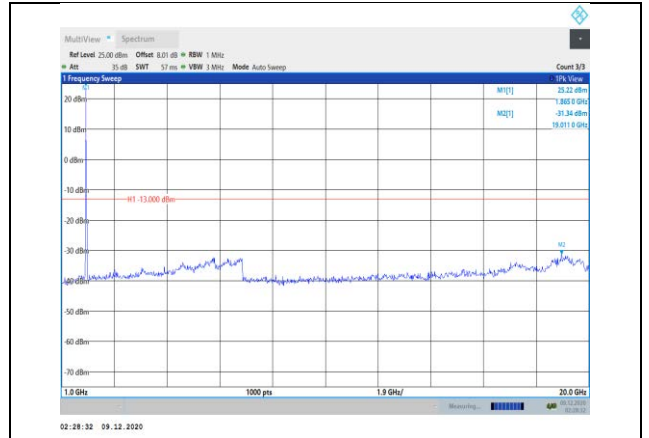
Band2-20MHz-QPSK-18900-1RB#0- Range2:1000~20000MHz
