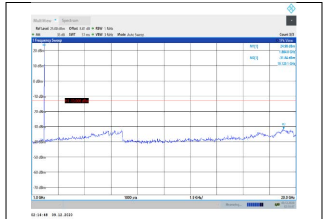
Band2-5MHz-QPSK-18900-1RB#0- Range2:1000~20000MHz
