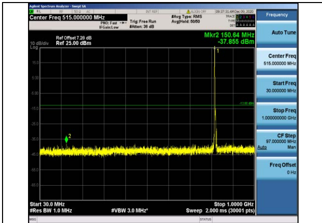
Band26-5MHz-QPSK-26765-1RB#0- Range1:30~1000MHz
