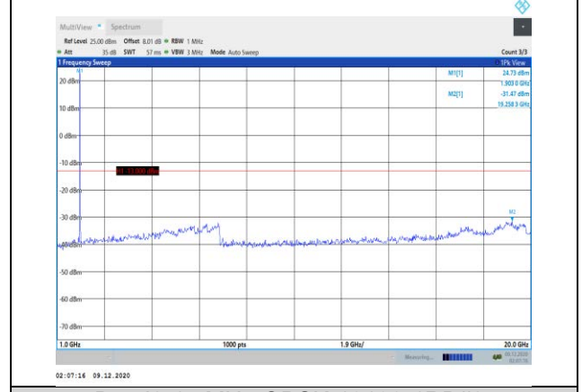
Band2-1.4MHz-QPSK-19193-1RB#0-Range2:1000~20000MHz
