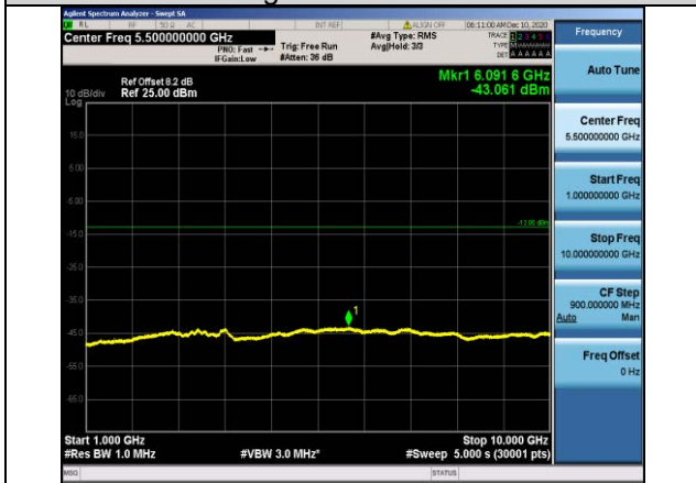
Band13-5MHz-QPSK-23230-1RB#0-Range2:1000~10000MHz
