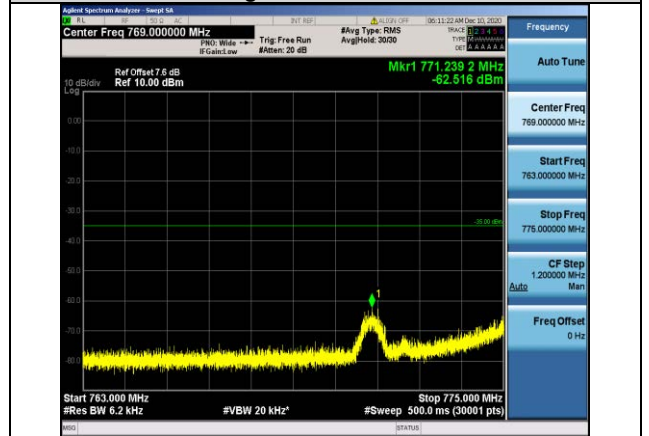
Band13-5MHz-QPSK-23230-1RB#0-Range3:763~775MHz
