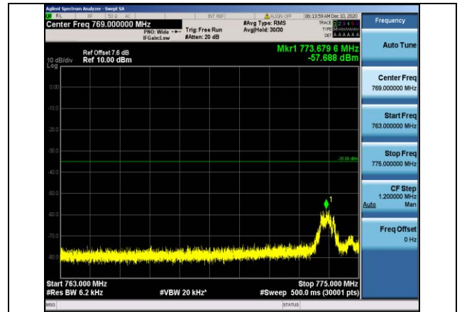
Band13-5MHz-QPSK-23255-1RB#0-Range3:763~775MHz
