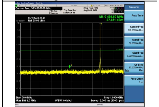
Band13-5MHz-QPSK-23230-1RB#0-Range1:30~1000MHz
