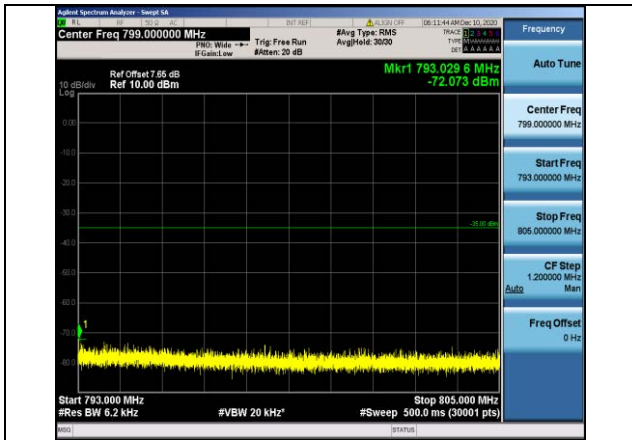
Band13-5MHz-QPSK-23230-1RB#0-Range4:793~805MHz
