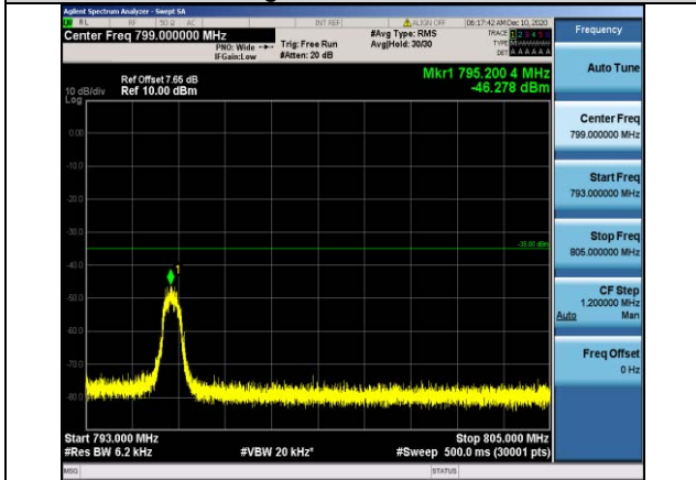
Band13-10MHz-QPSK-23230-1RB#0- Range4:793~805MHz
