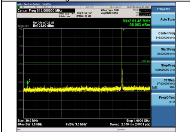
Band13-5MHz-QPSK-23255-1RB#0-Range1:30~1000MHz
