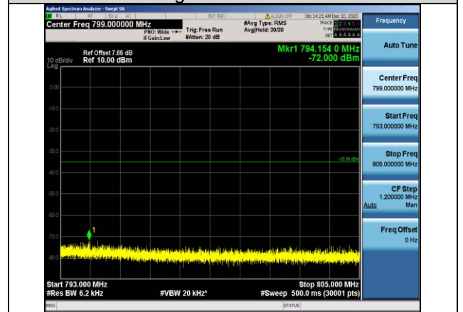
Band13-5MHz-QPSK-23255-1RB#0-Range4:793~805MHz
