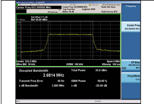
Band26-3MHz-QPSK-26775-15RB#0-2.6814
