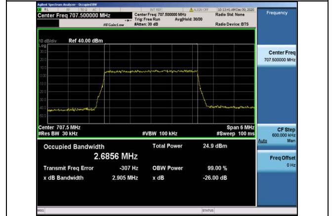
Band12-3MHz-QPSK-23095-15RB#0-2.6856
