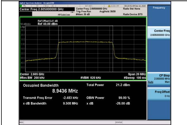
Band41-10MHz-QPSK-40740-50RB#0-8.9436
