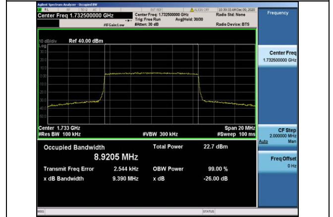
Band4-10MHz-QPSK-20175-50RB#0-8.9205
