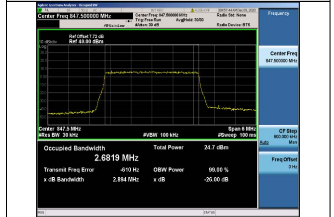
Band5-3MHz-QPSK-20635-15RB#0-2.6819
