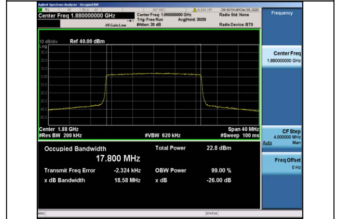
Band2-20MHz-QPSK-18900-100RB#0-17.800
