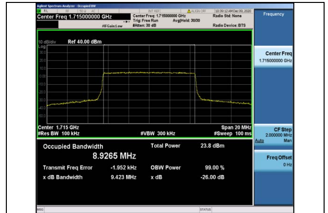
Band4-10MHz-QPSK-20000-50RB#0-8.9265
