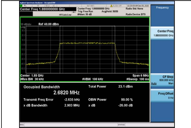
Band2-3MHz-16QAM-18900-15RB#0-2.6820
