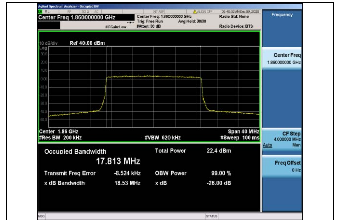
Band2-20MHz-QPSK-18700-100RB#0-17.813
