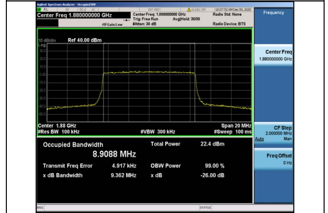
Band2-10MHz-QPSK-18900-50RB#0-8.9088
