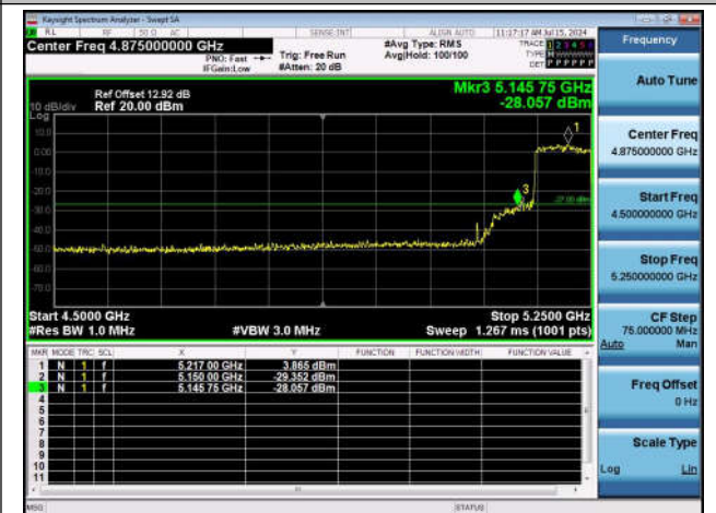
11AC80SISO-Ant1-5210-PASS
