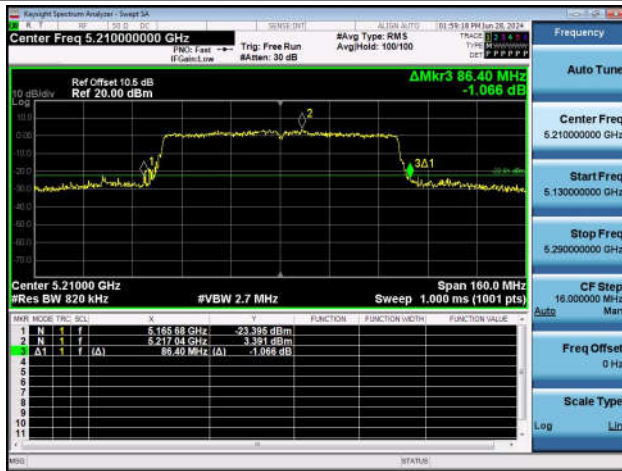
11AC80SISO-Ant1-5210-26dB EBW
