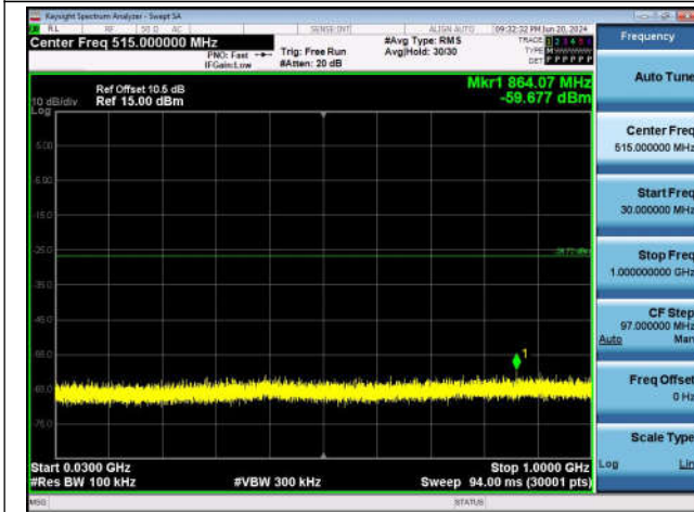
11G-Ant1-2462-30~1000-PASS
