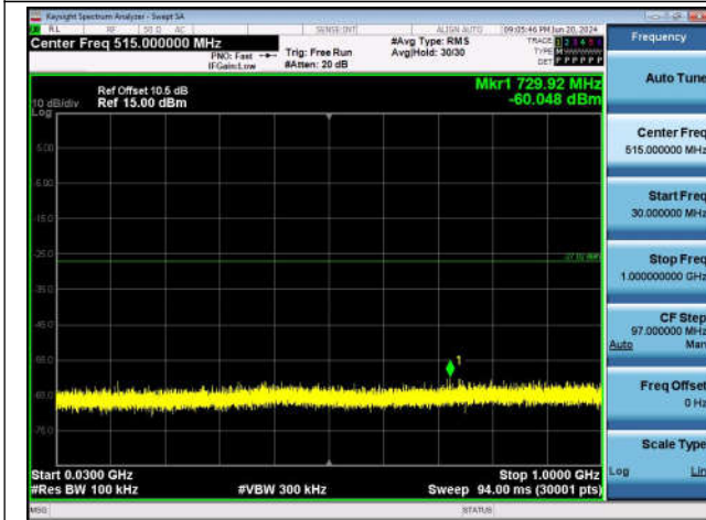
11G-Ant1-2412-30~1000-PASS
