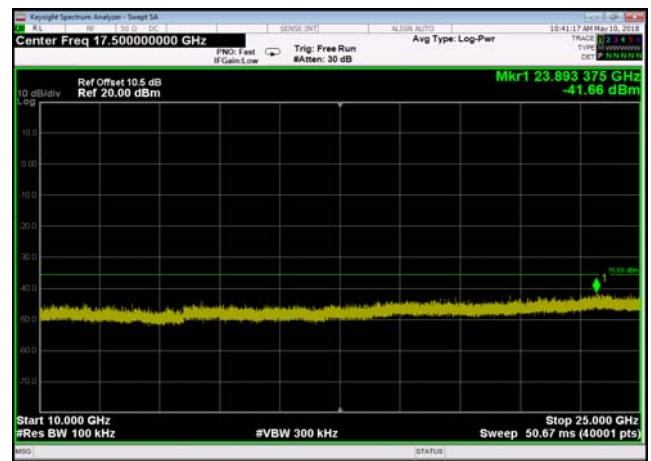
802.11n(HT40),2452MHz,Ant0,Plot 5,10000MHz~25000MHz
