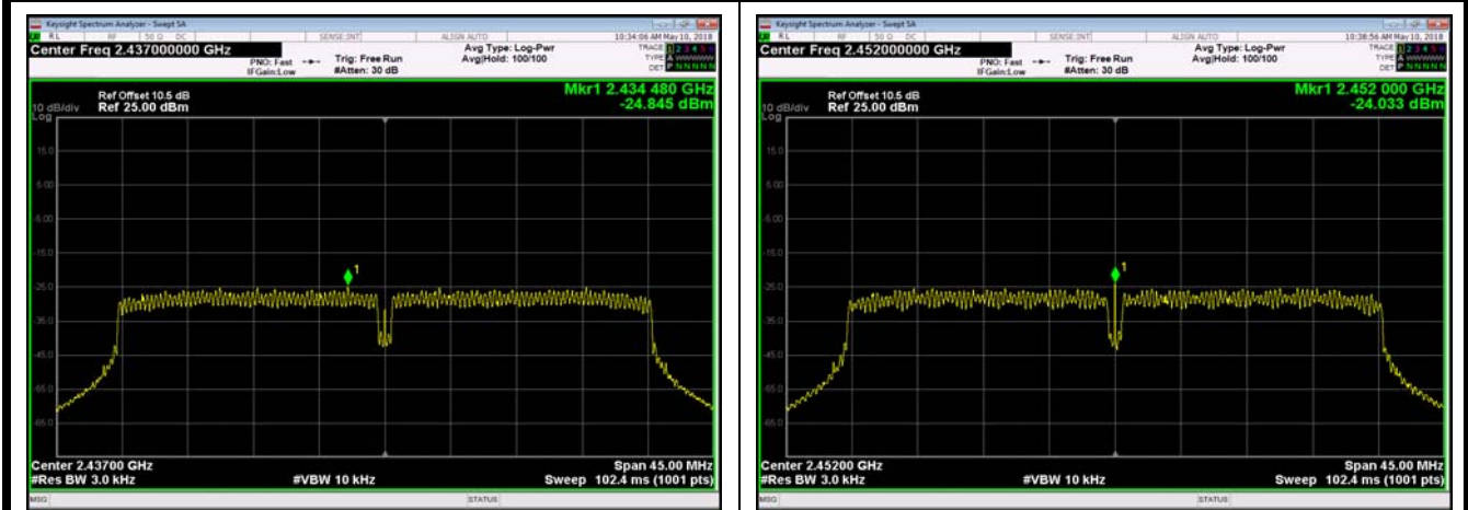
802.11n(HT40),2437MHz,Ant0
