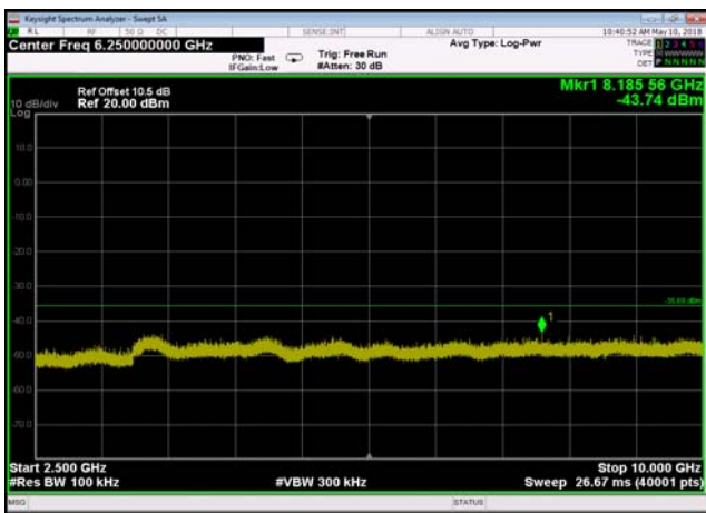
802.11n(HT40),2452MHz,Ant0,Plot 4,2500MHz~10000MHz
