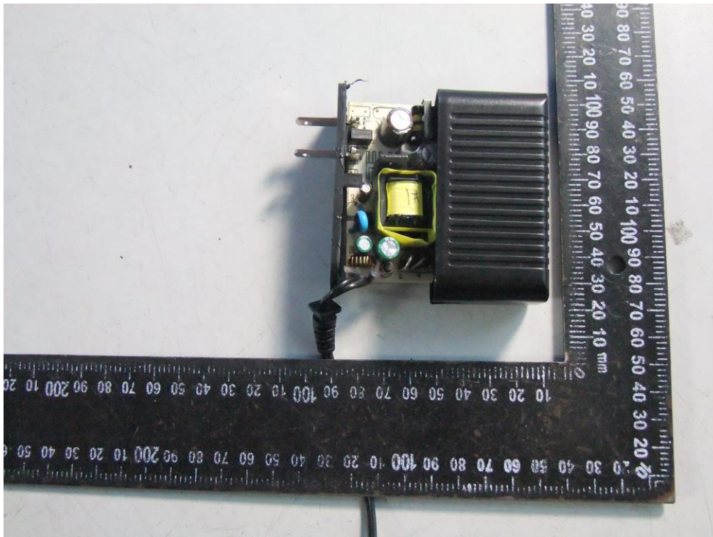
Adapter -- ZAU-A050260A-04
