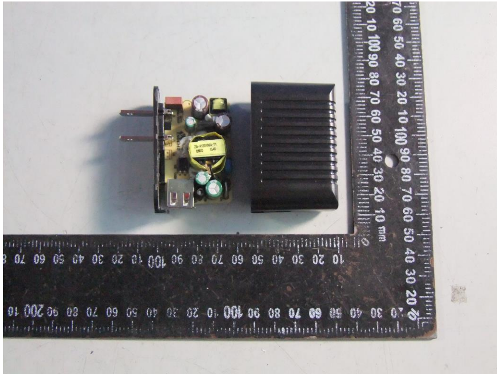
Adapter -- ZAU-A050150A-02
