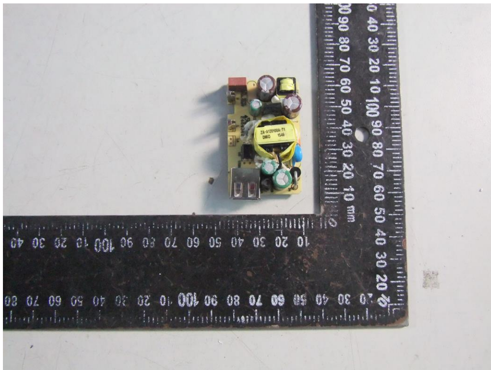
Adapter -- ZAU-A050150A-02
