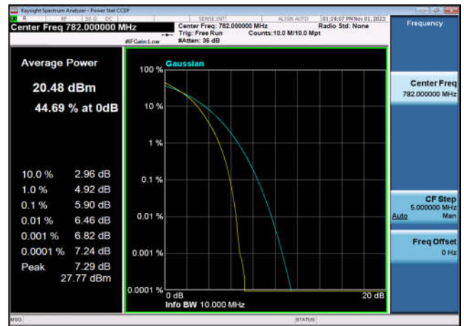
FDD13_HighRange_10MHz_782_fullIRB_Q16
