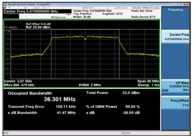
U-NII-2c 99% OBW & 26dB EBW-802.11n(40MHz) ,5670MHz,Ant1
