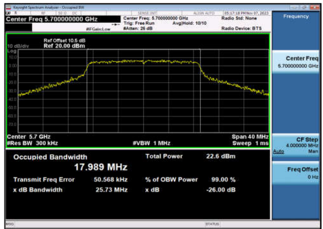
U-NII-2c 99% OBW & 26dB EBW-802.11ac(20MHz) ,5700MHz,Ant1
