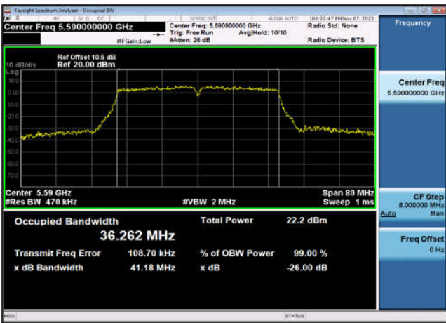
U-NII-2c 99% OBW & 26dB EBW-802.11n(40MHz) ,5590MHz,Ant1
