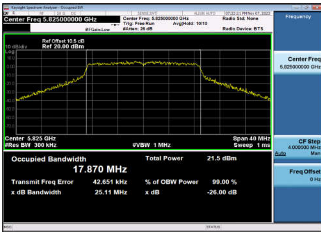
U-NII-3 99% OBW & 26dB EBW-802.11ac(20MHz) ,5825MHz,Ant1
