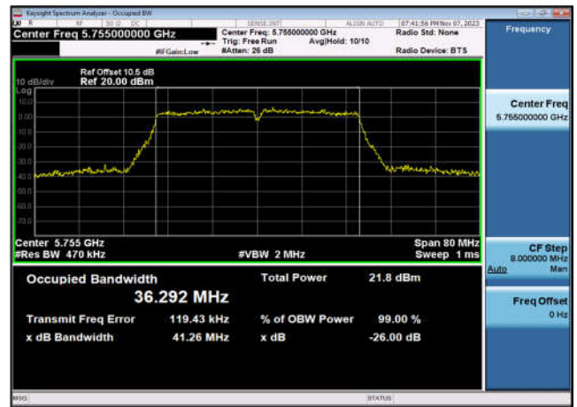
U-NII-3 99% OBW & 26dB EBW-802.11ac(40MHz) ,5755MHz,Ant1
