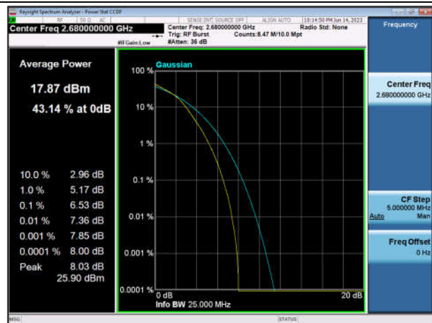
TDD41_HighRange_20MHz_2680_fullRB_Q16
