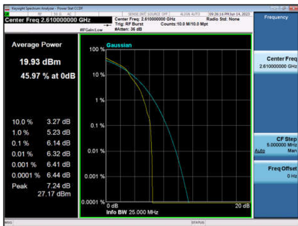
TDD38_HighRange_20MHz_2610_OneRB_high_Q16
