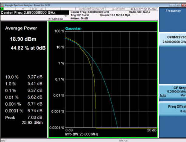
TDD41_HighRange_20MHz_2680_OneRB_high_Q16
