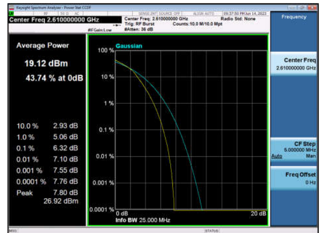
TDD38_HighRange_20MHz_2610_fullIRB_Q16
