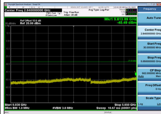
U-NII-3 ,Plot 2,30MHz~5650MHz-802.11a c(40MHz),5755MHz,Ant1
