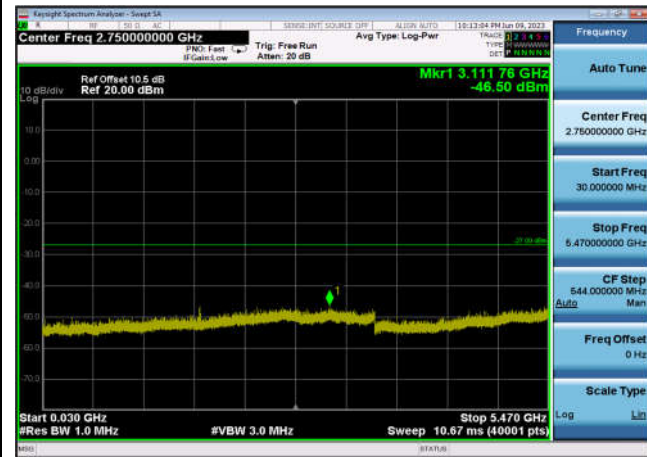
U-NII-2c ,Plot 2,30MHz~5470MHz-802.11 ac(80MHz),5530MHz,Ant1
