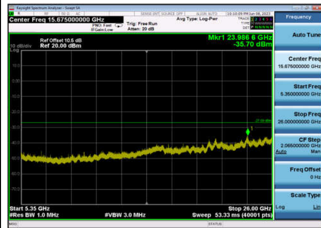
U-NII-2a ,Plot 3,5350MHz~26000MHz-802 .11n(20MHz),5320MHz,Ant1
