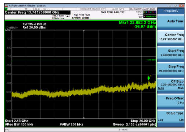
,Plot 4,2483.5MHz~25000MHz-802.11n(HT20),2462MHz,Ant0
