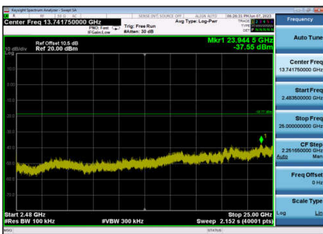
,Plot 4,2483.5MHz~25000MHz-802.11n(HT40),2437MHz,Ant0
