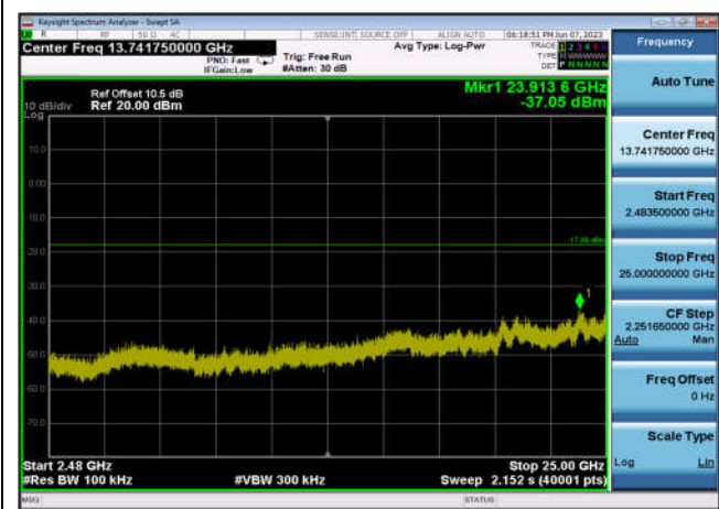
,Plot 4,2483.5MHz~25000MHz-802.11n(HT40),2452MHz,Ant0
