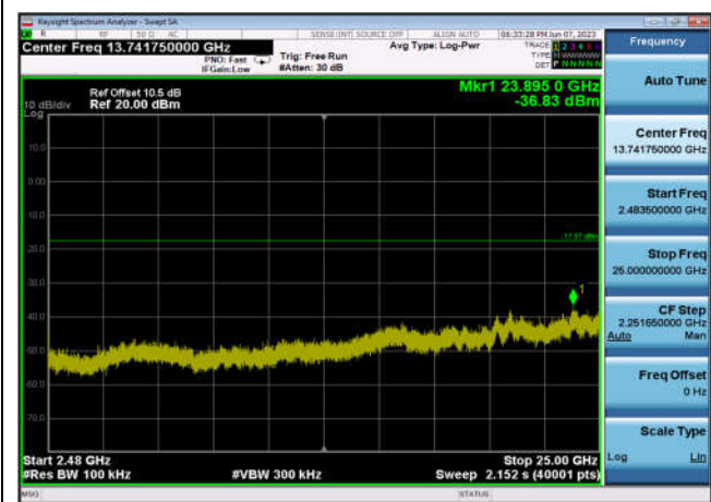
,Plot 4,2483.5MHz~25000MHz-802.11n(HT40),2452MHz,Ant0
