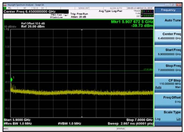
U-NII-3 ,Plot 3,5900MHz~7000MHz-802.1 1ac(20MHz),5745MHz,Ant2
