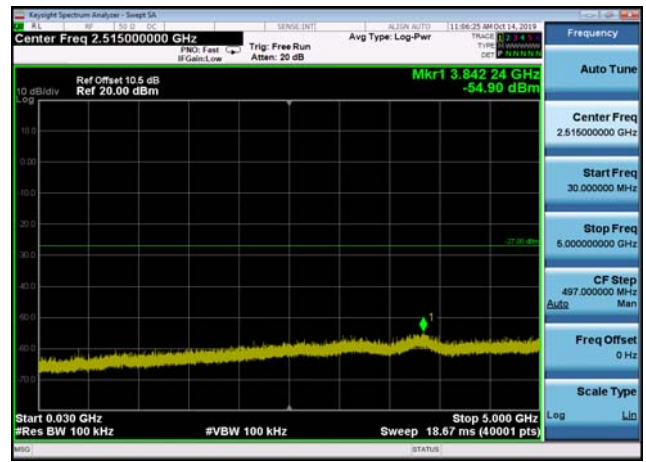
U-NII-3 ,Plot 2,30MHz~5000MHz-802.11a c(20MHz),5785MHz,Ant2
