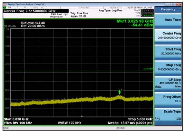
U-NII-3 ,Plot 2,30MHz~5000MHz-802.11a c(40MHz),5795MHz,Ant2
