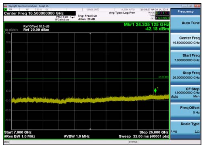
U-NII-3 ,Plot 4,7000MHz~26000MHz-802. 11ac(20MHz),5785MHz,Ant2
