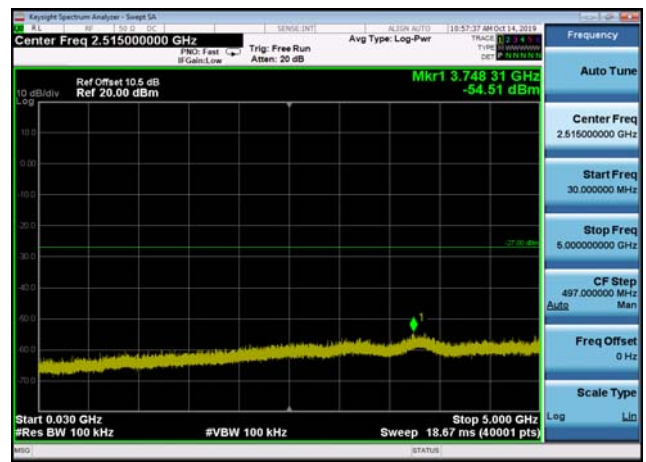
U-NII-3 ,Plot 2,30MHz~5000MHz-802.11a c(20MHz),5825MHz,Ant2
