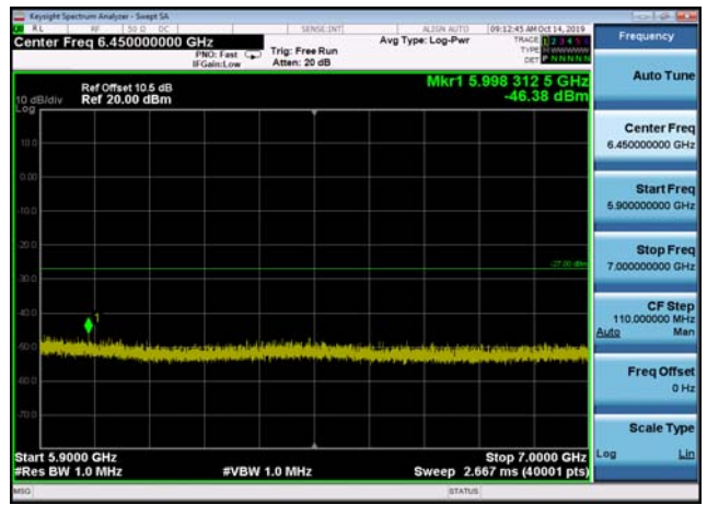
U-NII-3 ,Plot 3,5900MHz~7000MHz-802.1 1a(20MHz),5825MHz,Ant2
