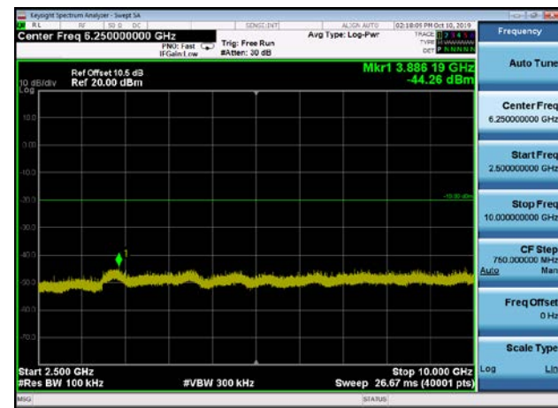
,Plot 4,2500MHz~10000MHz-802.11n(HT40),2452MHz
