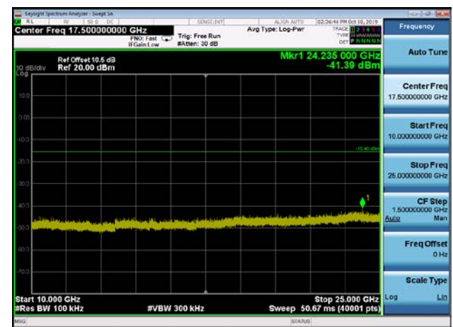
,Plot 5,10000MHz~25000MHz-802.11n(HT40),2452MHz
