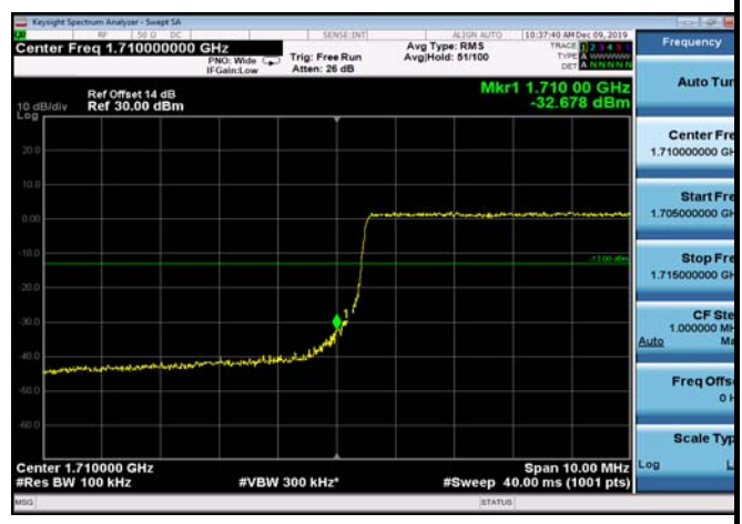
LowRange_FDD66_15MHz_1717.5_OneRB_low_Q16
