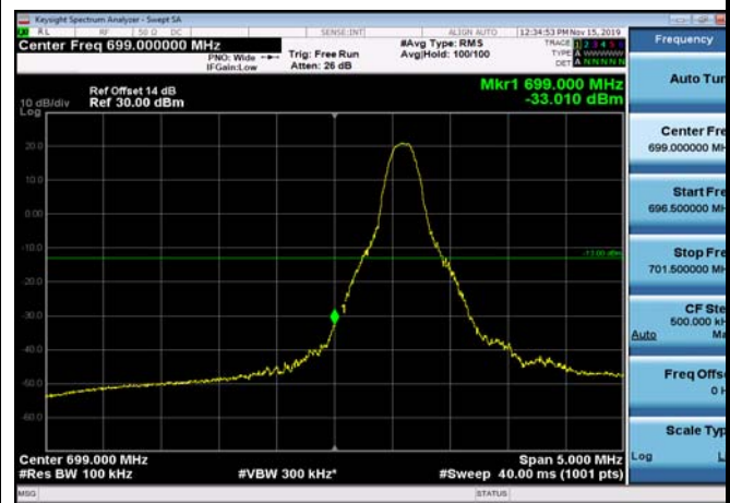
LowRange_FDD12_10MHz_704_fullRB_Low_Q16
