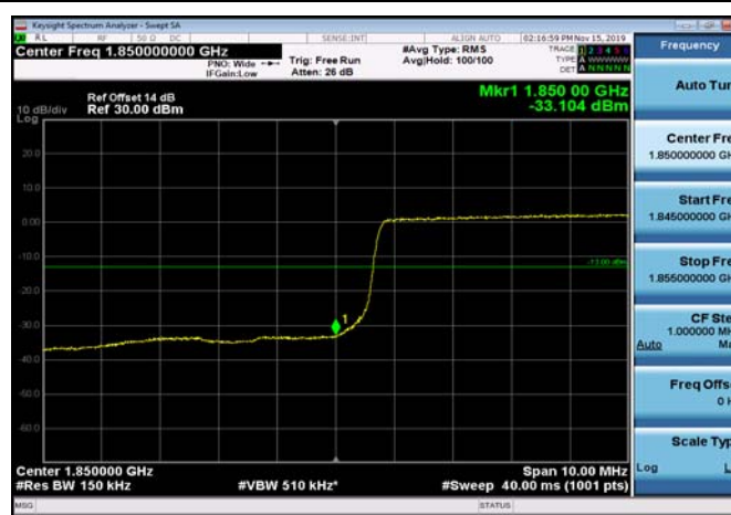
LowRange_FDD25_20MHz_1860_OneRB_low_Q16
