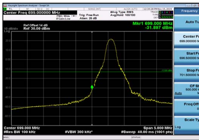
LowRange_FDD12_10MHz_704_fullRB_Low_QPSK
