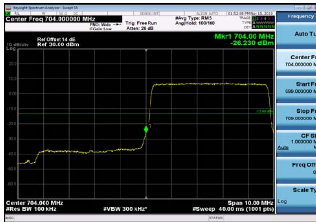
LowRange_FDD17_10MHz_709_OneRB_low_QPSK
