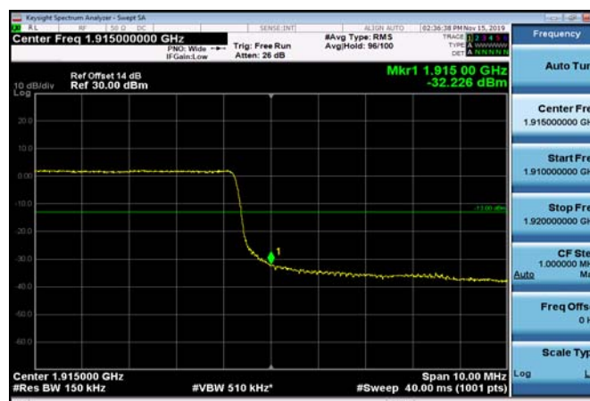
HighRange_FDD25_20MHz_1905_OneRB_high_Q16
