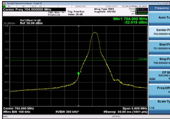
LowRange_FDD17_10MHz_709_fullRB_Low_QPSK
