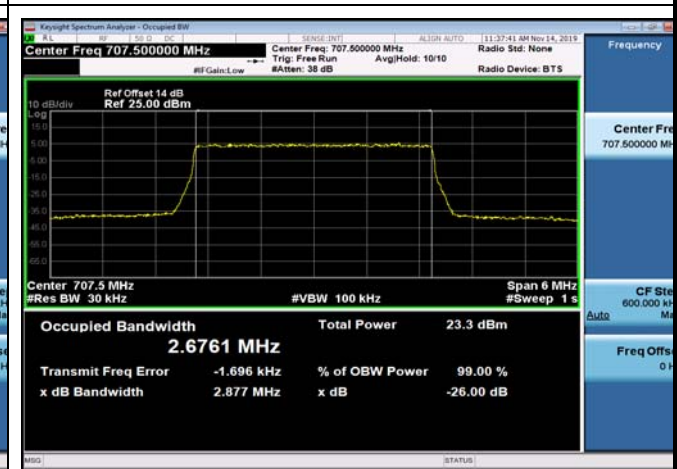
FDD12_MidRange_5_707.5_Q16
