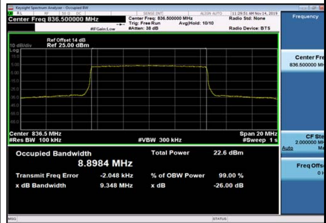
FDD07_MidRange_5_2535_Q16
