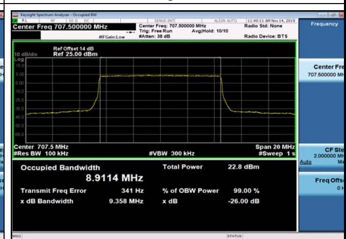
FDD12_MidRange_10_707.5_Q16
