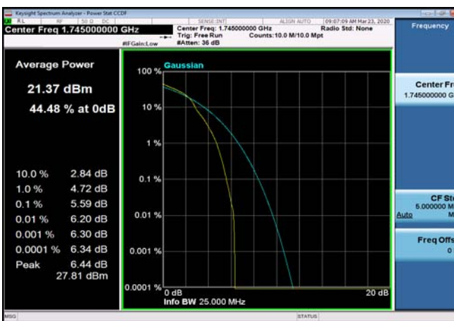
FDD04_HighRange_20MHz_1745_OneRB_high_Q16
