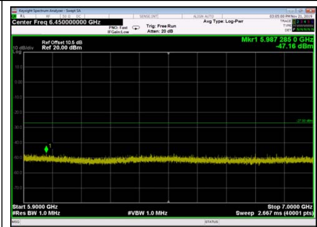
U-NII-2c ,Plot 3,5900MHz~7000MHz-802. 11ac(40MHz),5590MHz,Ant1
