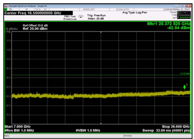
U-NII-2c ,Plot 4,7000MHz~26000MHz-802 .11ac(20MHz),5600MHz,Ant1
