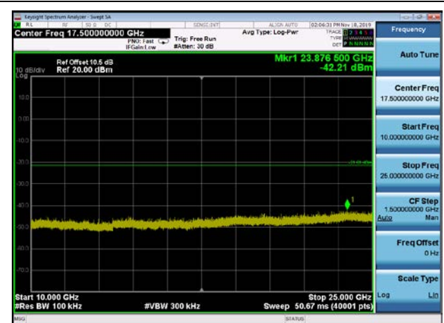
,Plot 5,10000MHz~25000MHz-802.11n(HT40),2452MHz,Ant0
