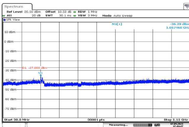
U-NII-2a,802.11ac(40MHz),5270MHz ,Ant1,Plot 2,30MHz~5150MHz
