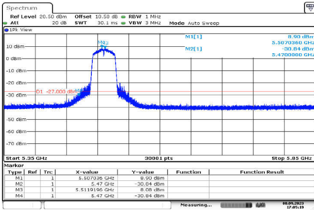
U-NII-2c,802.11ac(40MHz),5510MHz ,Ant1,Plot 1,Band Edge
