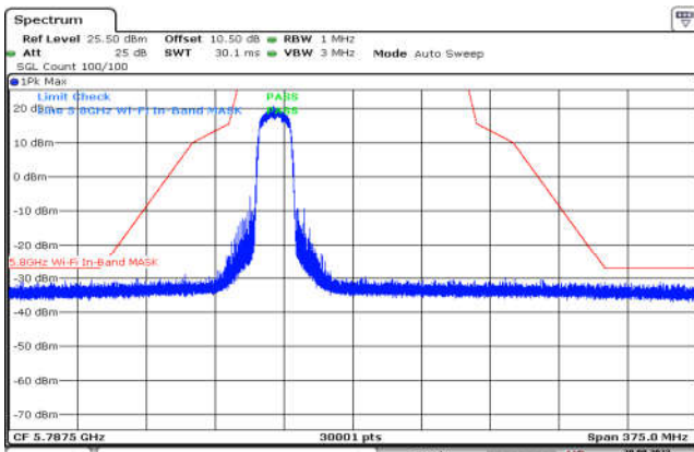
U-NII-3,802.11ac(20MHz),5825MHz ,Ant1,Plot 1,Band Edge
