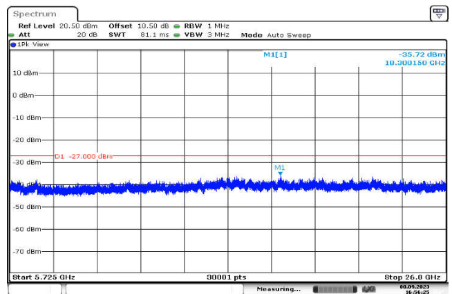
U-NII-2c,802.11ac(40MHz),5590MHz ,Ant1,Plot 3,5725MHz~26000MHz
