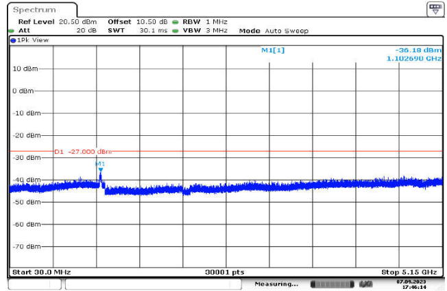
U-NII-2a,802.11ac(40MHz),5310MHz ,Ant1,Plot 2,30MHz~5150MHz
