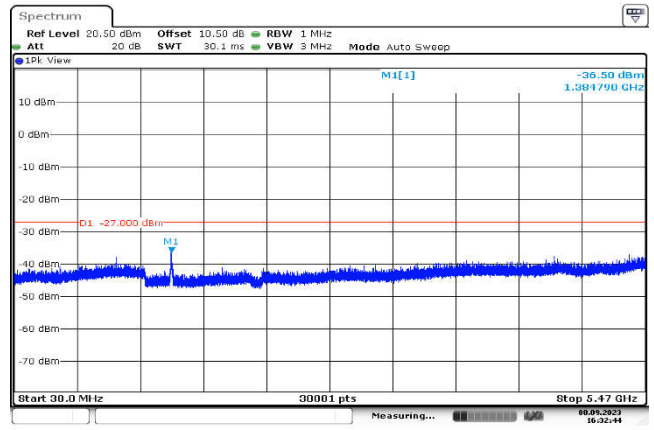
U-NII-2c,802.11n(40MHz),5590MHz ,Ant1,Plot 2,30MHz~5470MHz
