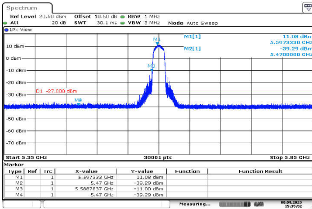
U-NII-2c,802.11ac(20MHz),5600MHz ,Ant1,Plot 1,Band Edge
