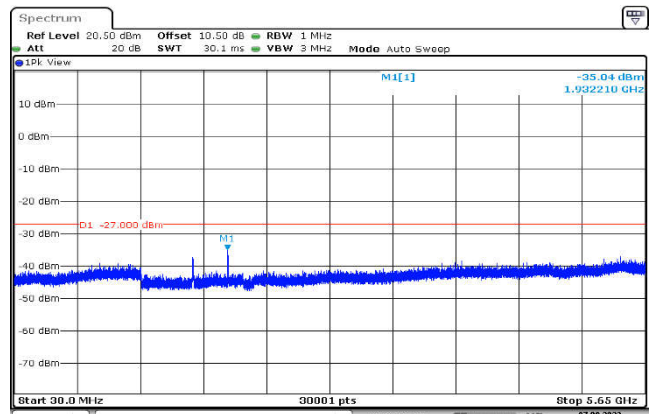
U-NII-3,802.11ac(20MHz),5825MHz ,Ant1,Plot 2,30MHz~5650MHz
