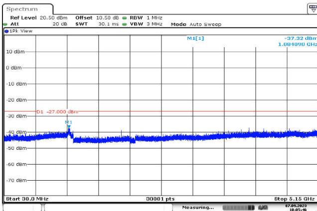
U-NII-2a,802.11ac(80MHz),5290MHz ,Ant1,Plot 2,30MHz~5150MHz
