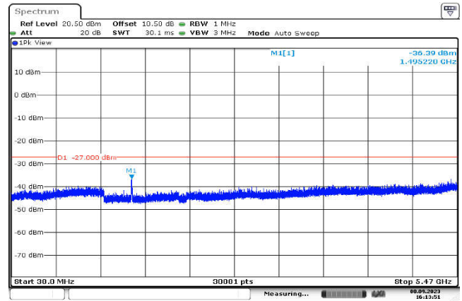
U-NII-2c,802.11n(20MHz),5700MHz ,Ant1,Plot 2,30MHz~5470MHz
