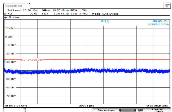
U-NII-2a,802.11ac(40MHz),5270MHz ,Ant1,Plot 3,5350MHz~26000MHz
