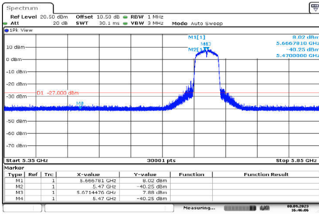
U-NII-2c,802.11ac(40MHz),5670MHz ,Ant1,Plot 1,Band Edge
