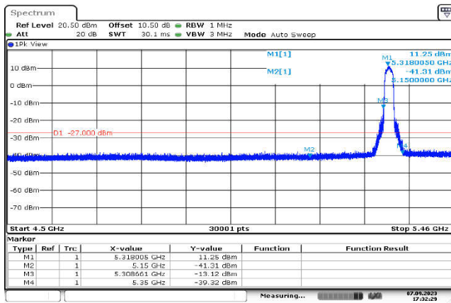
U-NII-2a,802.11ac(20MHz),5320MHz ,Ant1,Plot 1,Band Edge
