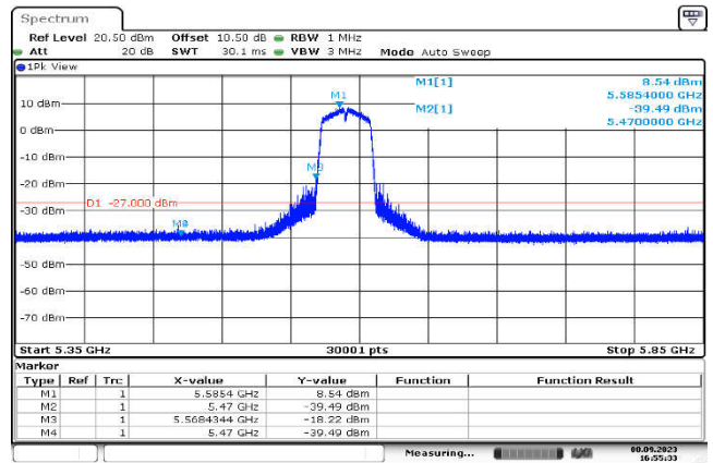
U-NII-2c,802.11ac(40MHz),5590MHz ,Ant1,Plot 1,Band Edge
