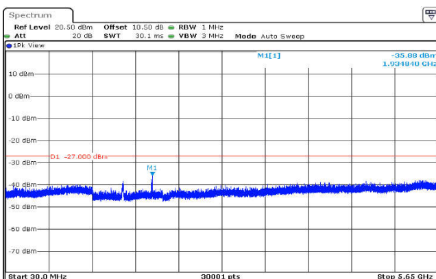
U-NII-3,802.11n(40MHz),5755MHz ,Ant1,Plot 2,30MHz~5650MHz
