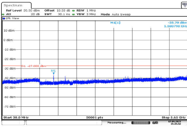
U-NII-3,802.11ac(20MHz),5785MHz ,Ant1,Plot 2,30MHz~5650MHz
