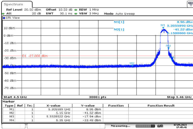
U-NII-2a,802.11ac(40MHz),5310MHz ,Ant1,Plot 1,Band Edge
