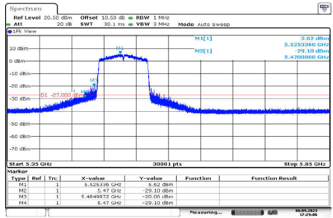
U-NII-2c,802.11ac(80MHz),5530MHz ,Ant1,Plot 1,Band Edge
