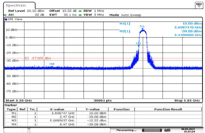
U-NII-2c,802.11ac(20MHz),5700MHz ,Ant1,Plot 1,Band Edge
