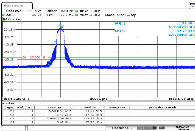
U-NII-2c,802.11n(20MHz),5500MHz ,Ant1,Plot 1,Band Edge
