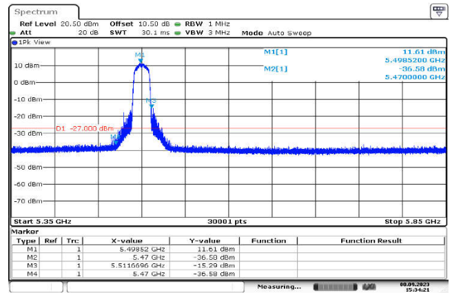
U-NII-2c,802.11ac(20MHz),5500MHz ,Ant1,Plot 1,Band Edge
