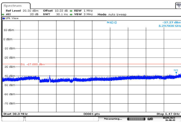
U-NII-2c,802.11n(40MHz),5670MHz ,Ant1,Plot 2,30MHz~5470MHz
