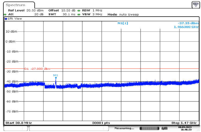
U-NII-2c,802.11ac(40MHz),5670MHz ,Ant1,Plot 2,30MHz~5470MHz
