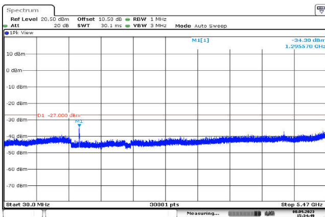
U-NII-2c,802.11ac(20MHz),5500MHz ,Ant1,Plot 2,30MHz~5470MHz
