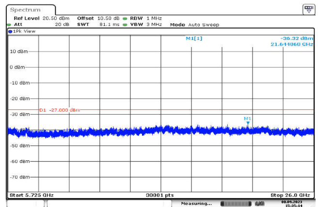
U-NII-2c,802.11ac(20MHz),5500MHz ,Ant1,Plot 3,5725MHz~26000MHz
