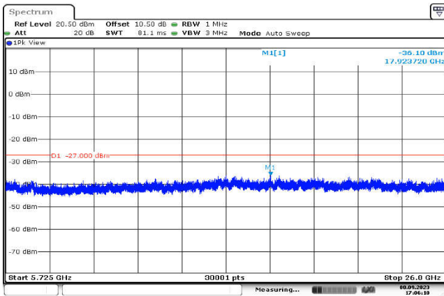
U-NII-2c,802.11ac(40MHz),5510MHz ,Ant1,Plot 3,5725MHz~26000MHz
