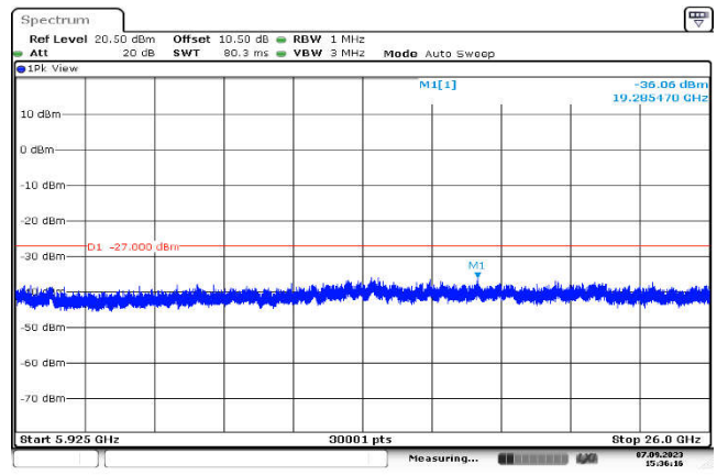
U-NII-3,802.11ac(20MHz),5785MHz ,Ant1,Plot 3,5925MHz~26000MHz
