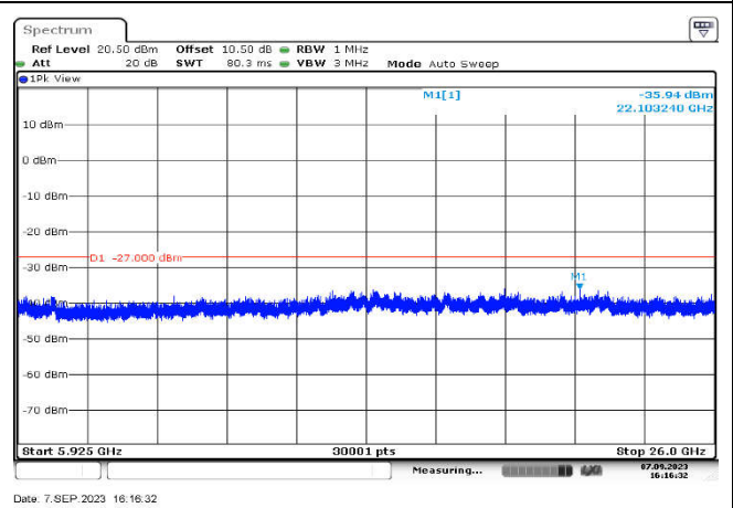
U-NII-3,802.11ac(80MHz),5775MHz ,Ant1,Plot 3,5925MHz~26000MHz
