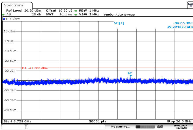
U-NII-2c,802.11ac(40MHz),5670MHz ,Ant1,Plot 3,5725MHz~26000MHz
