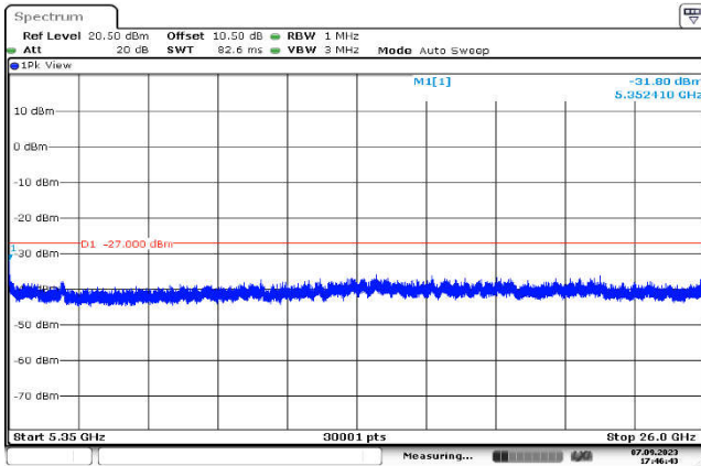
U-NII-2a,802.11ac(40MHz),5310MHz ,Ant1,Plot 3,5350MHz~26000MHz
