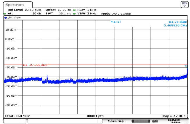
U-NII-2c,802.11ac(40MHz),5510MHz ,Ant1,Plot 2,30MHz~5470MHz
