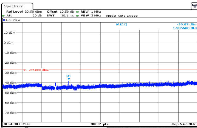
U-NII-3,802.11ac(40MHz),5755MHz ,Ant1,Plot 2,30MHz~5650MHz
