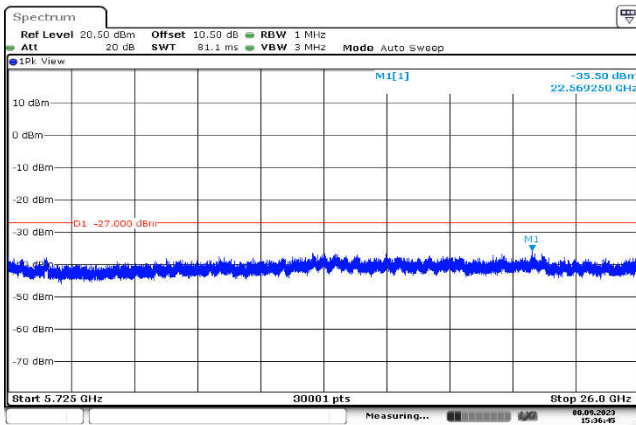
U-NII-2c,802.11ac(20MHz),5600MHz ,Ant1,Plot 3,5725MHz~26000MHz
