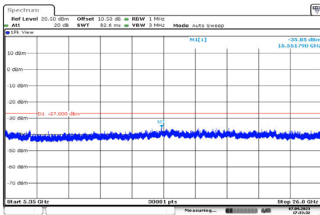
U-NII-2a,802.11ac(20MHz),5320MHz ,Ant1,Plot 3,5350MHz~26000MHz
