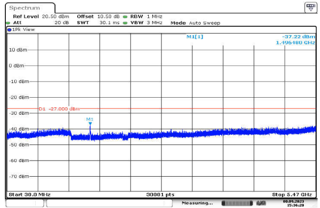
U-NII-2c,802.11ac(20MHz),5600MHz ,Ant1,Plot 2,30MHz~5470MHz
