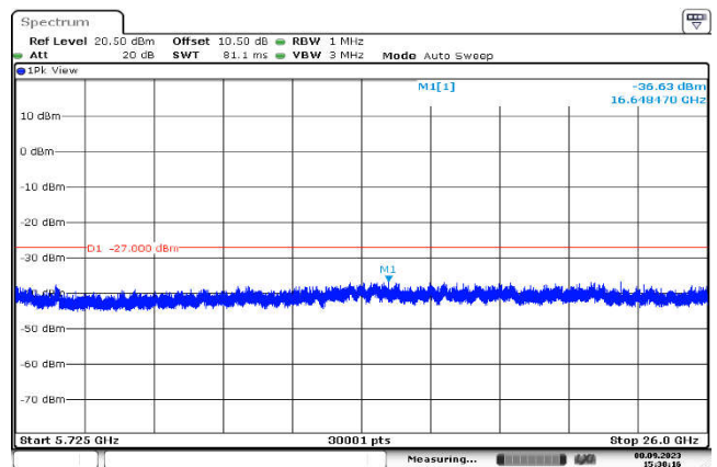
U-NII-2c,802.11ac(20MHz),5700MHz ,Ant1,Plot 3,5725MHz~26000MHz
