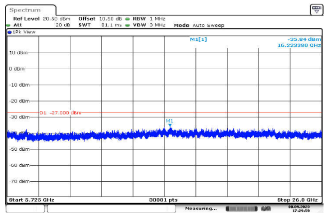
U-NII-2c,802.11ac(80MHz),5530MHz ,Ant1,Plot 3,5725MHz~26000MHz
