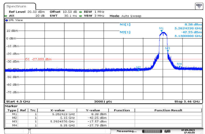
U-NII-2a,802.11ac(40MHz),5270MHz ,Ant1,Plot 1,Band Edge
