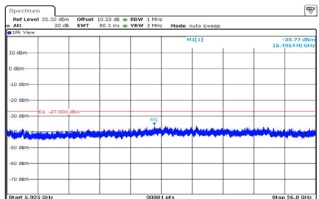
U-NII-3,802.11n(40MHz),5755MHz ,Ant1,Plot 3,5925MHz~26000MHz
