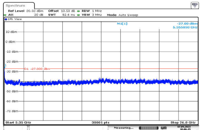
U-NII-2a,802.11ac(80MHz),5290MHz ,Ant1,Plot 3,5350MHz~26000MHz
