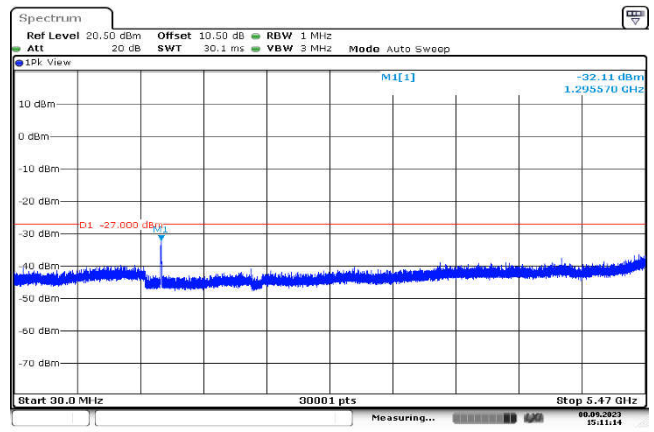
U-NII-2c,802.11a(20MHz),5500MHz ,Ant1,Plot 2,30MHz~5470MHz
