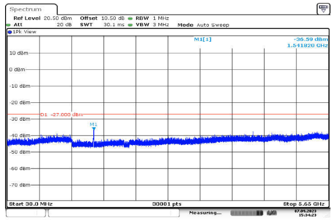
U-NII-3,802.11ac(20MHz),5745MHz ,Ant1,Plot 2,30MHz~5650MHz
