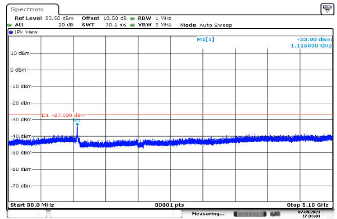
U-NII-2a,802.11ac(20MHz),5320MHz ,Ant1,Plot 2,30MHz~5150MHz
