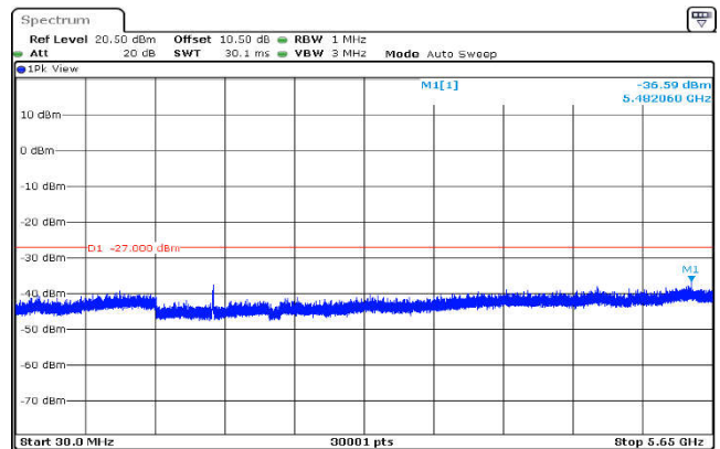
U-NII-3,802.11n(20MHz),5825MHz ,Ant1,Plot 2,30MHz~5650MHz
