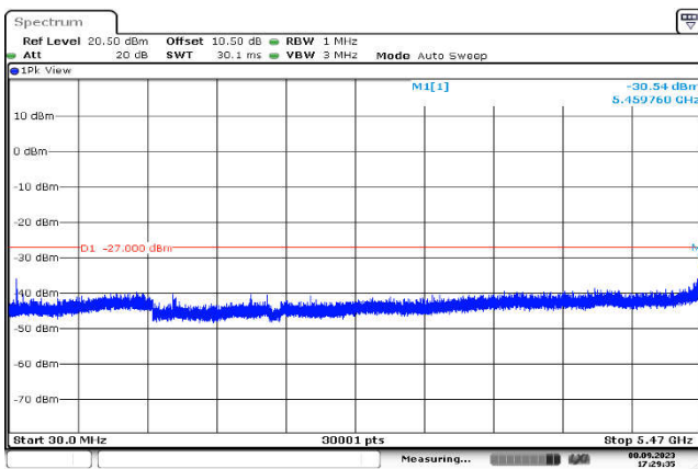
U-NII-2c,802.11ac(80MHz),5530MHz ,Ant1,Plot 2,30MHz~5470MHz
