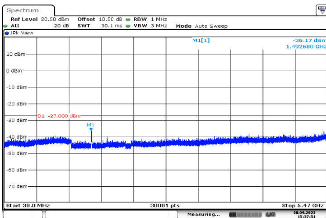
U-NII-2c,802.11ac(20MHz),5700MHz ,Ant1,Plot 2,30MHz~5470MHz
