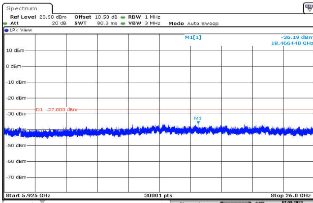
U-NII-3,802.11ac(20MHz),5825MHz ,Ant1,Plot 3,5925MHz~26000MHz
