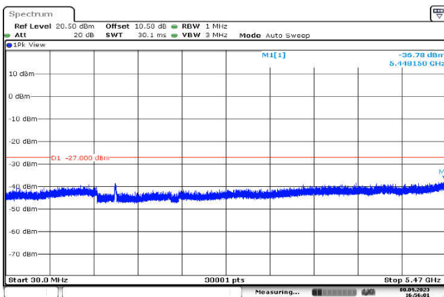
U-NII-2c,802.11ac(40MHz),5590MHz ,Ant1,Plot 2,30MHz~5470MHz
