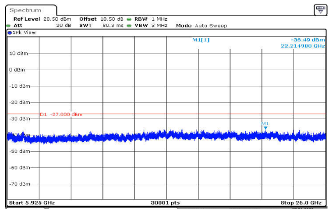
U-NII-3,802.11ac(40MHz),5755MHz ,Ant1,Plot 3,5925MHz~26000MHz
