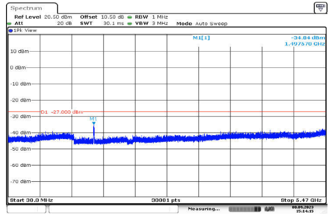
U-NII-2c,802.11a(20MHz),5700MHz ,Ant1,Plot 2,30MHz~5470MHz
