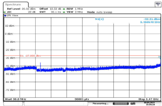
U-NII-2c,802.11n(20MHz),5500MHz ,Ant1,Plot 2,30MHz~5470MHz
