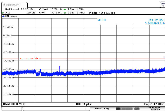
U-NII-2c,802.11n(40MHz),5510MHz ,Ant1,Plot 2,30MHz~5470MHz
