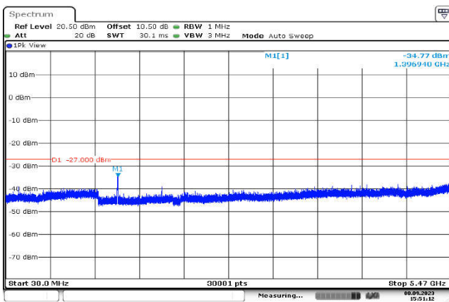
U-NII-2c,802.11n(20MHz),5600MHz ,Ant1,Plot 2,30MHz~5470MHz
