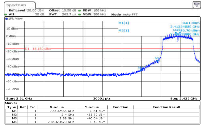
802.11n(HT20),2412MHz,Ant0,Plot 2,Band Edge
