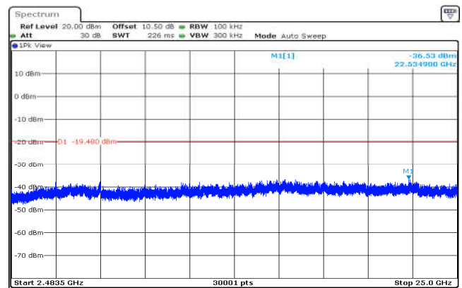
802.11n(HT40),2452MHz,Ant0,Plot 4,2483.5MHz~25000MHz
