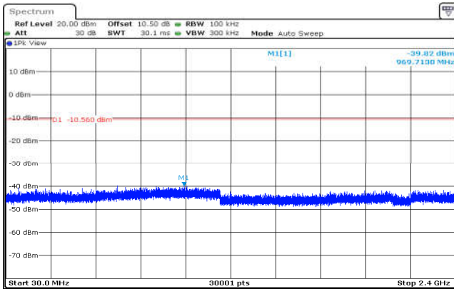
802.11b,2437MHz,Ant0,Plot 3,30MHz~240 0MHz
