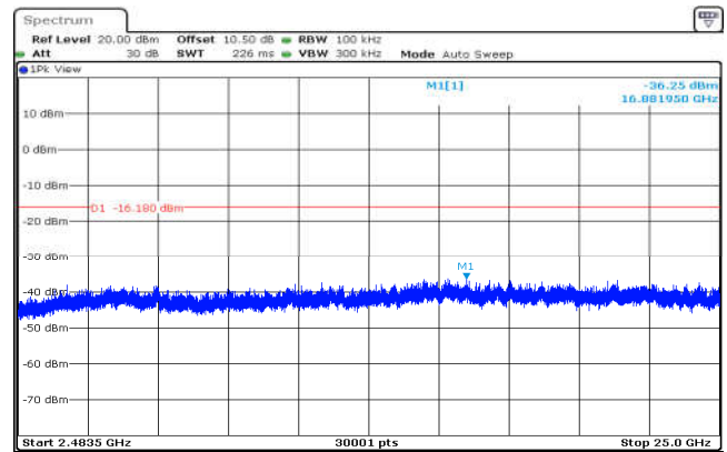
802.11n(HT20),2437MHz,Ant0,Plot 4,2483.5MHz~25000MHz
