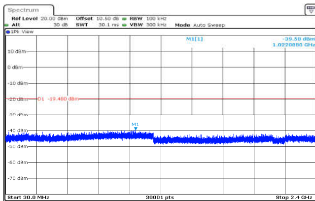
802.11n(HT40),2452MHz,Ant0,Plot 3,30MHz~2400MHz
