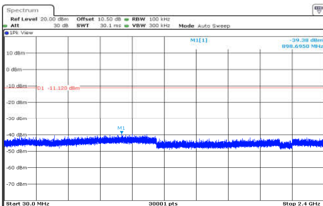
802.11b,2462MHz,Ant0,Plot 3,30MHz~240 0MHz
