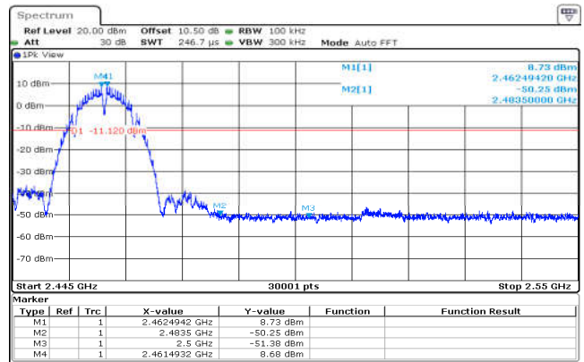
802.11b,2462MHz,Ant0,Plot 2,Band Edge
