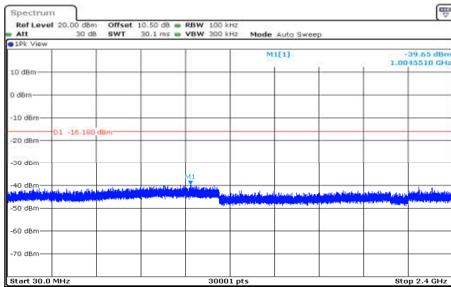
802.11n(HT20),2437MHz,Ant0,Plot 3,30MHz~2400MHz
