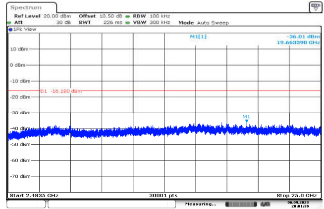
802.11n(HT20),2412MHz,Ant0,Plot 4,2483.5MHz~25000MHz
