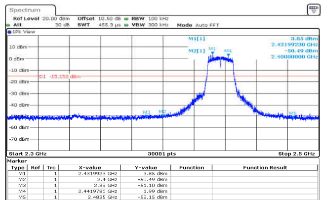
802.11g,2437MHz,Ant0,Plot 2,Band Edge
