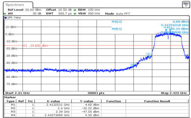
802.11g,2412MHz,Ant0,Plot 2,Band Edge
