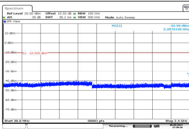
802.11b,2412MHz,Ant0,Plot 3,30MHz~2400MHz
