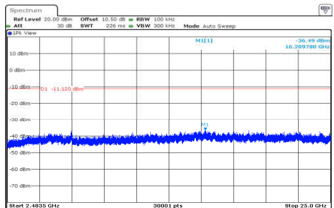
802.11b,2462MHz,Ant0,Plot 4,2483.5MHz ~25000MHz
