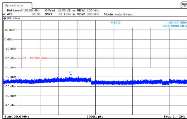
802.11n(HT40),2437MHz,Ant0,Plot 3,30MHz~2400MHz
