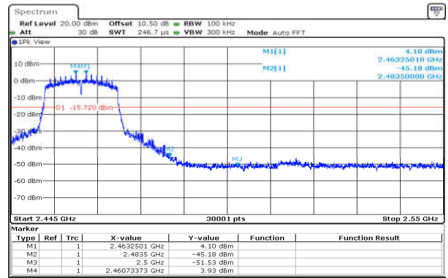
802.11n(HT20),2462MHz,Ant0,Plot 2,Band Edge
