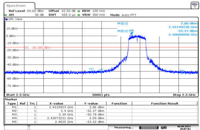
802.11n(HT20),2437MHz,Ant0,Plot 2,Band Edge
