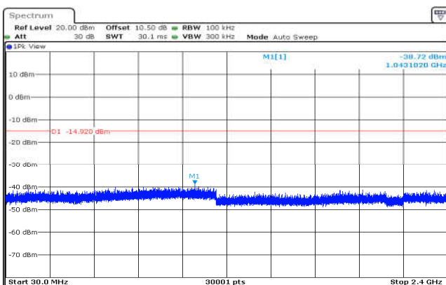
802.11g,2462MHz,Ant0,Plot 3,30MHz~240 0MHz
