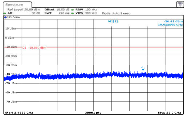
802.11b,2437MHz,Ant0,Plot 4,2483.5MHz ~25000MHz
