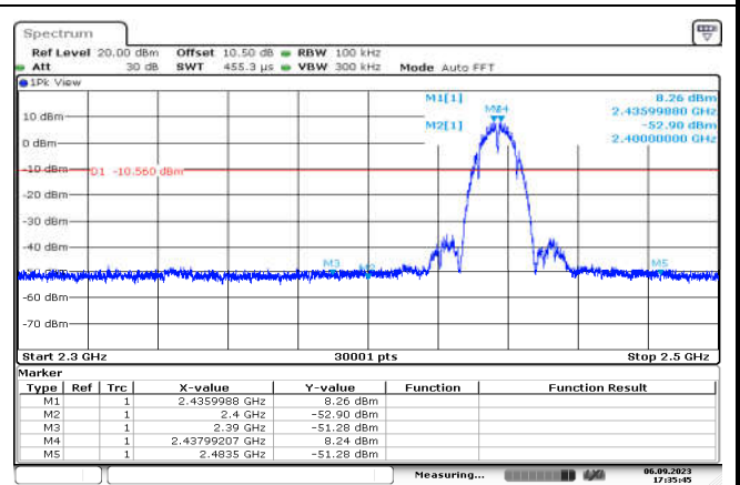
802.11b,2437MHz,Ant0,Plot 2,Band Edge
