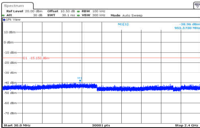
802.11g,2437MHz,Ant0,Plot 3,30MHz~240 0MHz
