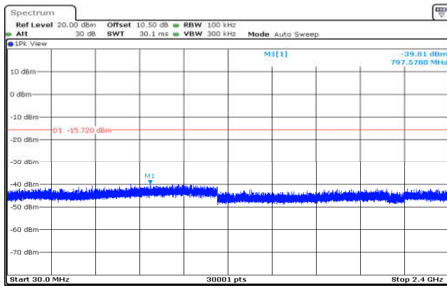
802.11n(HT20),2462MHz,Ant0,Plot 3,30MHz~2400MHz
