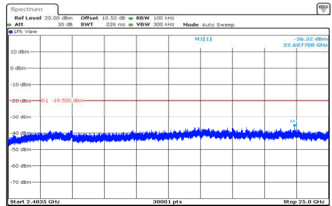
802.11n(HT40),2437MHz,Ant0,Plot 4,2483.5MHz~25000MHz
