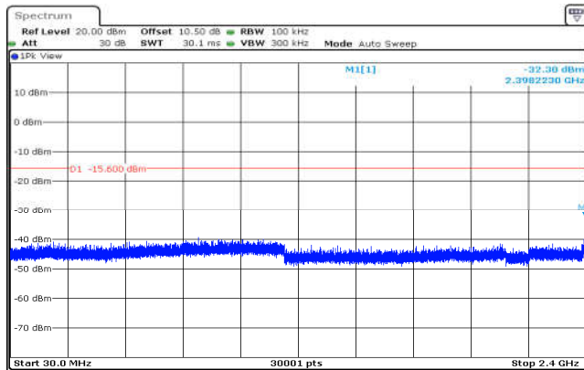
802.11g,2412MHz,Ant0,Plot 3,30MHz~240 0MHz
