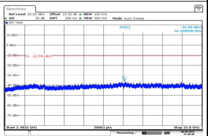
802.11b,2412MHz,Ant0,Plot 4,2483.5MHz~25000MHz
