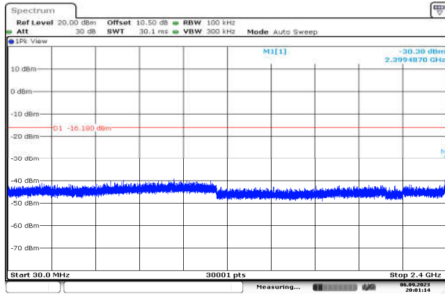
802.11n(HT20),2412MHz,Ant0,Plot 3,30MHz~2400MHz
