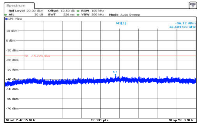
802.11n(HT20),2462MHz,Ant0,Plot 4,2483.5MHz~25000MHz
