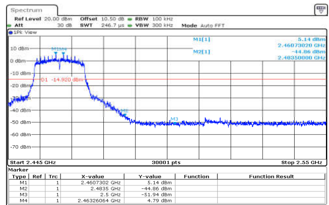
802.11g,2462MHz,Ant0,Plot 2,Band Edge
