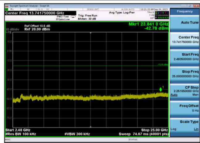
,Plot 4,2483.5MHz~25000MHz-802.11n(HT20),2462MHz,Ant0
