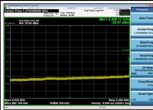
,Plot 3,30MHz~2400MHz-802.11n(HT20),2462MHz,Ant0
