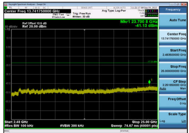
,Plot 4,2483.5MHz~25000MHz-802.11n(HT40),2452MHz,Ant0
