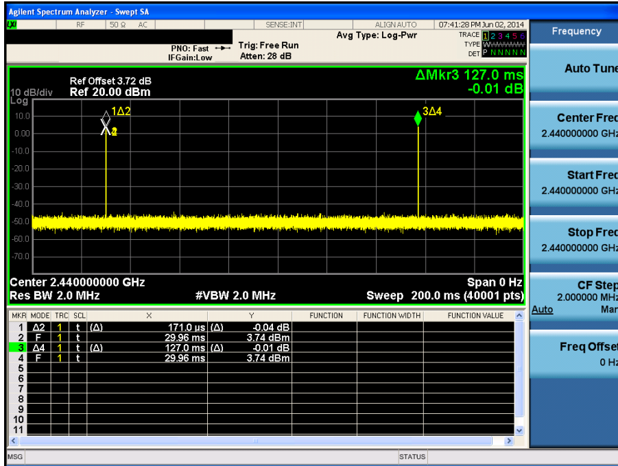
1 Pulse on time : 0.171ms
