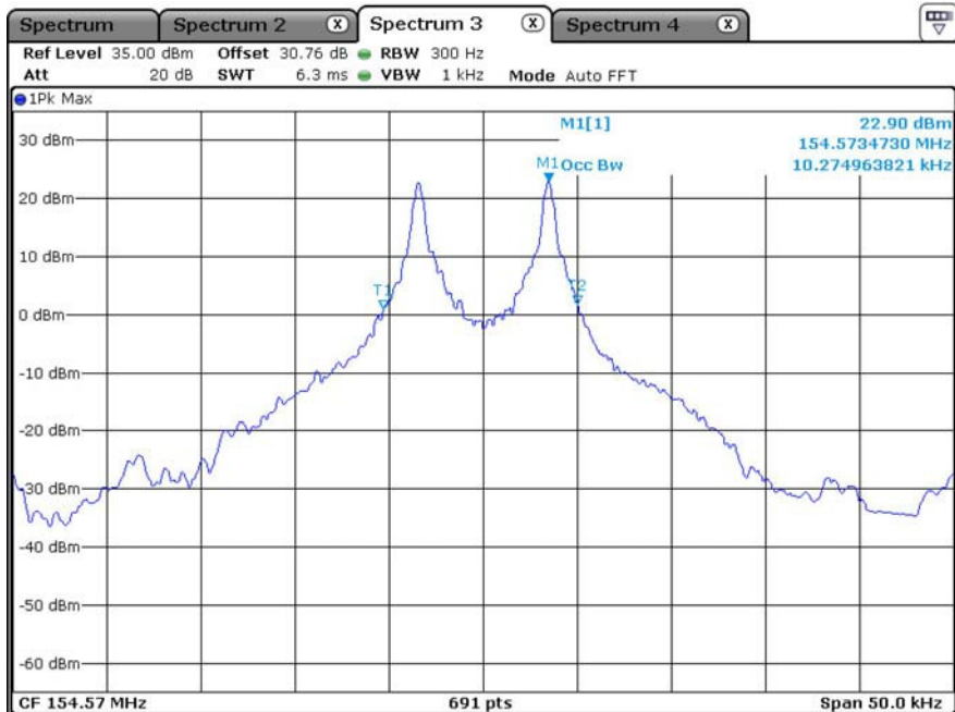
(Ch4 : 154.570 MHz)
