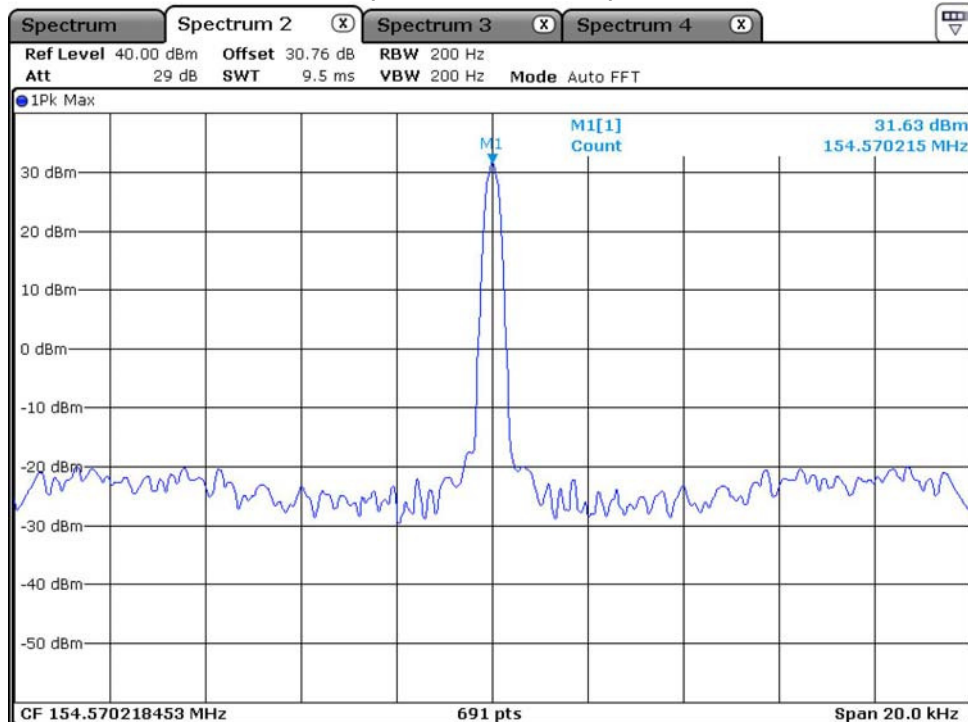
(Ch4 : 154.570 MHz)
