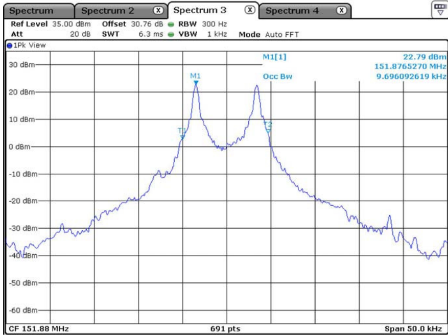
(Ch2 : 151.880 MHz)
