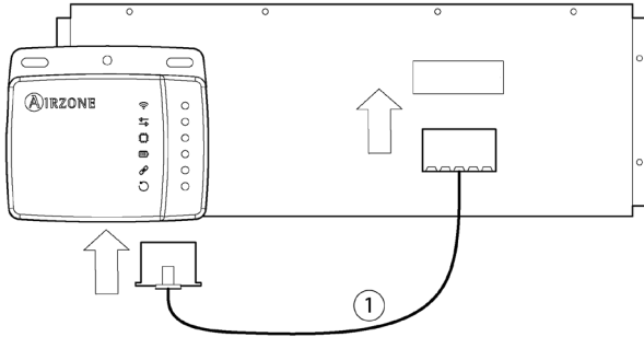
Anschlusschema
