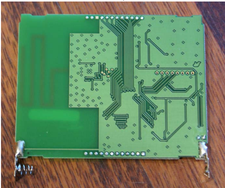
PCB Top
