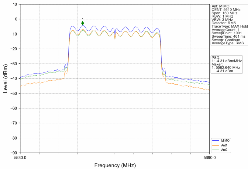
802.11ac(VHT80)_HCH_5610MHz_MIMO_NTNV
