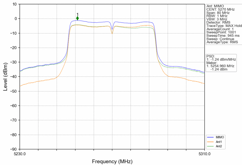
802.11n(HT40)_LCH_5270MHz_MIMO_NTNV
