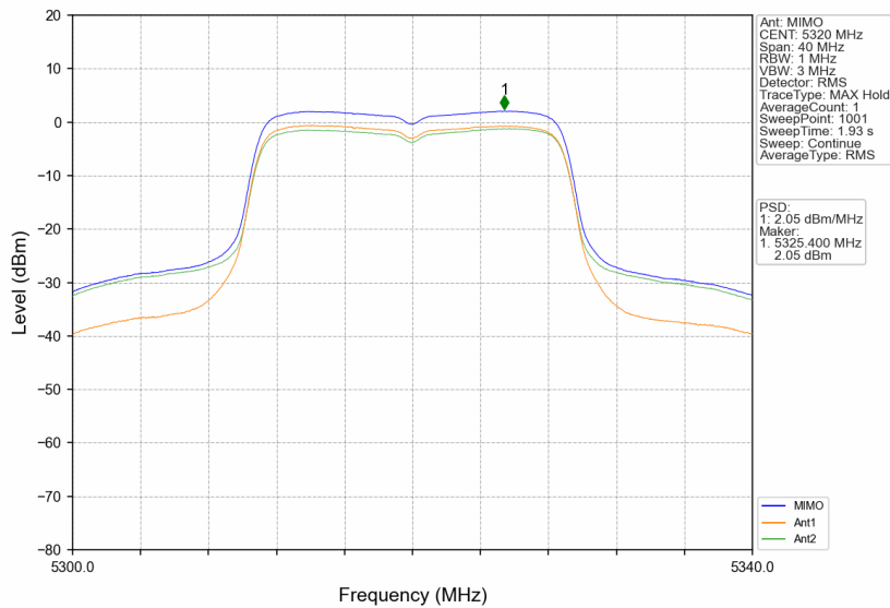
802.11n(HT20)_HCH_5320MHz_MIMO_NTNV
