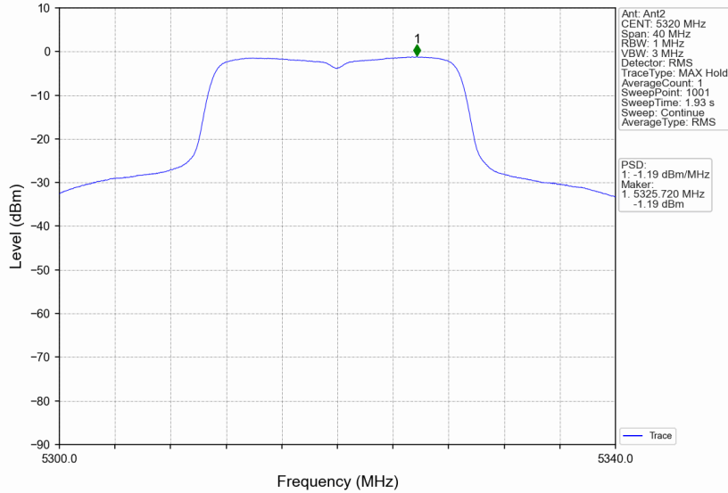
802.11n(HT20)_HCH_5320MHz_MIMO_NTNV
