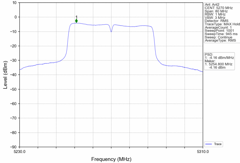
802.11n(HT40)_LCH_5270MHz_MIMO_NTNV
