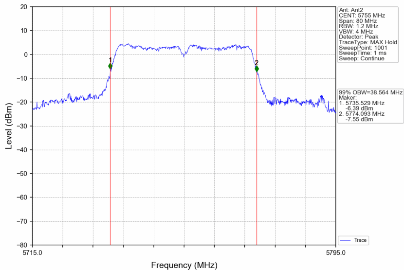
802.11ac(VHT40)_LCH_5755MHz_Ant2_NTNV
