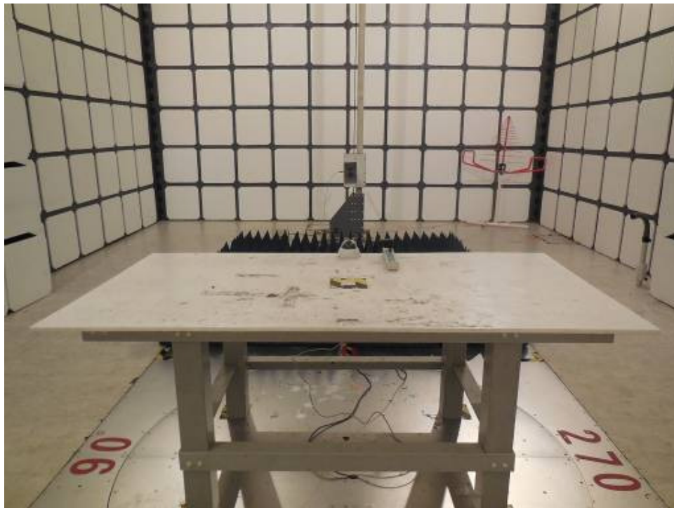
30MHz~1000MHz
