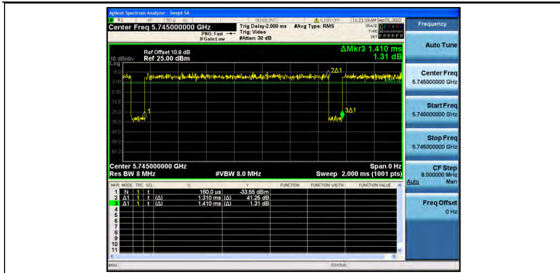
11AC20MIMO_Ant2_5745
