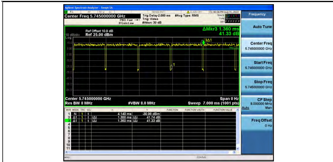
11N20MIMO_Ant2_5745
