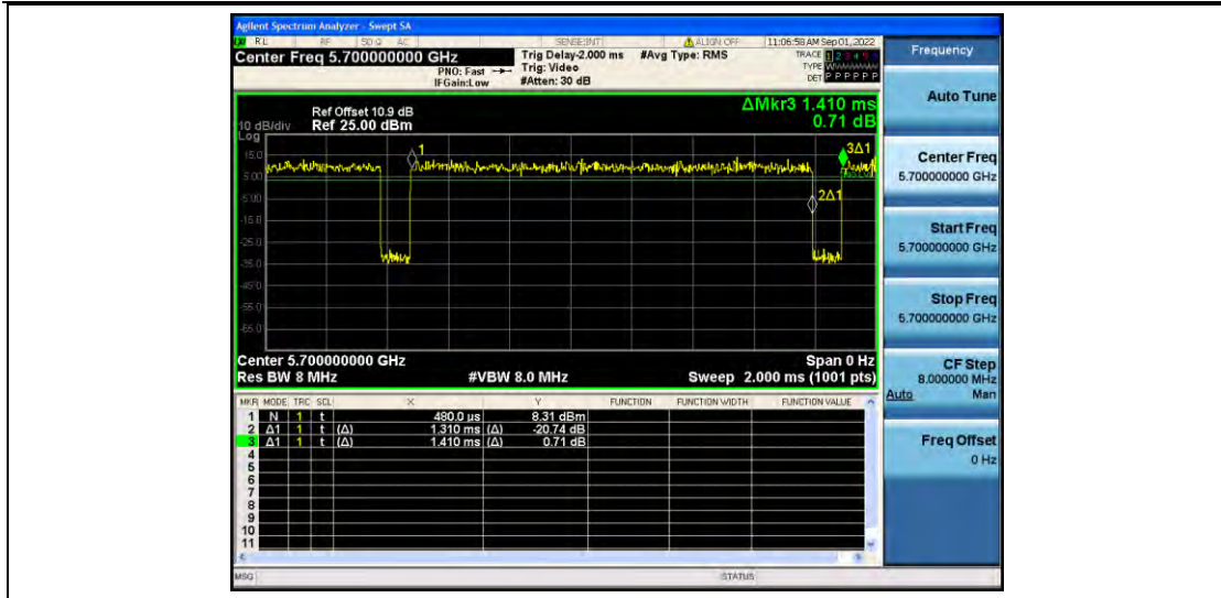
11AC20MIMO_Ant2_5700
