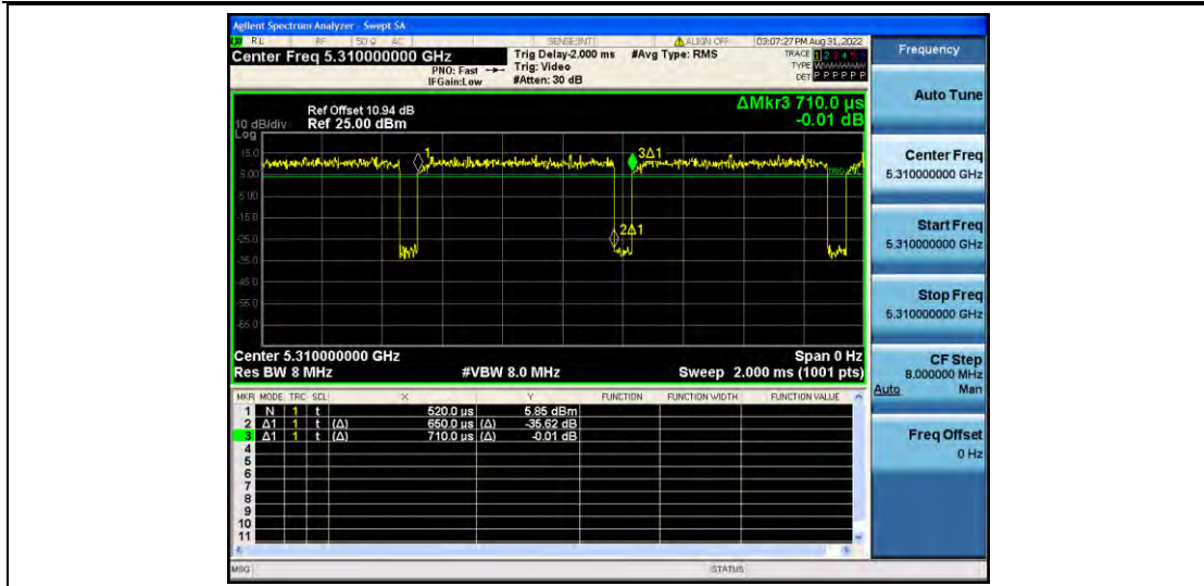
11N40MIMO_Ant2_5310
