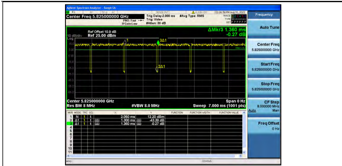
11N20MIMO_Ant2_5825
