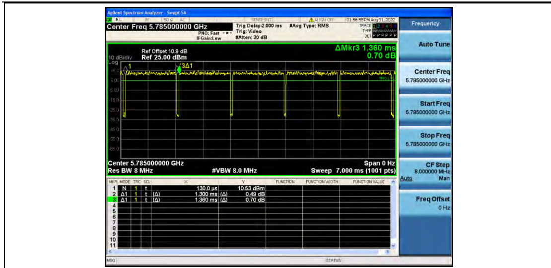
11N20MIMO_Ant2_5785
