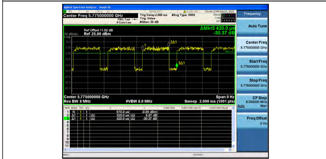
11AC80MIMO_Ant2_5775
