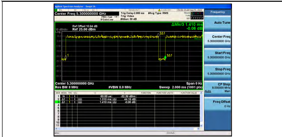
11AC20MIMO_Ant2_5300
