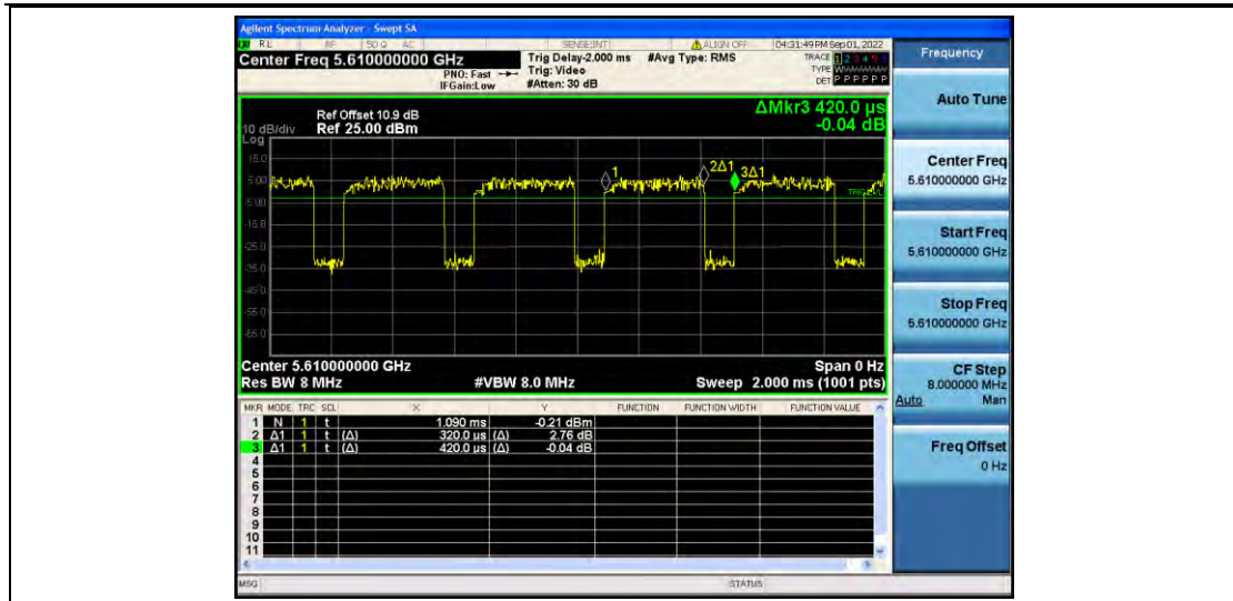
11AC80MIMO_Ant2_5610
