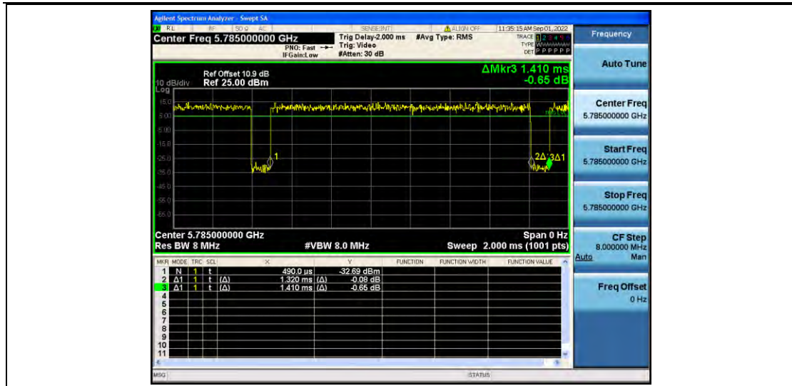
11AC20MIMO_Ant2_5785
