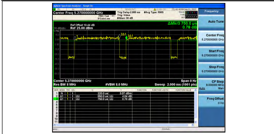
11AC40MIMO_Ant2_5270
