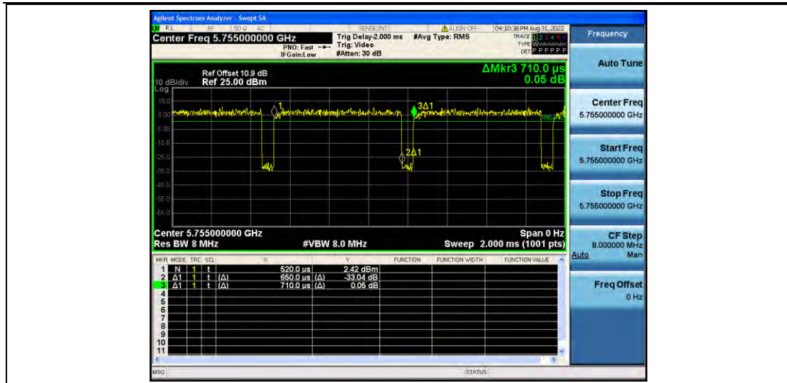
11N40MIMO_Ant2_5755
