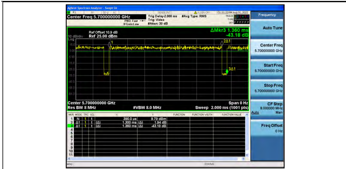
11N20MIMO_Ant2_5700
