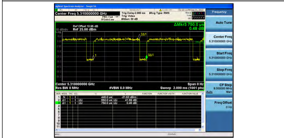
11AC40MIMO_Ant1_5310
