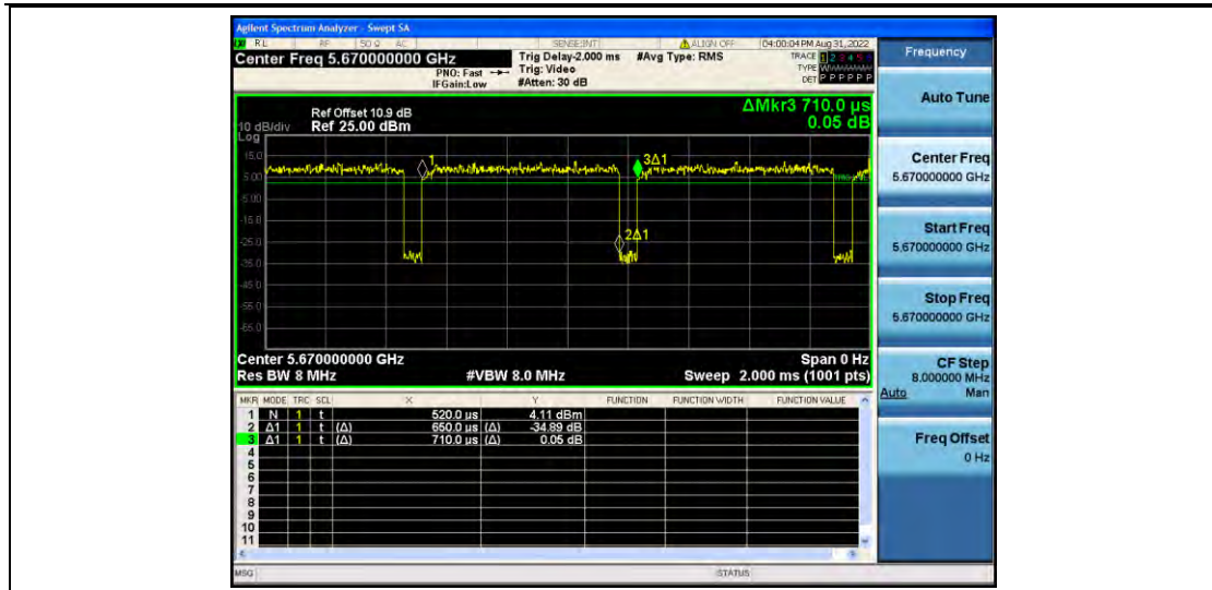
11N40MIMO_Ant2_5670
