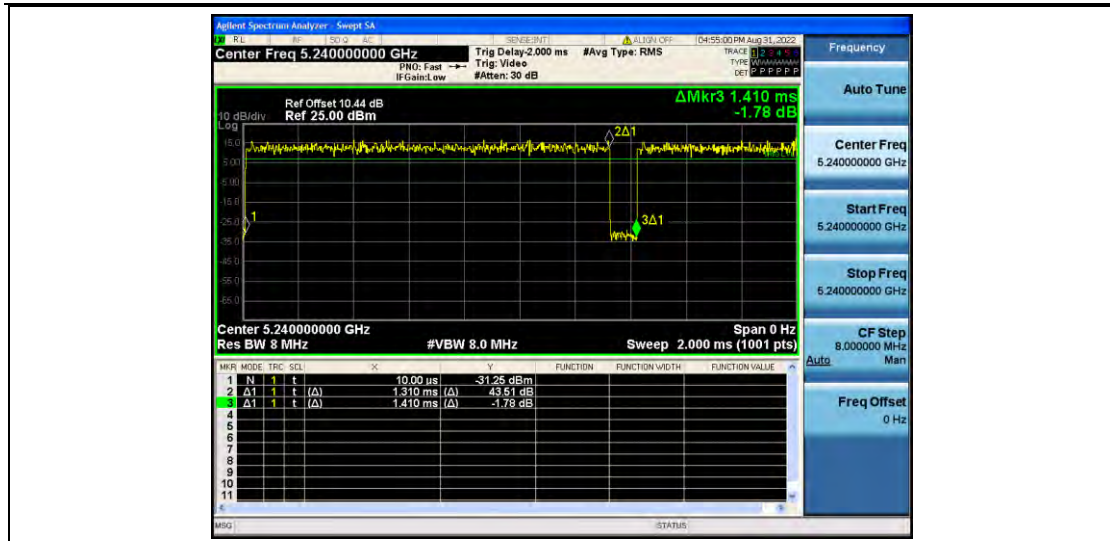
11AC20MIMO_Ant2_5240
