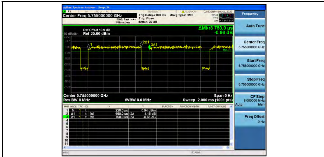
11AC40MIMO_Ant2_5755
