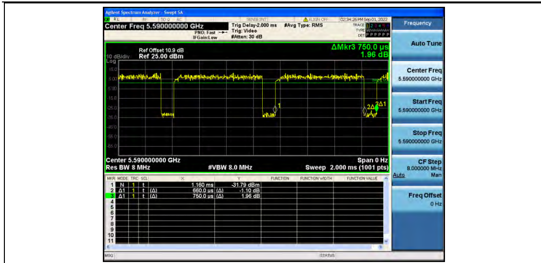
11AC40MIMO_Ant2_5590
