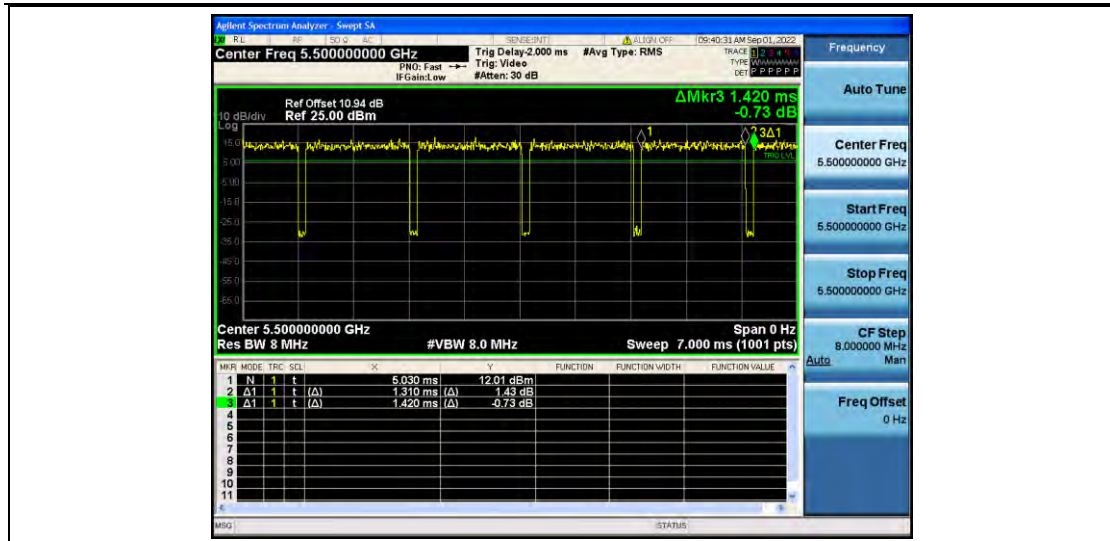
11AC20MIMO_Ant2_5500
