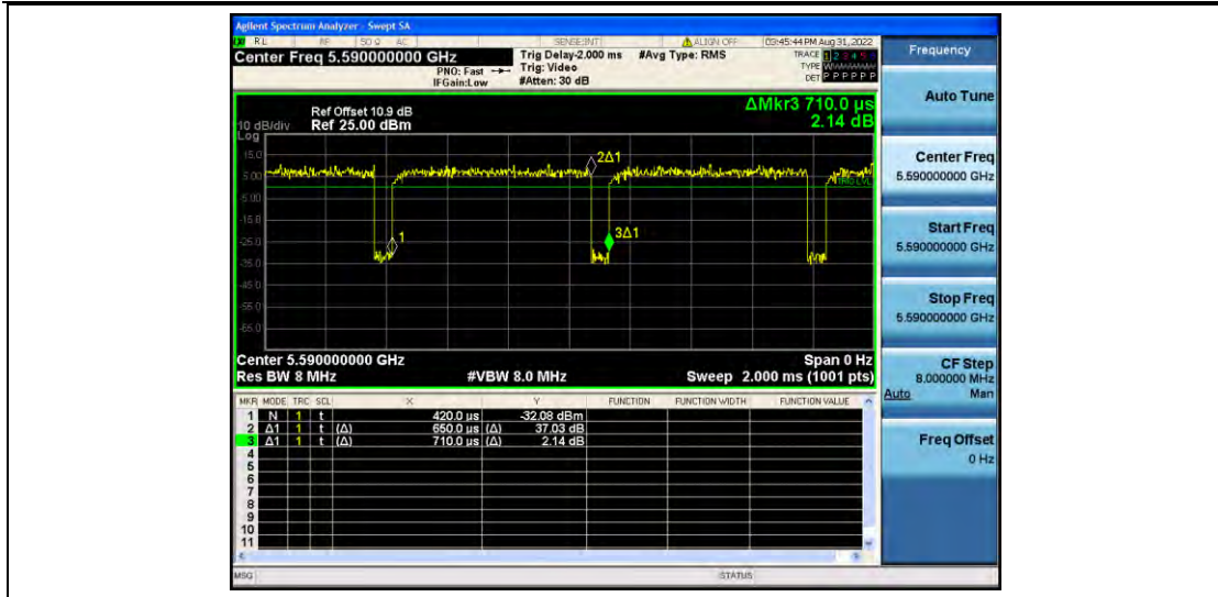
11N40MIMO_Ant2_5590
