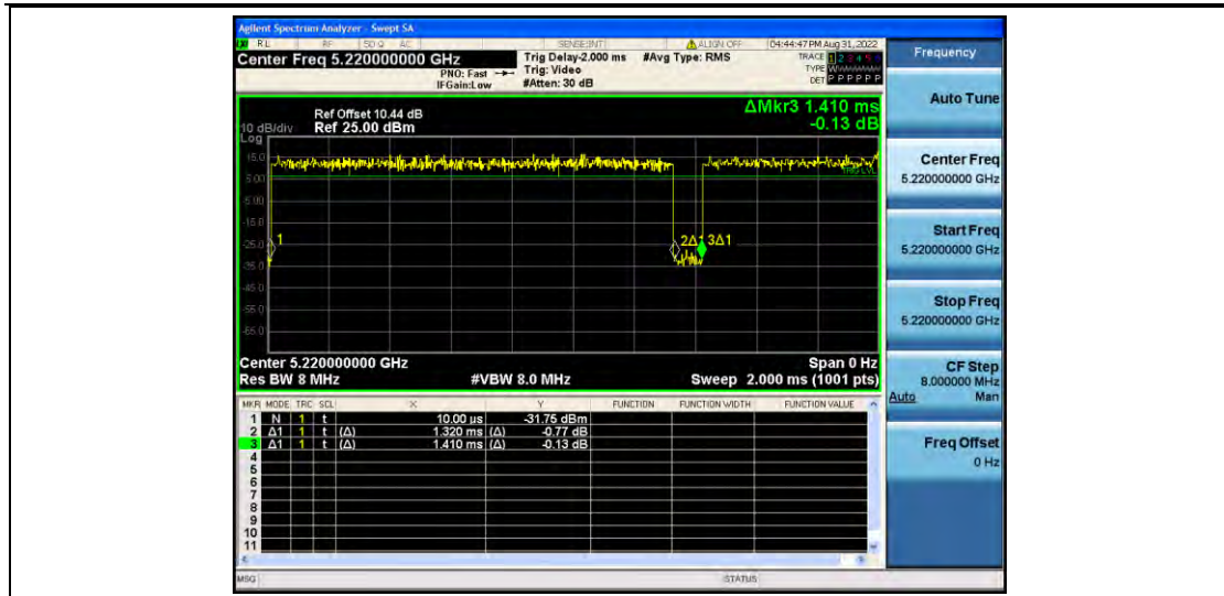
11AC20MIMO_Ant2_5220
