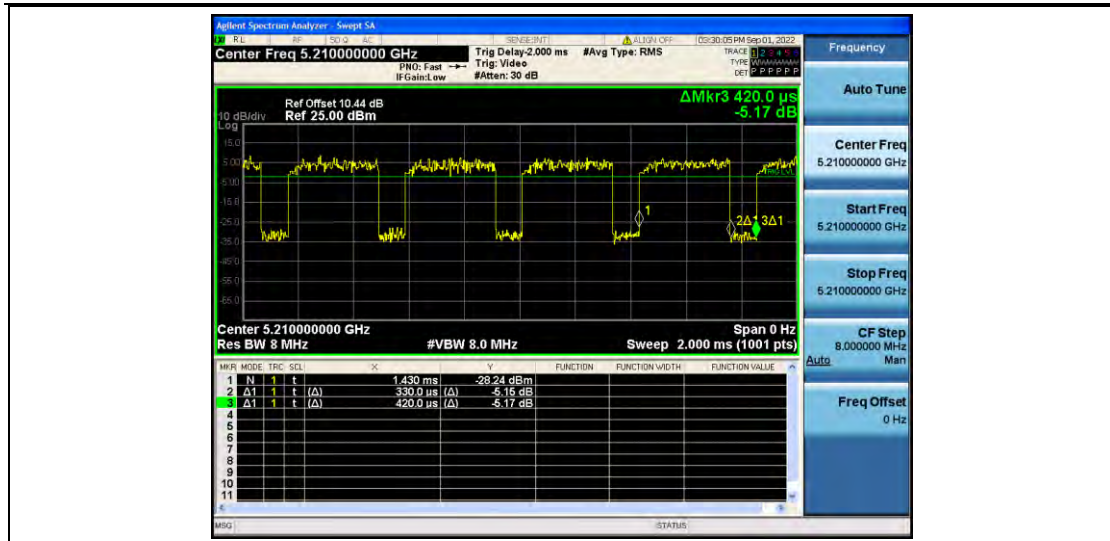
11AC80MIMO_Ant2_5210
