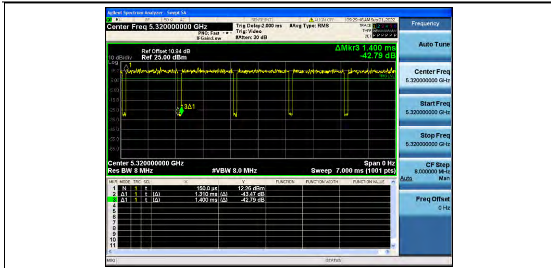
11AC20MIMO_Ant2_5320
