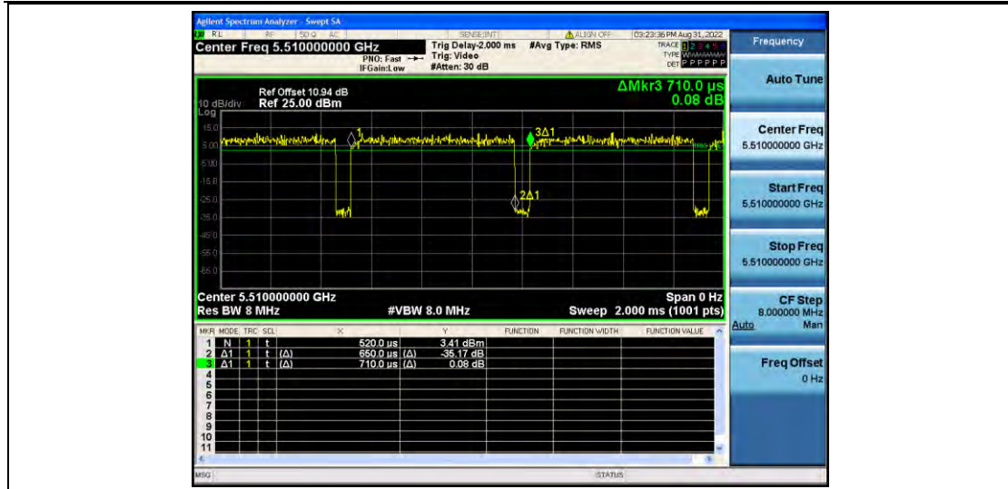
11N40MIMO_Ant2_5510
