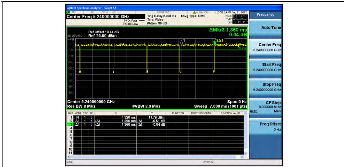
11N20MIMO_Ant2_5240
