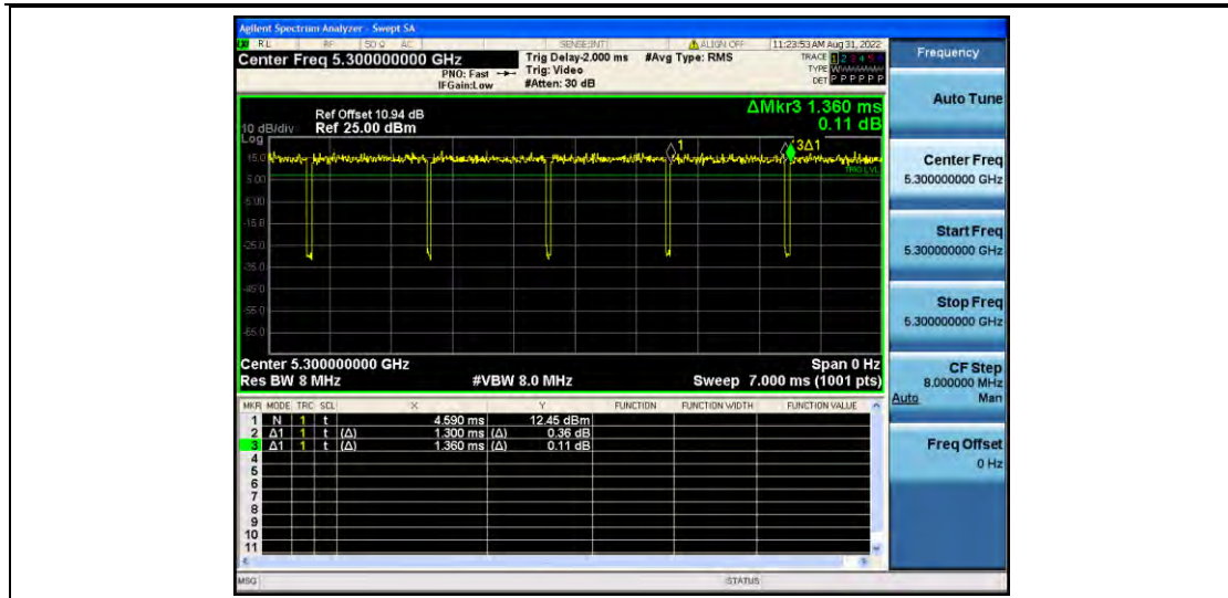
11N20MIMO_Ant2_5300
