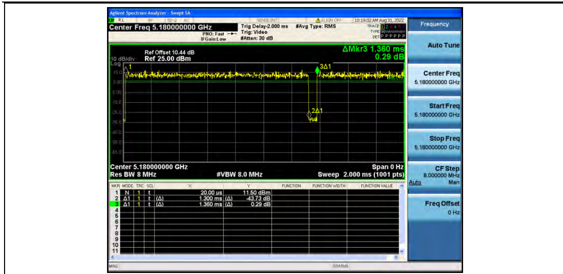
11N20MIMO_Ant2_5180
