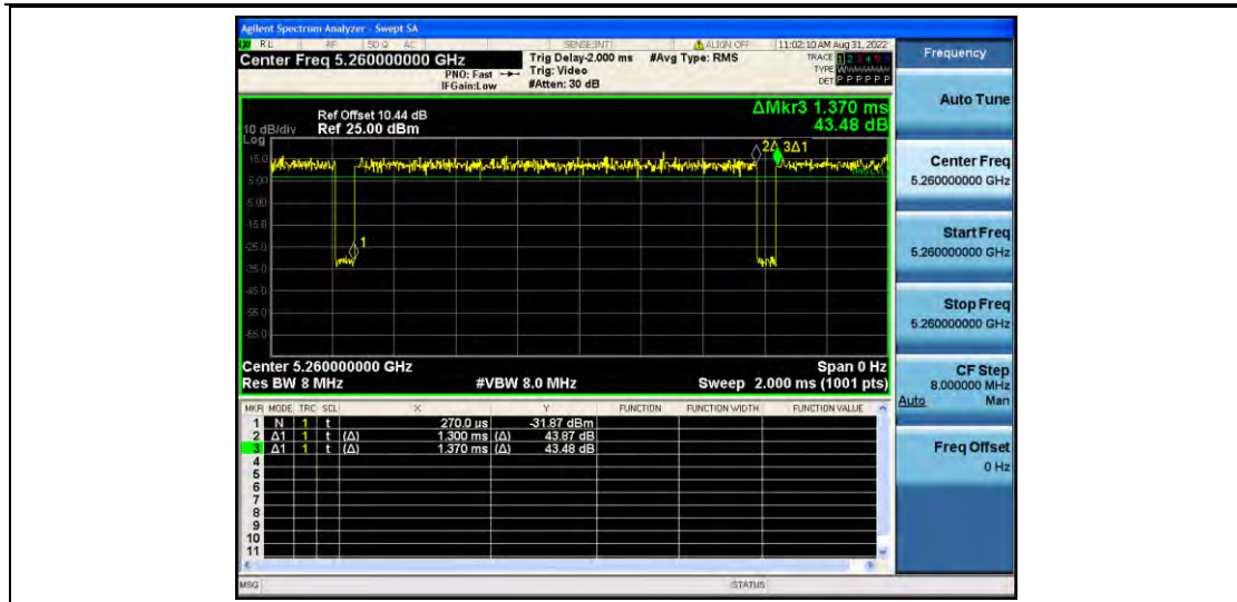
11N20MIMO_Ant2_5260
