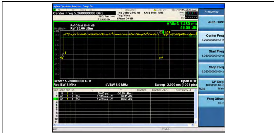
11A_Ant2_5260
