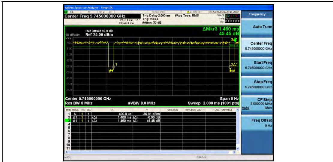
11A_Ant2_5745
