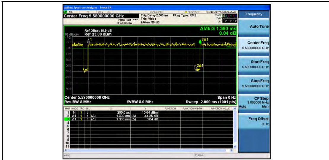
11N20MIMO_Ant2_5580
