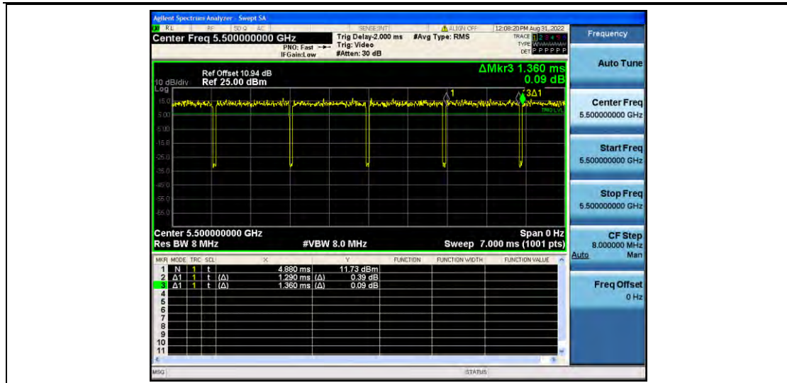
11N20MIMO_Ant2_5500
