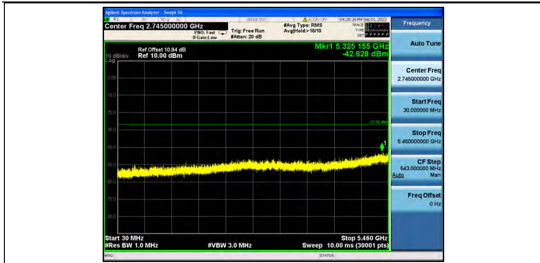
11AC80MIMO_Ant1_5530_5735~4000
