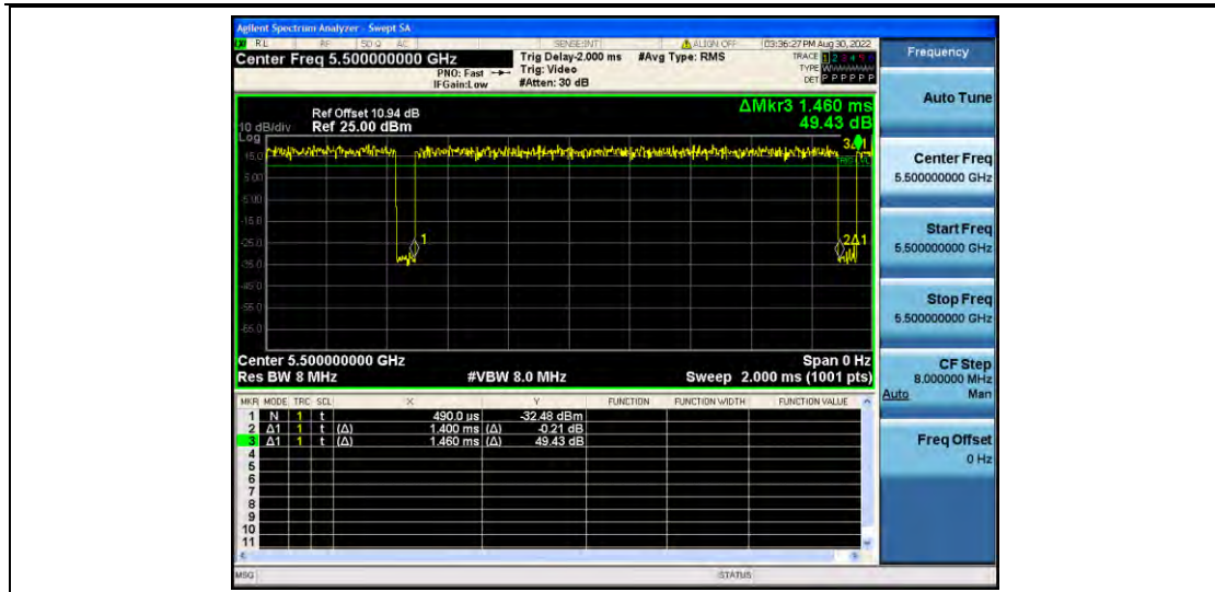
11A_Ant2_5500
