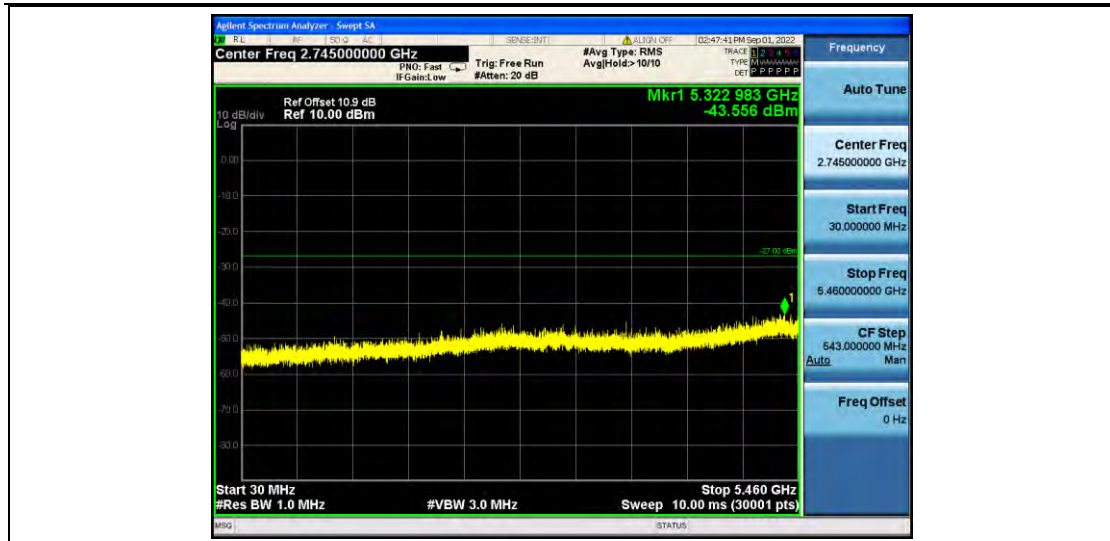
11AC40MIMO_Ant1_5670_5735~40000
