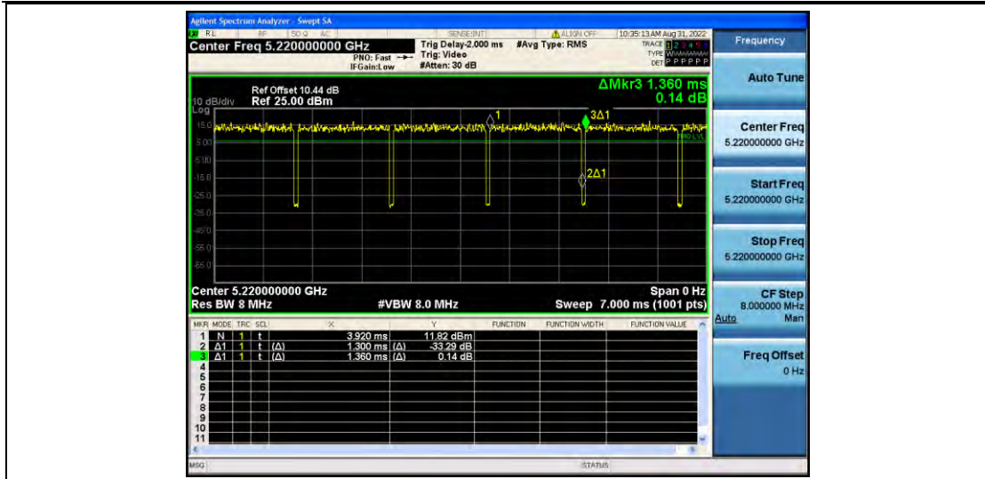
11N20MIMO_Ant2_5220
