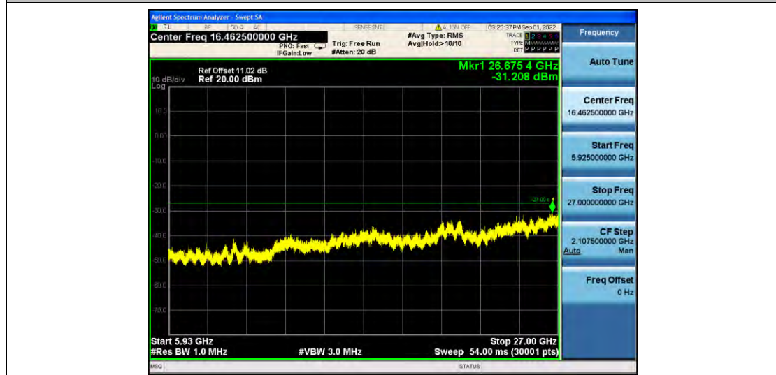
11AC80MIMO_Ant1_5210_30~5140
