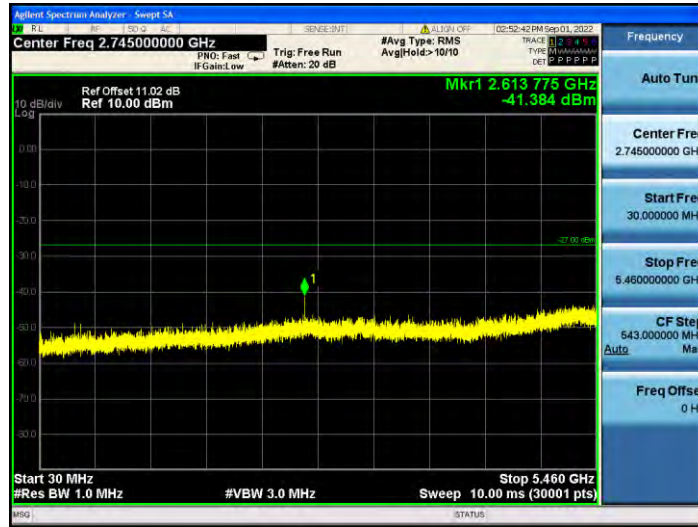
11AC40MIMO_Ant2_5670_5735~4000
