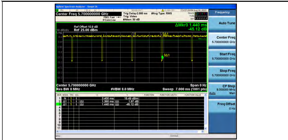
11A_Ant2_5700
