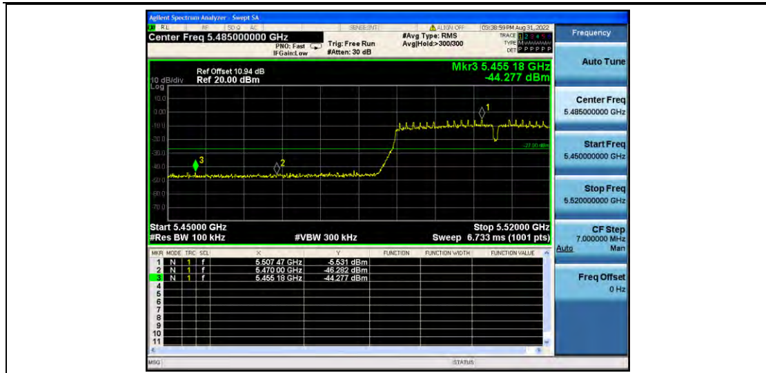
11N40MIMO_Ant2_Low_5510
