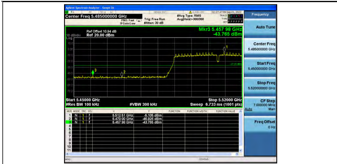
11AC40MIMO_Ant2_Low_5510
