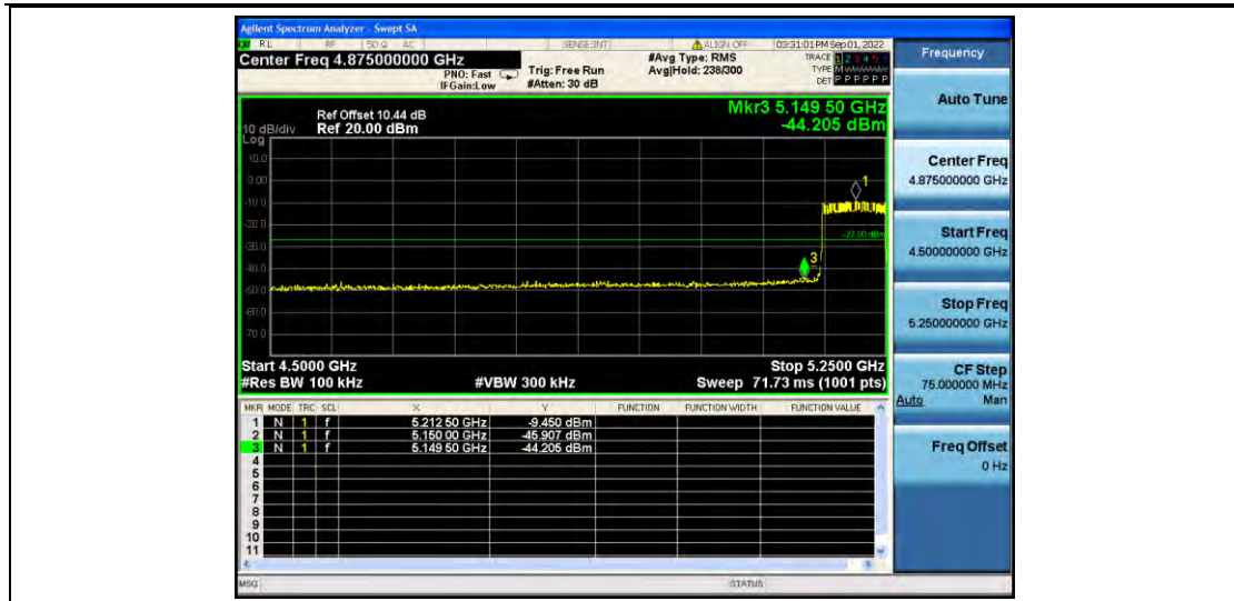
11AC80MIMO_Ant2_Low_5210
