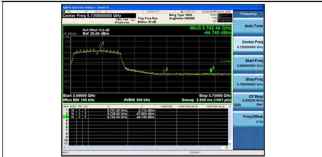
11N20MIMO_Ant2_High_5700
