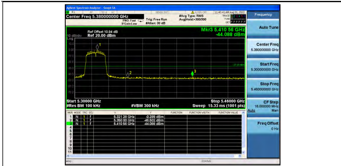
11N20MIMO_Ant2_High_5320
