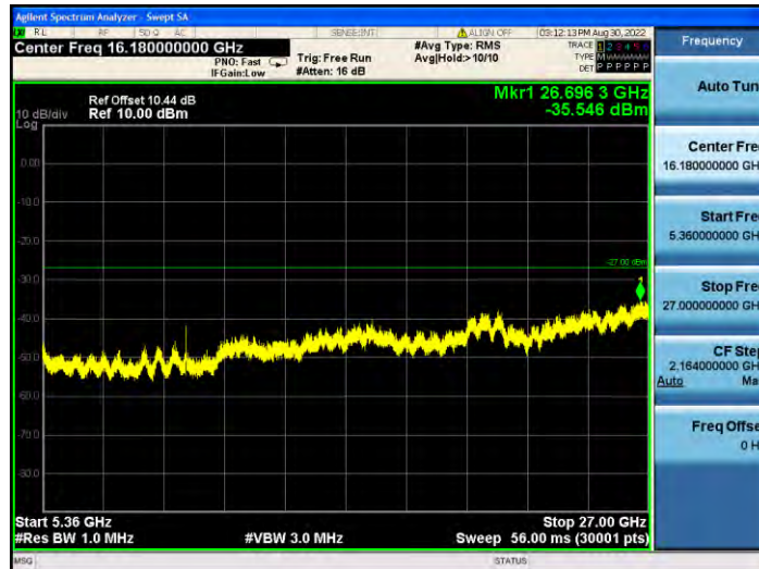
11A_Ant2_5240_30~5140
