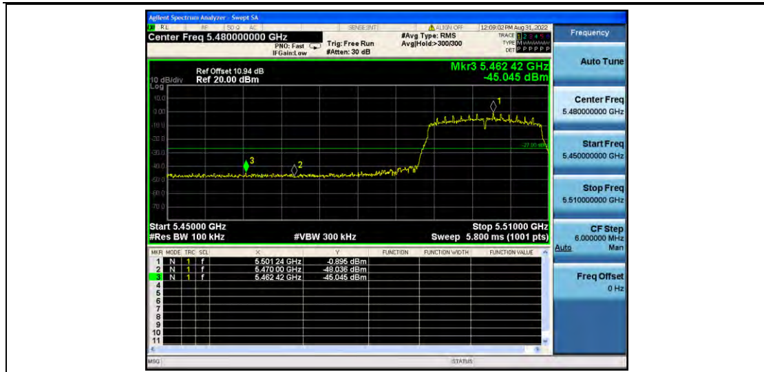
11N20MIMO_Ant2_Low_5500
