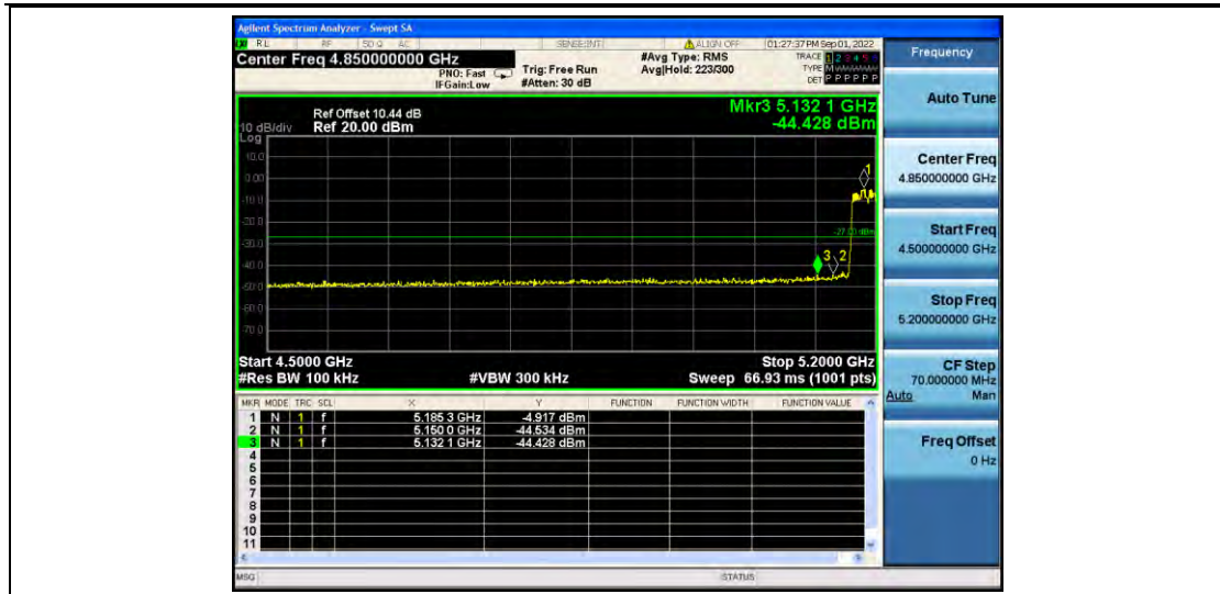
11AC40MIMO_Ant2_Low_5190
