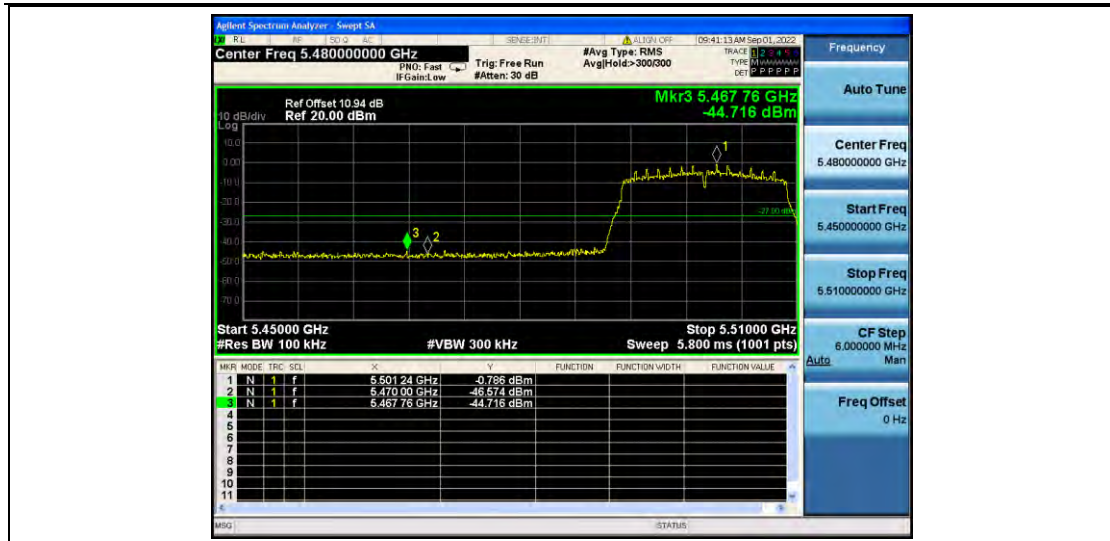
11AC20MIMO_Ant2_Low_5500
