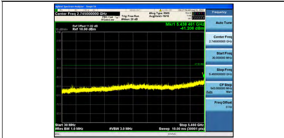
11A_Ant2_5580_5735~40000
