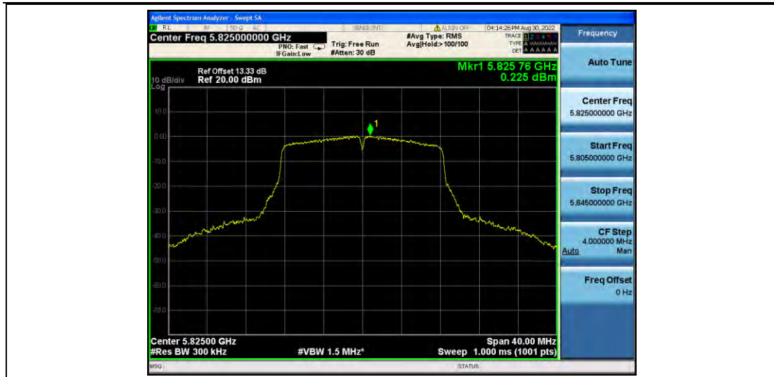
11A_Ant2_5825
