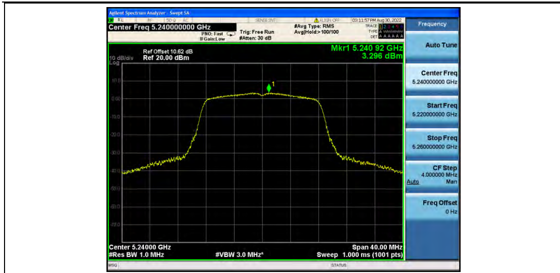
11A_Ant2_5240
