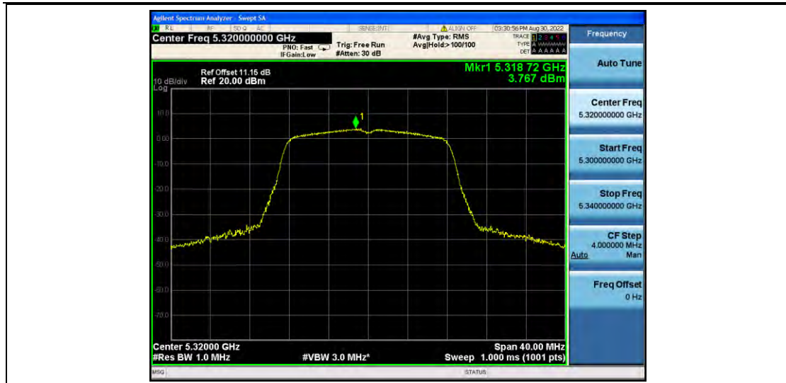
11A_Ant2_5320
