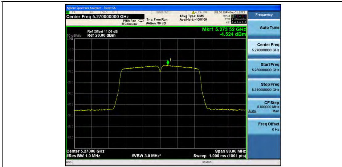
11AC40MIMO_Ant2_5270
