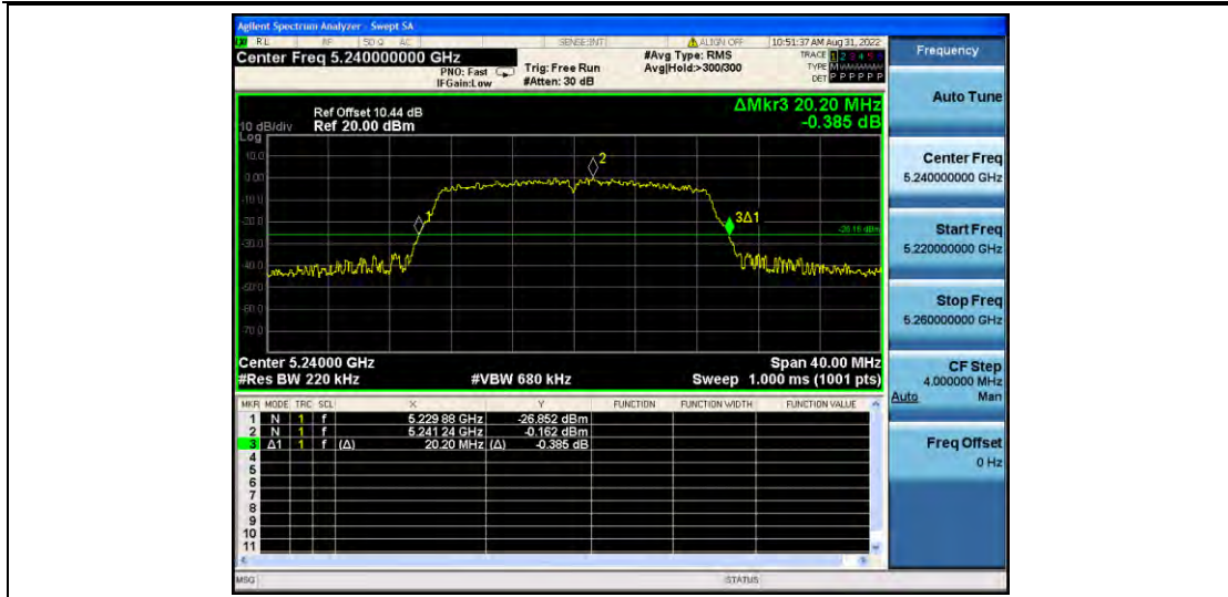
11N20MIMO_Ant2_5240
