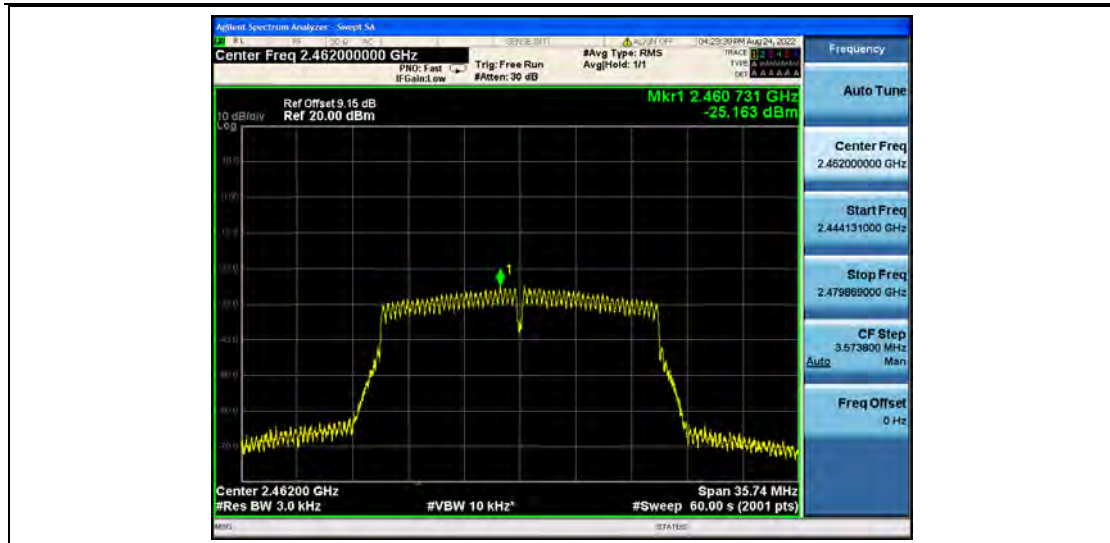
11N20MIMO_Ant2_2462
