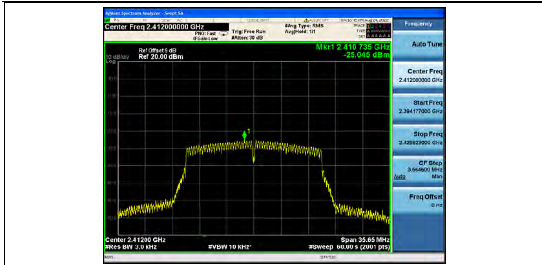
11N20MIMO_Ant2_2412
