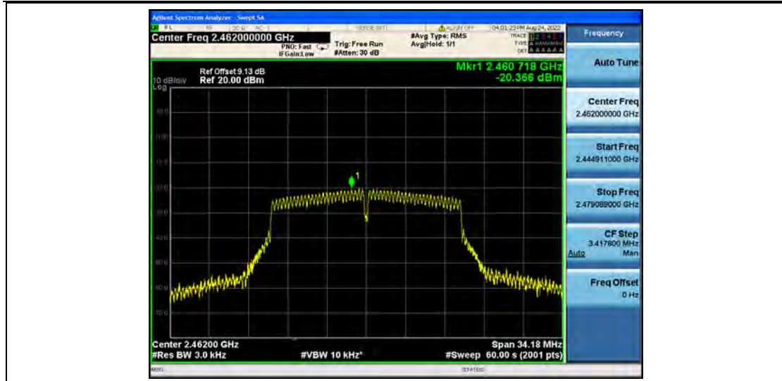
11G_Ant2_2462
