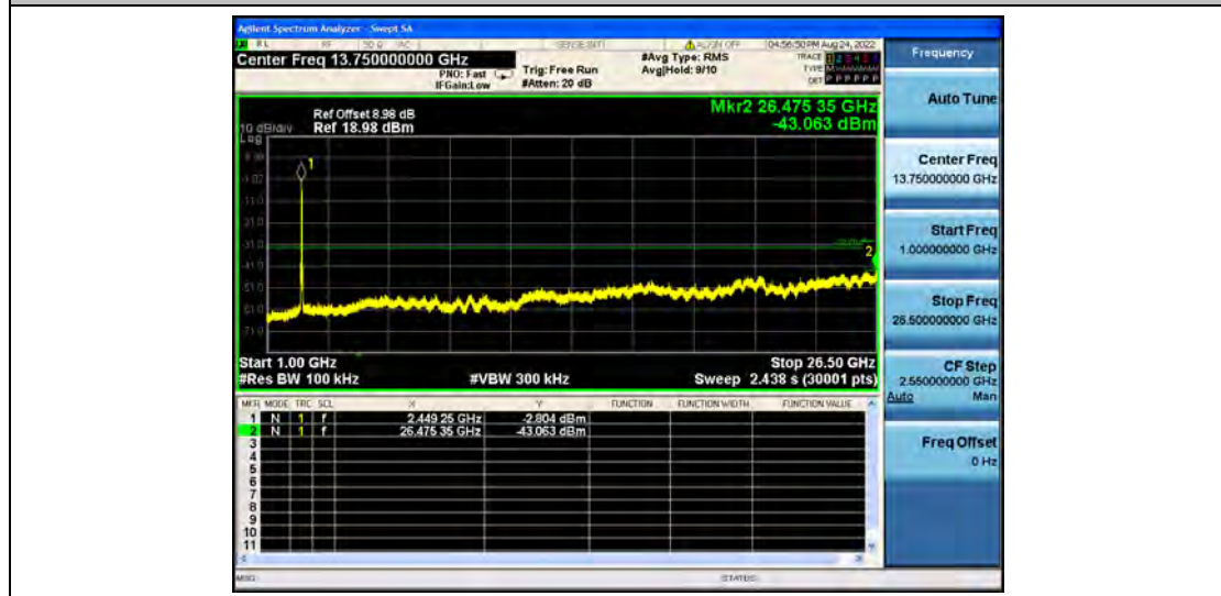
11N40MIMO_Ant2_2452_1000~26500
