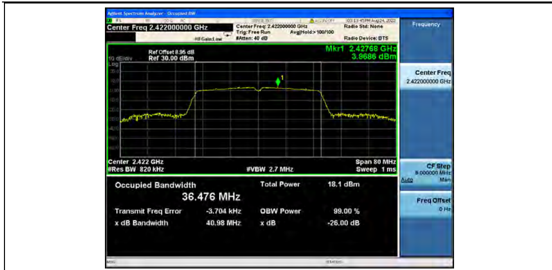
11N40MIMO_Ant2_2422
