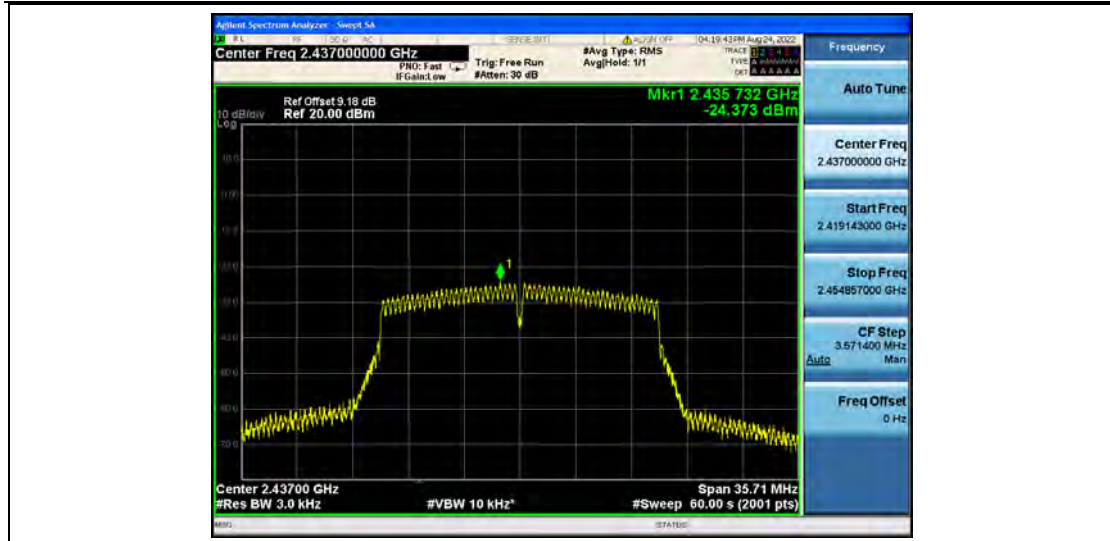
11N20MIMO_Ant2_2437
