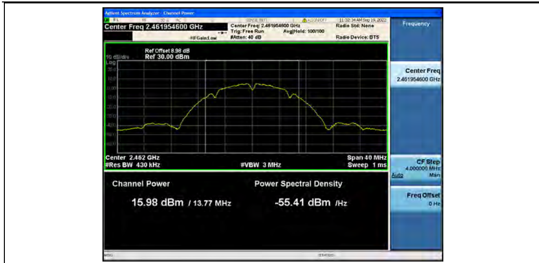
11B_Ant2_2462
