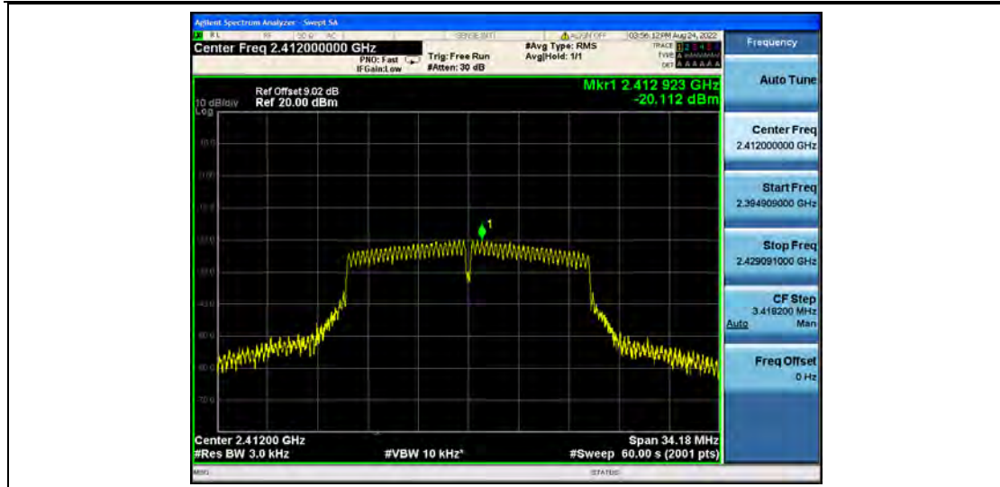
11G_Ant2_2412
