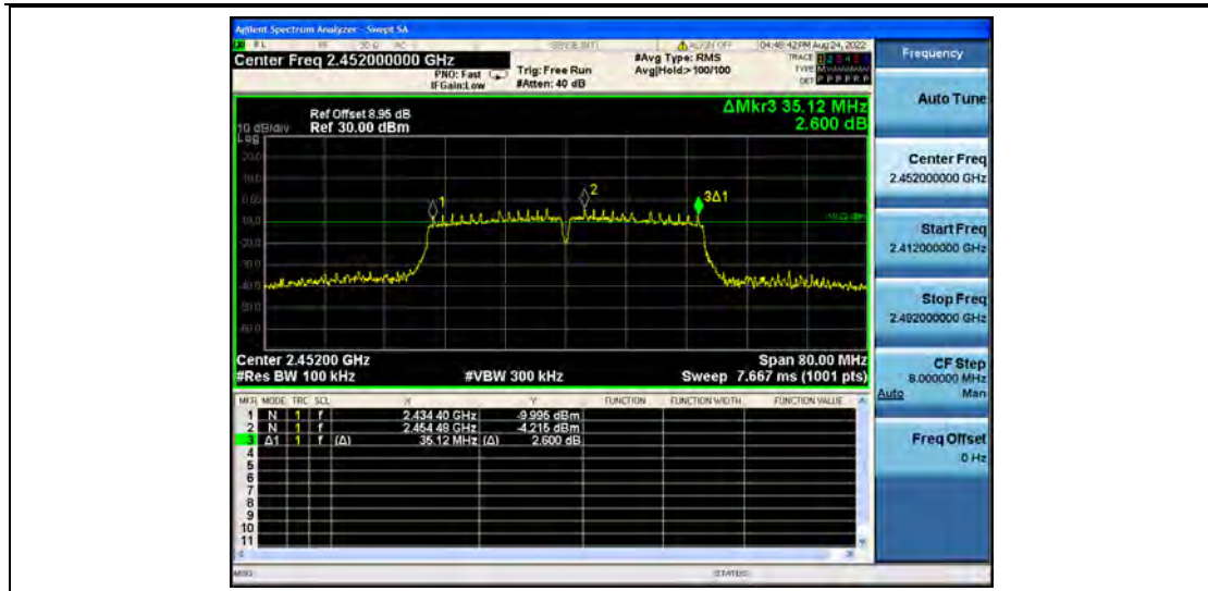
11N40MIMO_Ant2_2452
