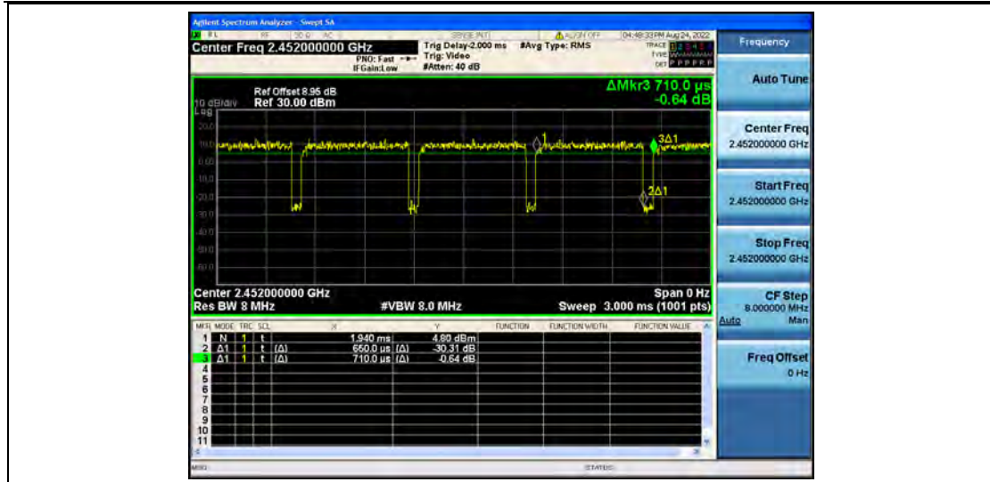
11N40MIMO_Ant2_2452
