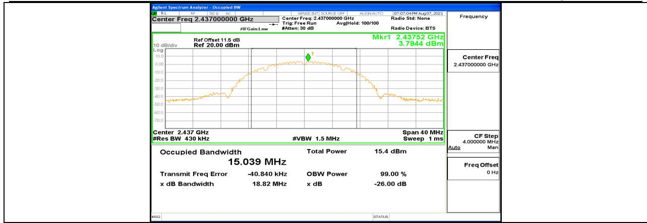
11B Ant2 2437
