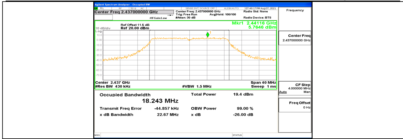
11N20MIMO Ant2 2437
